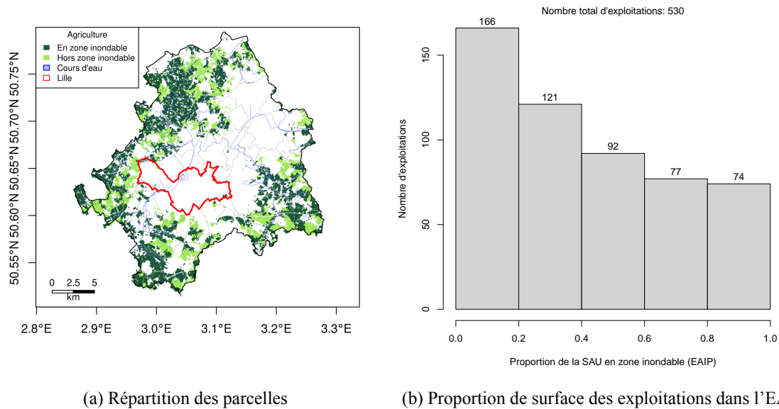
Fig. 3.3 : Exposition de la surface agricole utile (SAU) aux inondations sur le territoire de Lille (source : personnelle, données : EAIP, RPG)
