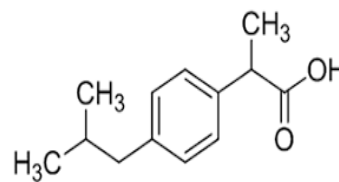
Ibuprofen
