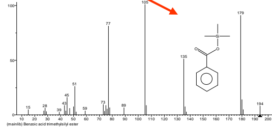
BENZOÏC ACID
