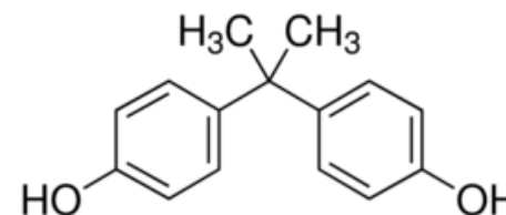
Bisphenol A
