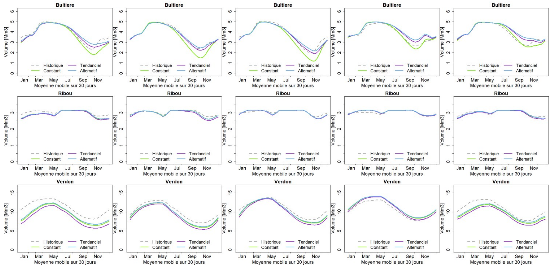
Figure 166 : Régime du volume des 3 gros barrages sur 2050 superposé pour les 3 scénarios et la période historique. En ligne, les 3 barrages, en colonne, les 5 modèles climatiques (selon l'ordre suivant : C2, B3, F4, A1, C1)
