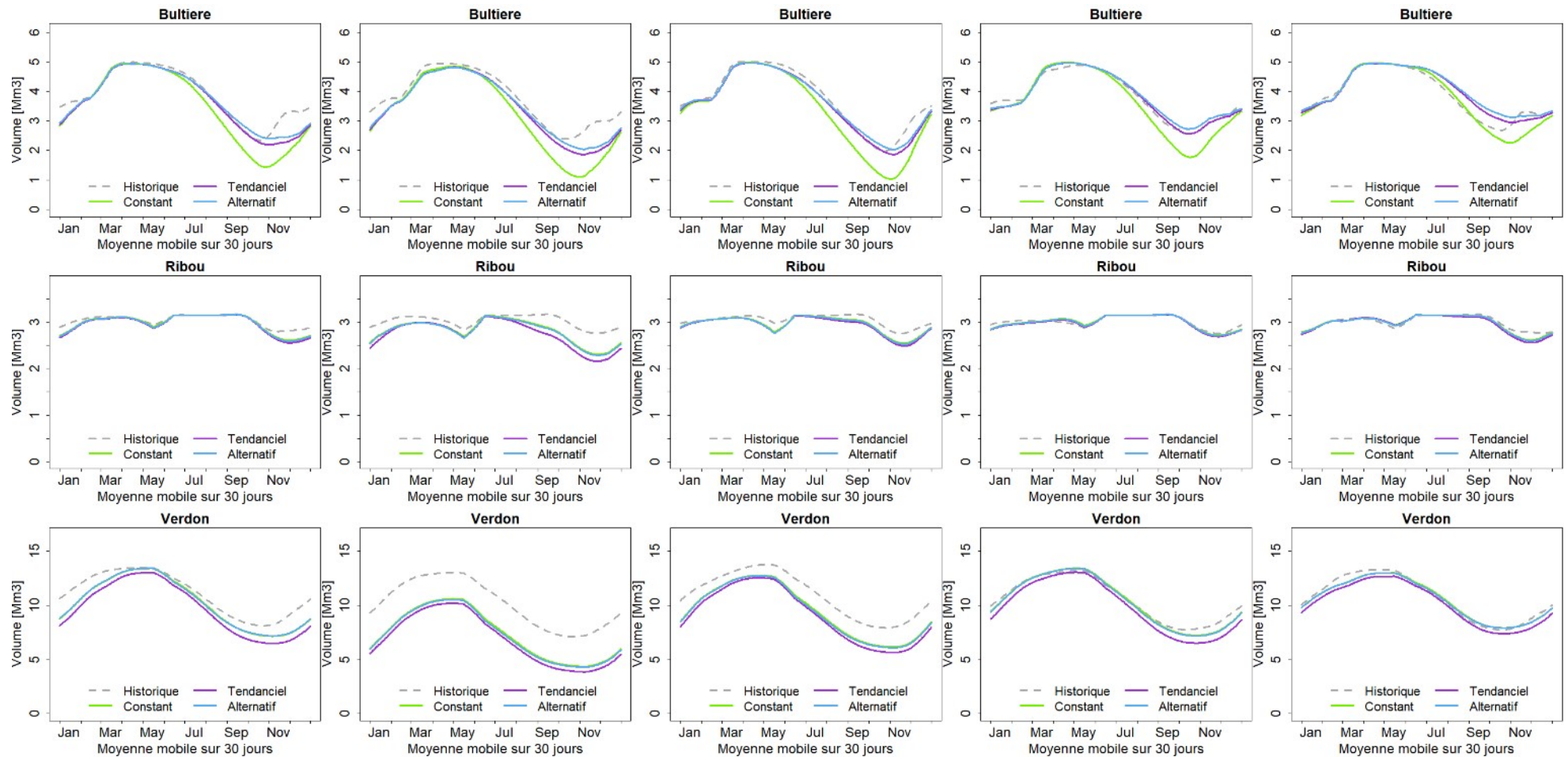
Figure 183 : Régime du volume des 3 gros barrages sur 2070 superposé pour les 3 scénarios et la période historique. En ligne, les 3 barrages, en colonne, les 5 modèles climatiques
