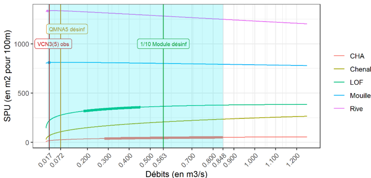
Figure 22: Evolution des surfaces pondérées utiles en fonction du débit sur la Maine à Aigrefeuille (MAIN). (La portion de courbe épaissie correspond à la plage de débit biologique pour la guilde considérée).
