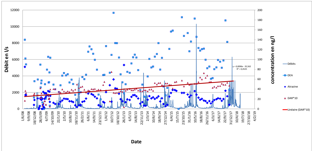
Figure 3. Evolution temporelle de la concentration moyenne mensuelle de l'atrazine (en bleu foncé) et de son produit de dégradation la DEA (en bleu clair) et des débits associés. Le rapport entre la DEA et l'atrazine (le DAR * 10, en rouge) et la régression linéaire.
