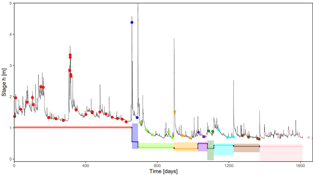
Figure 21. Evolution du paramètre « b1 » du contrôle à bas débit
