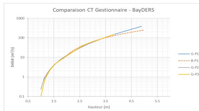
Figure 19. Loire à Goudet : comparaison des courbes de tarage gestionnaire et BayDERS sur la première période détectée par BayDERS
