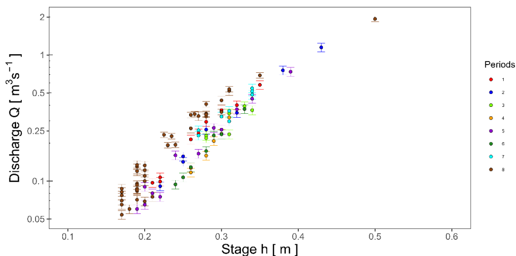
Figure 5. Jaugeages (en échelle log) après segmentation BIC – CI, a priori de l'écart du \mu = 0.5 \text{ m}^3/\text{s} et incertitude relative variable de 5 % et 8 %
