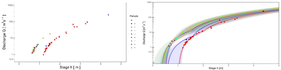
Figure 20. La Loire à Goudet : jaugeages groupé par périodes en suivant la méthode BaRatin (à gauche) et courbe de tarage multi-période issue du BaRatin-SPD (à droite)
