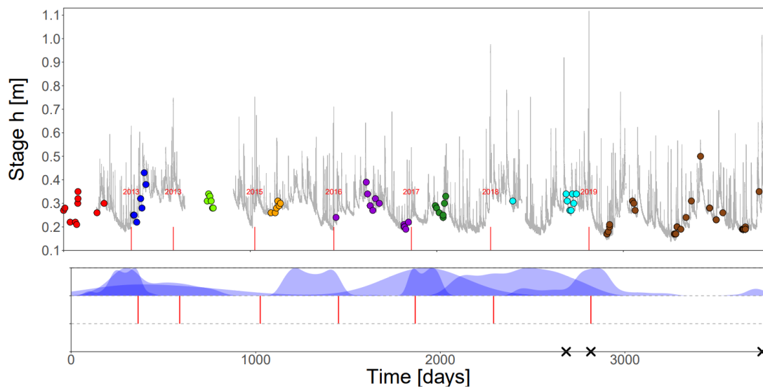
Figure 3. Limnigramme après segmentation BIC - CI, a priori sur l'écart moyen \mu = 0.5 \text{ m}^3/\text{s} et incertitude relative variable de 5 % et 8 %
