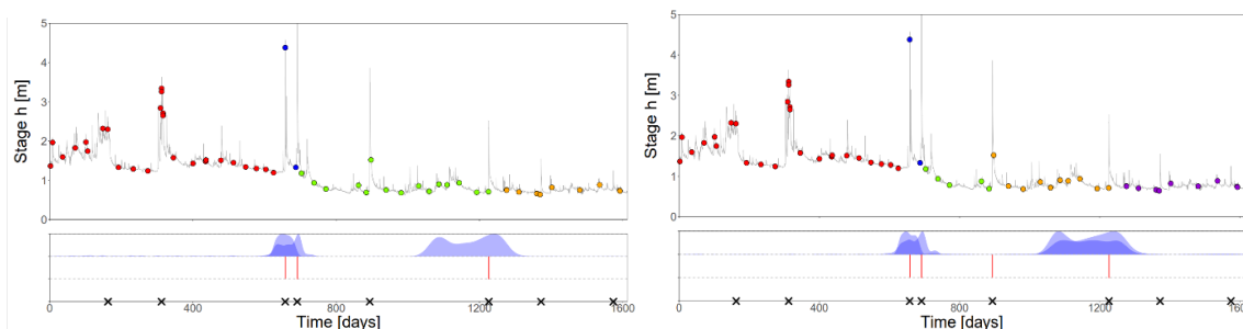
Figure 16. Loire à Goudet, segmentation par jauges : incertitude associée constante à 15 % (à gauche) et constante à 20 % (à droite)
