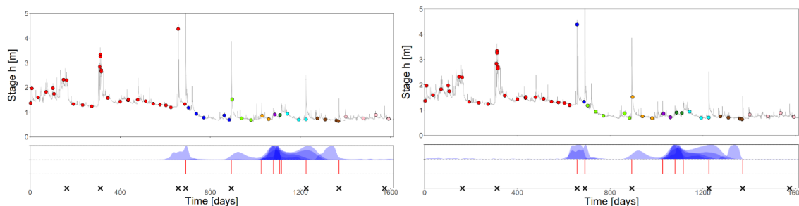
Figure 15. Loire à Goudet, segmentation par jauges : incertitude associée d'après Barème (à gauche) et constante à 10 % (à droite)
