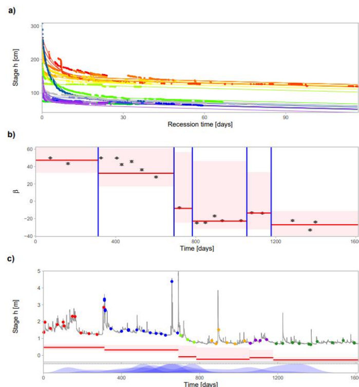
Figure 25. Loire à Goudet, période 01/2018 – 06/2022 : segmentation et évolution du fond du lit à partir de la méthode de segmentation par récession
