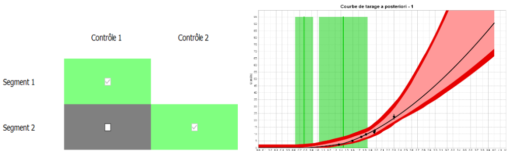
Figure 13. Matrice des contrôles et courbe de tarage a posteriori de la station de la Loire à Goudet
