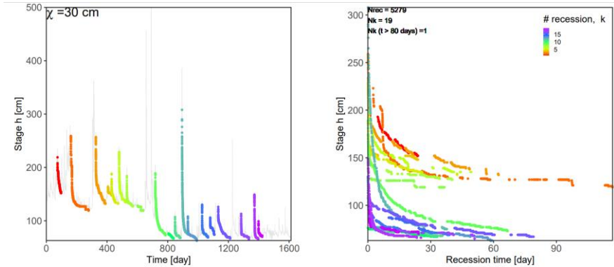
Figure 23. Loire à Goudet, période 01/2018 – 06/2022 : résultats de l'extraction des récessions
