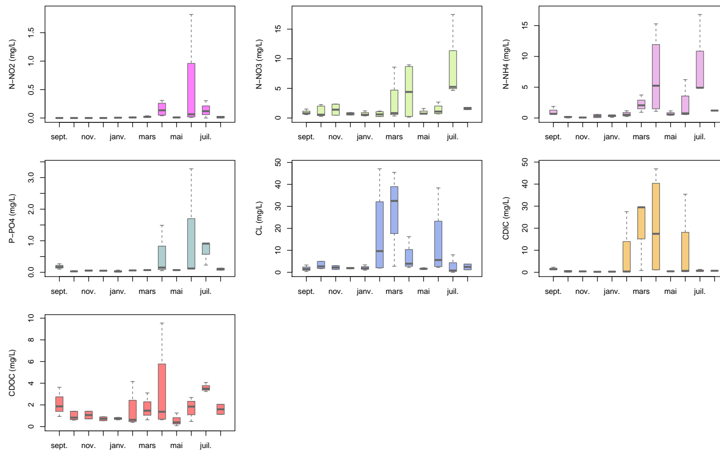
FIGURE 50 – Distributions des concentrations mensuelles en azote du nitrite (N-NO2), azote du nitrate (N-NO3), azote de l’ammonium (N-NH4), phosphore du phosphate (P-PO4), chlorure (CL), carbone inorganique dissous (DIC), carbone organique dissous (DOC) à la station BOISSY-P28 au cours de l’année hydrologique (les outliers ne sont pas représentés).
