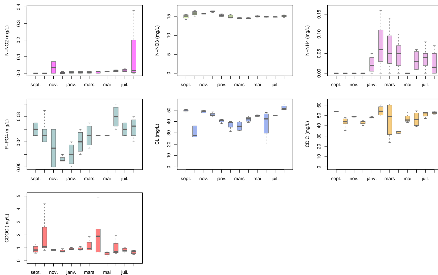
FIGURE 51 – Distributions des concentrations mensuelles en azote du nitrite (N-NO 2 ), azote du nitrate (N-NO 3 ), azote de l'ammonium (N-NH 4 ), phosphate (P-PO 4 ), chlorure (CL), carbone inorganique dissous (DIC), carbone organique dissous (DOC) à la station CHANTEMERLE-PG au cours de l'année hydrologique (les outliers ne sont pas représentés).
