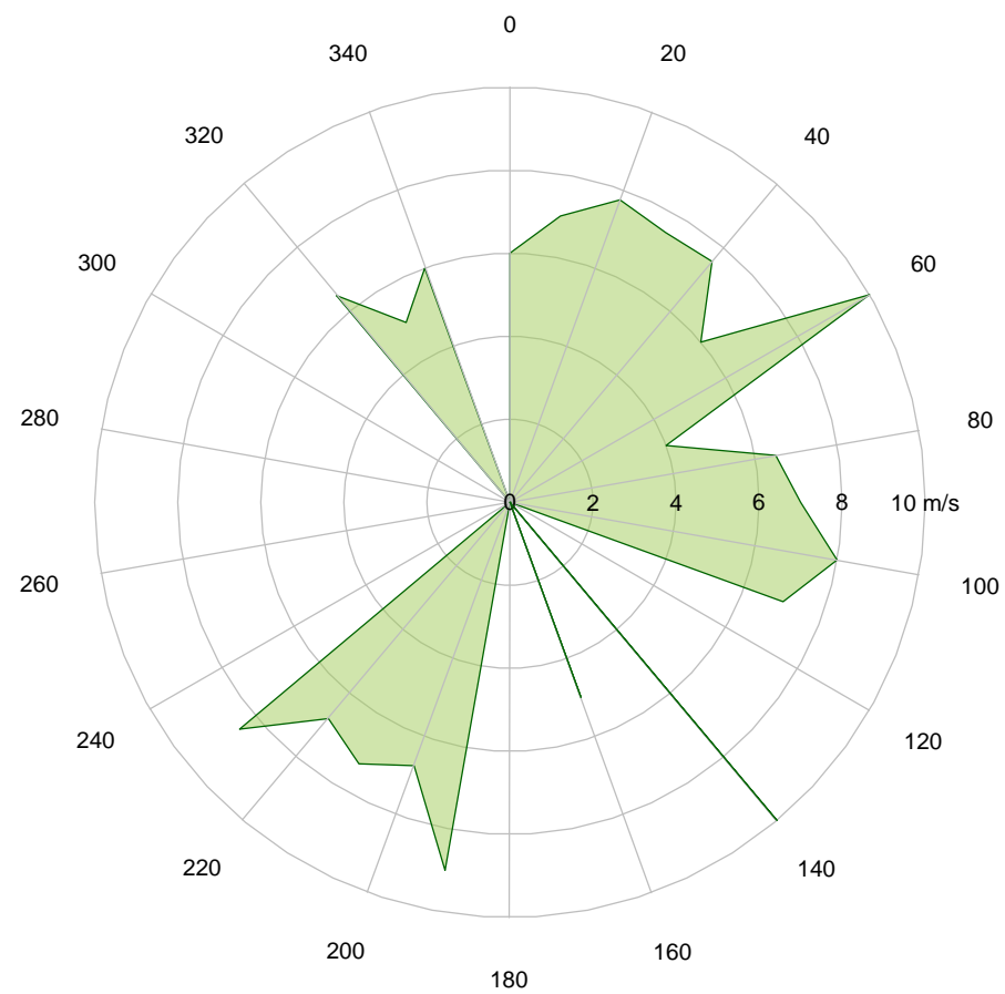
FIGURE 22 – Direction du vent à la station météorologique BOISSY-METEO entre le 01 juin 2013 et le le 30 août 2013.
