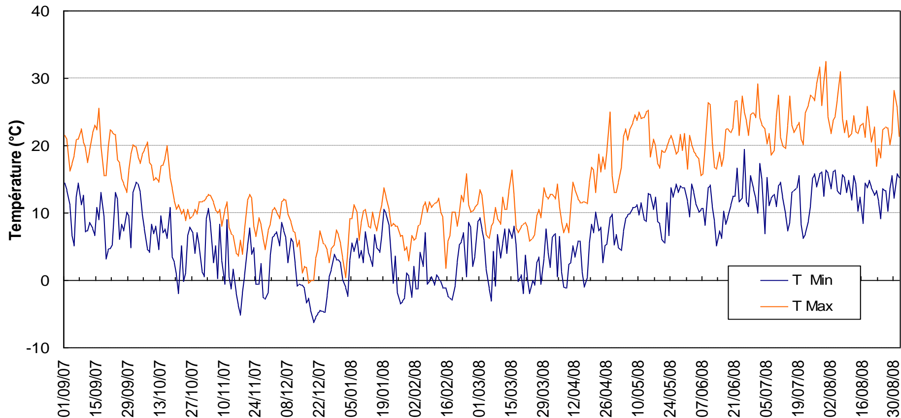
Station météo de Boissy Le Chatel : Valeurs journalières des températures maximales et minimales
