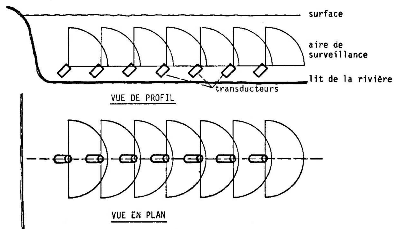
Figure 33 - Disposition des transducteurs dans le compteur " BENDIX "
