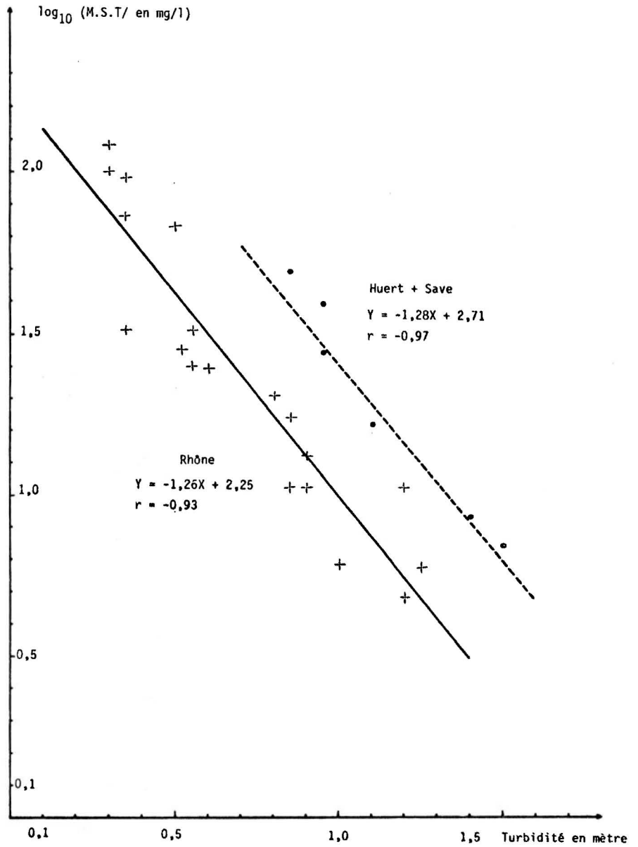
Figure 4 - Représentation de la corrélation Turbidité-Matières totales en suspension.
