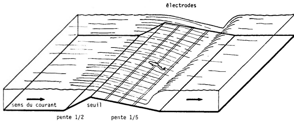
Figure 32 - Emplacement des électrodes sur un barrage de jaugeage " CRUMP "
