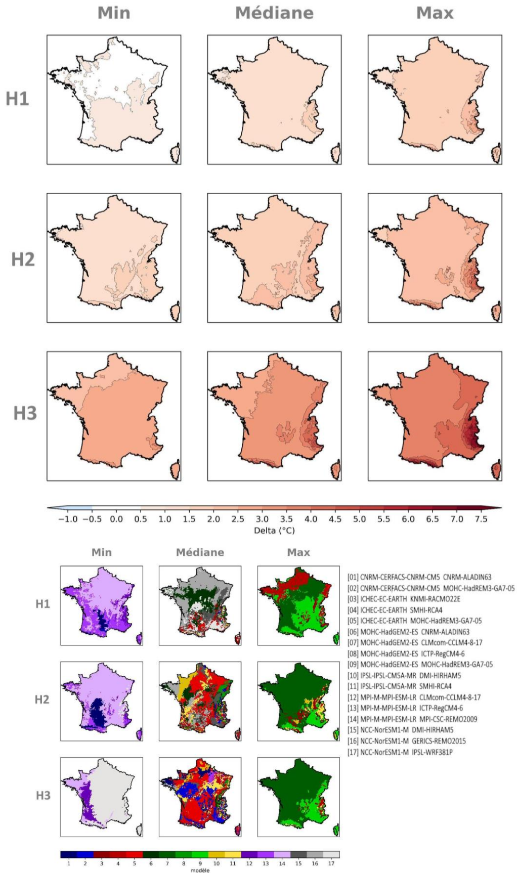
Figure 53 : Cartes des écarts de de température moyenne en hiver par horizon selon le scénario RCP8.5 (multi-horizon, mosaïque, Explore2-2024, CDF-t).
