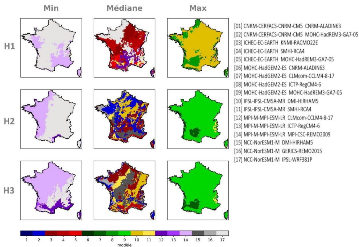
Figure 11 : Exemple de matrice mosaïque : identification du couple GCM/RCM de l'ensemble Explore2-2024 associé aux minimums, médianes et maximums des écarts de température moyenne annuelle sous RCP8.5 de la matrice multi-horizon.
