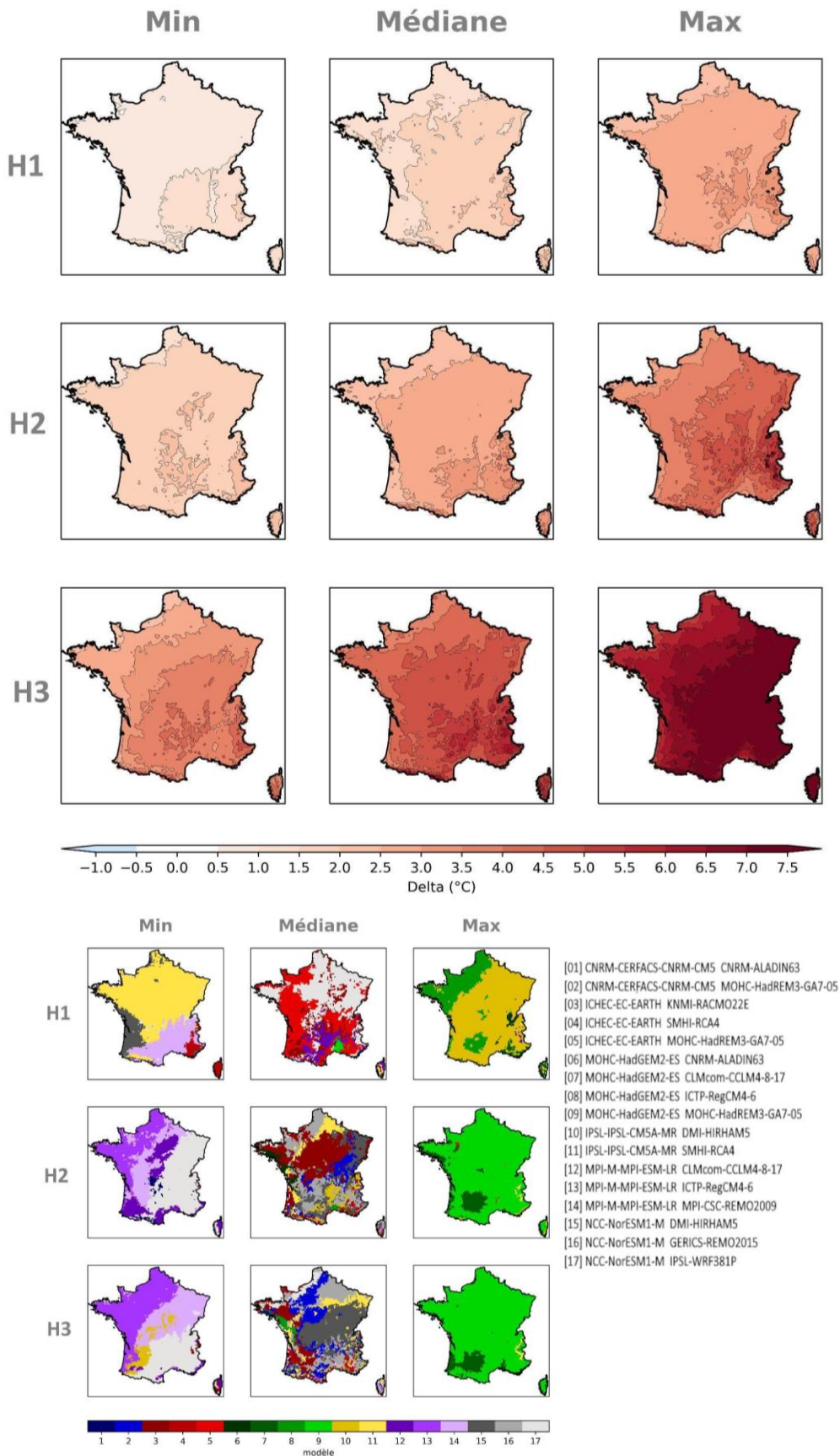
Figure 20 : Cartes des écarts de température moyenne en été à la période de référence par horizon selon le scénario RCP8.5 (multi-horizon, mosaïque, Explore2-2024, ADAMONT).
