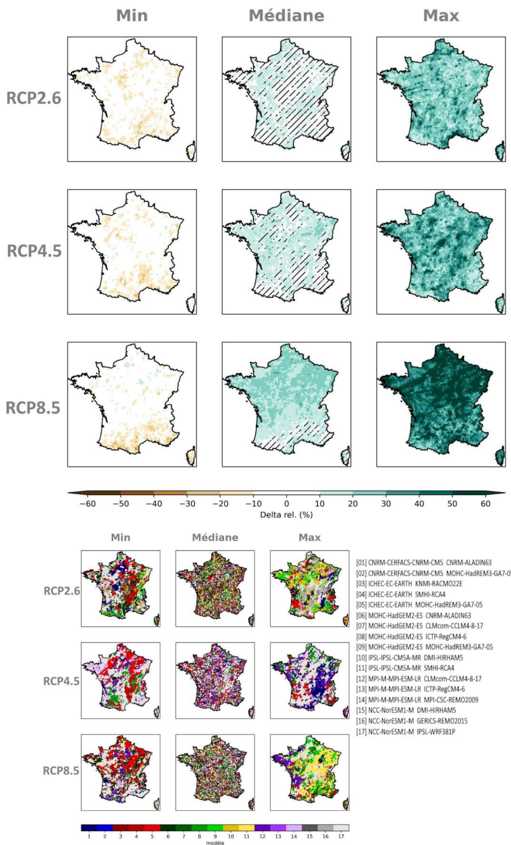
Figure 35 : Cartes des écarts relatifs de précipitations maximales annuelles journalières à la période de référence par scénario RCP à l'horizon lointain (H3, 2070-2099) (multi-scénario, mosaïque, Explore2-2024, ADAMONT).
