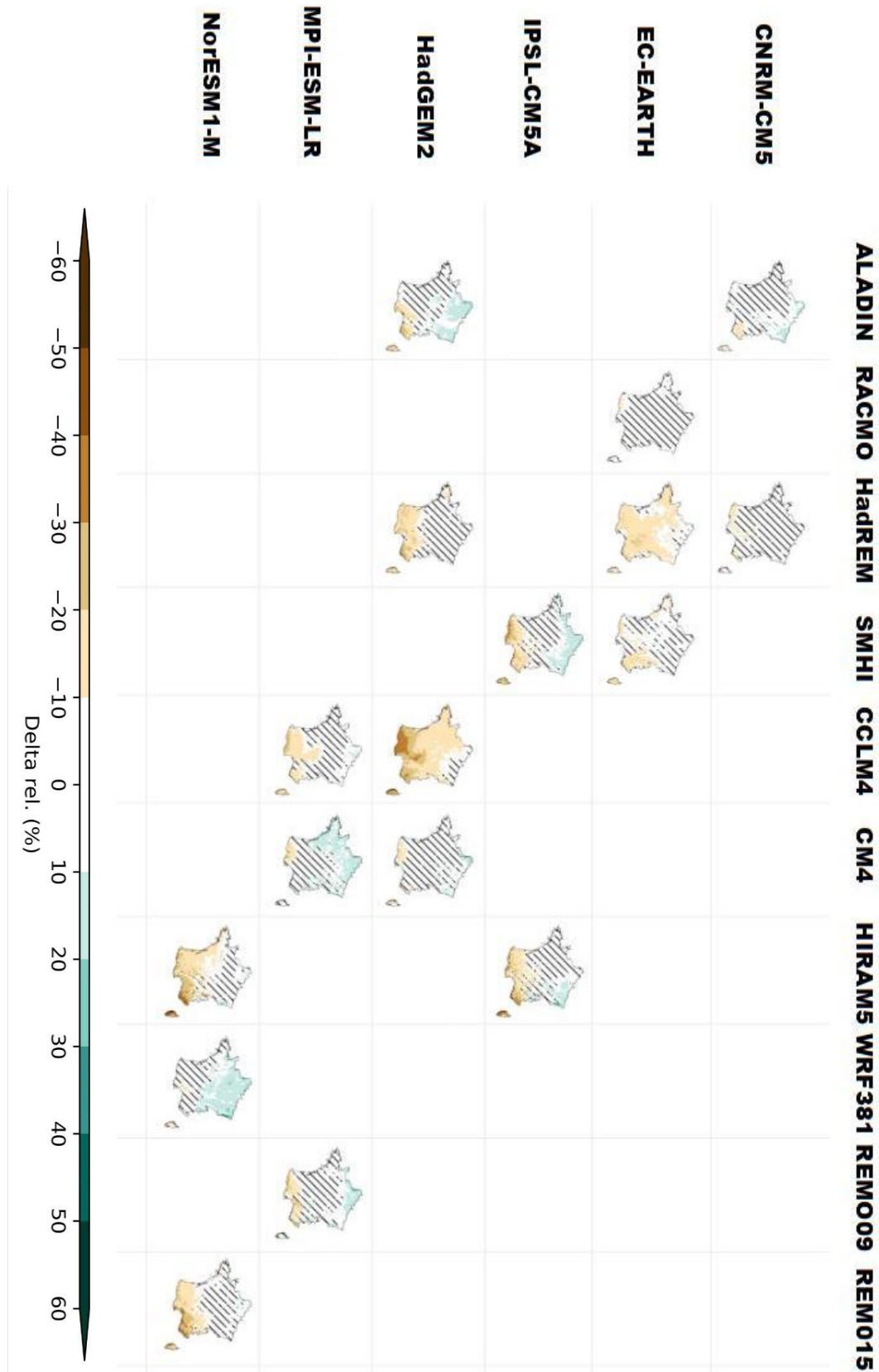
Figure 58 : Cartes des écarts de cumul annuel de précipitations à l'horizon lointain (H3, 2070-2099) pour le scénario RCP8.5 par rapport à la période de référence 1976-2005 pour chacun des 17 couples GCM/RCM de l'ensemble Explore2-2024. Les lignes correspondent aux GCMs, les colonnes aux RCMs (ensemble, Explore2-2024, CDF-t).
