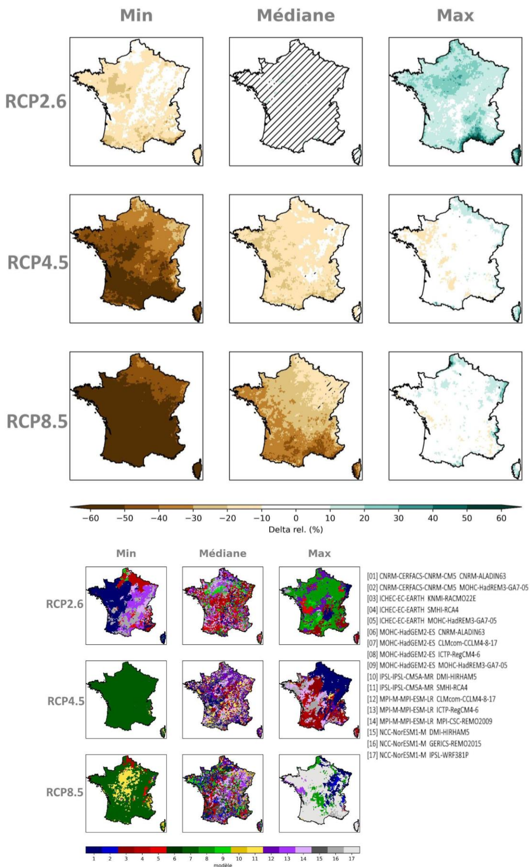
Figure 66 : Cartes des écarts de cumul hivernal de précipitations à la période de référence par scénario RCP à l'horizon lointain (H3, 2070-2099) (multi-scénario, mosaïque, Explore2-2024, CDF-t).
