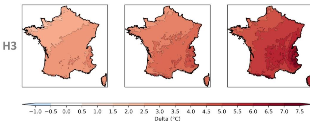
Figure 8 : Exemple de produit de distribution : cartes des écarts de température moyenne annuelle selon le scénario RCP8.5 entre l'horizon lointain (H3, 2070-2099) et la référence (1976-2005), minimum (gauche), médian (centre) et maximum (droite) de l'ensemble Explore2-2024 (méthode ADAMONT).
