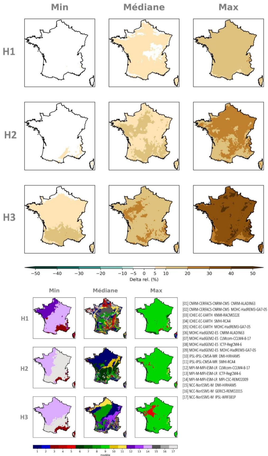
Figure 72 : Cartes des écarts de cumul annuel de l'évapotranspiration de référence par horizon selon le scénario RCP8.5 (multi-horizon, mosaïque, Explore2-2024, CDF-t).
