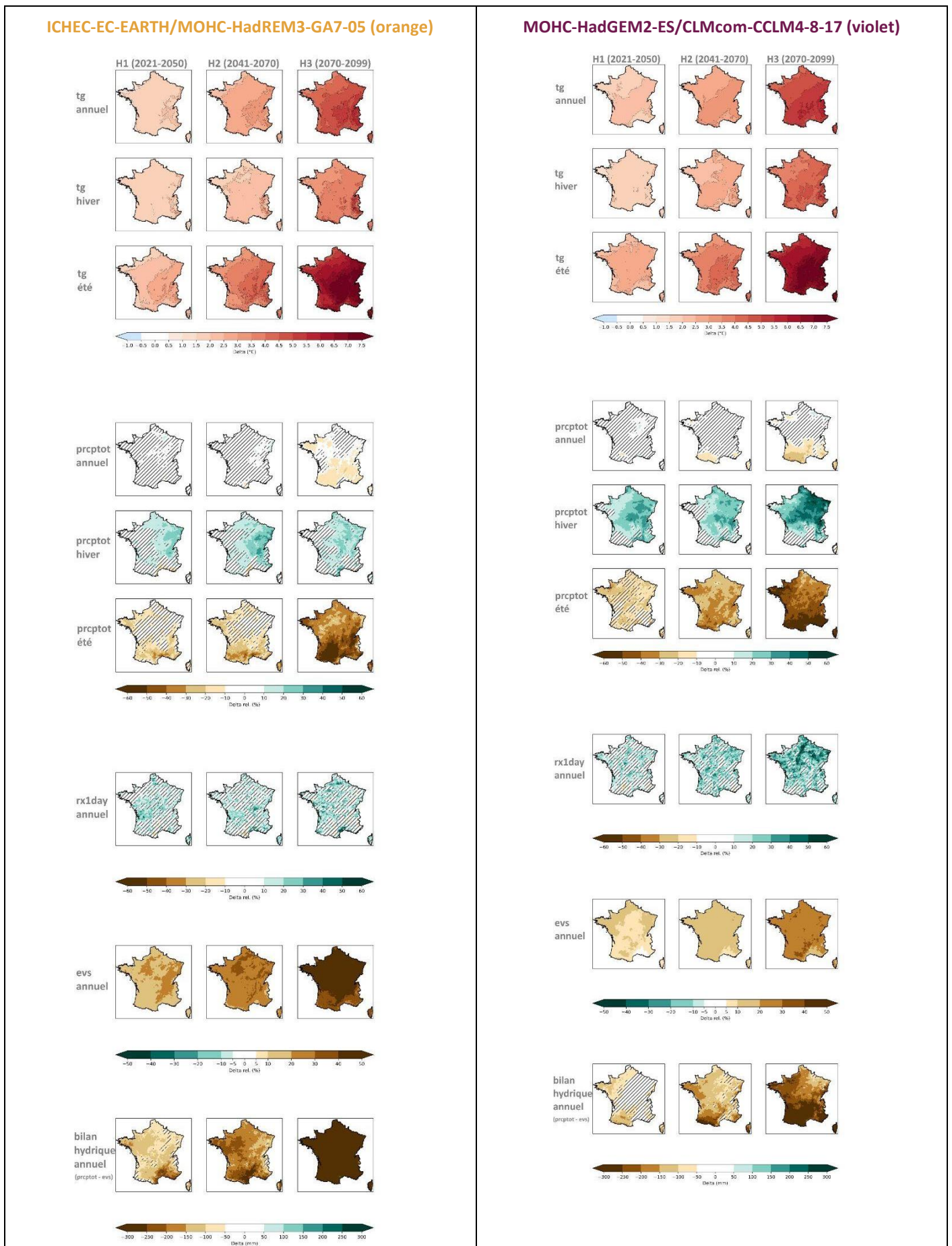
Figure 44 : Changements projetés par les quatre narratifs aux différents horizons. (suite).
