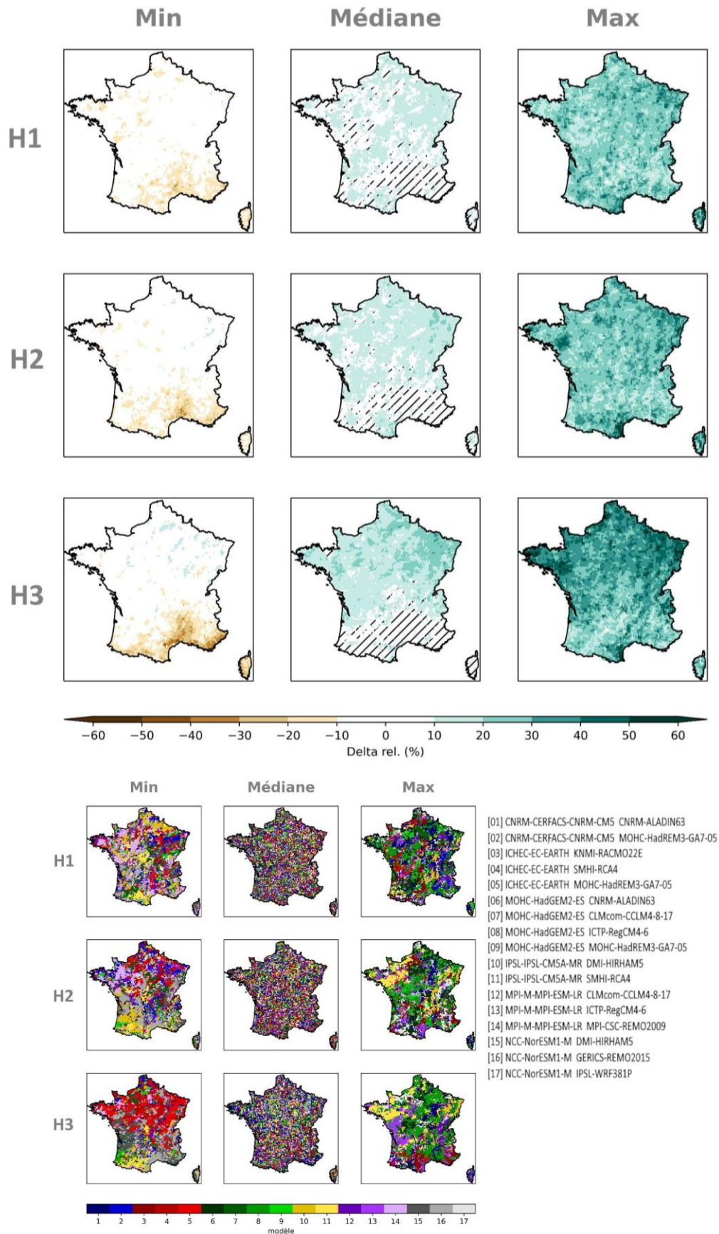
Figure 68 : Cartes des écarts relatifs de précipitations maximales annuelles journalières par horizon selon le scénario RCP8.5 (multi-horizon, mosaïque, Explore2-2024, CDF-t).
