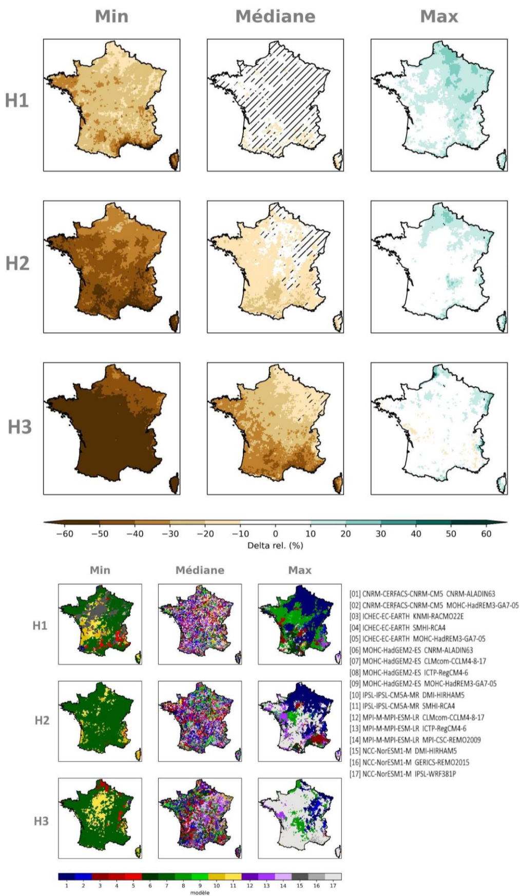
Figure 65 : Cartes des écarts de de cumul hivernal de précipitations par horizon selon le scénario RCP8.5 (multi-horizon, mosaïque, Explore2-2024, CDF-t).
