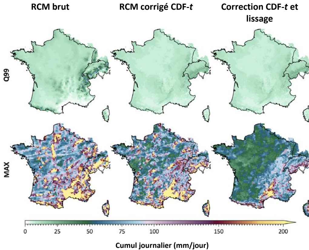
Figure 2 : Quantile 99 % (Q99) et maximum (MAX) des précipitations sur la période 2081-2100 (échantillonnés de septembre à décembre) pour le couple NCC-NorESM1-M/DMI-HIRHAM5 sous RCP 8.5. De gauche à droite : modèle brut, correction avec CDF-t sans ajustement des extrêmes de précipitations, et correction avec CDF-t après ajustement des extrêmes de précipitations.
