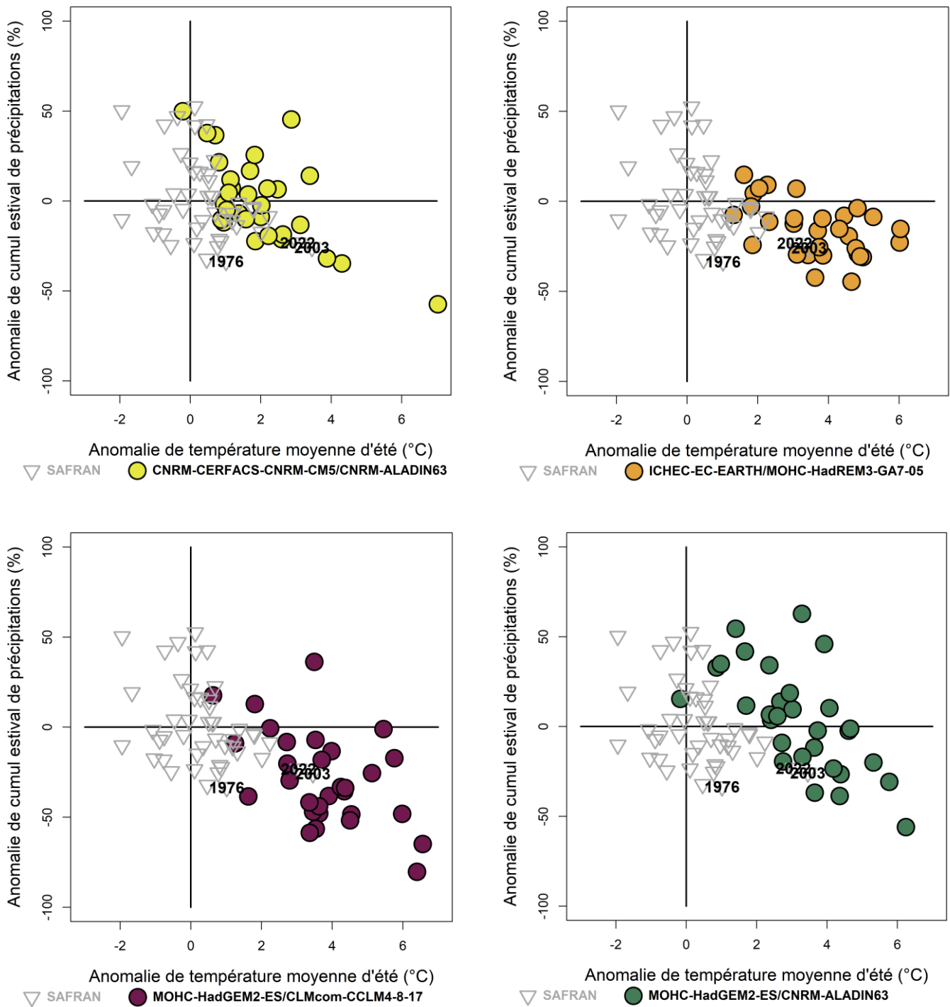
Figure 48 : Anomalies saisonnières (été : juin-juillet-août) de température (en abscisse) et précipitations (en ordonnée) pour la réanalyse SAFRAN (en jaune) et les quatre narratifs (en jaune). Les anomalies SAFRAN sont calculées par rapport à la période 1976-2005. L'année 2022 correspond au point d'anomalie +3°C en température et -23 % en précipitations. Pour les narratifs, les anomalies sont calculées par rapport à chacune des simulations historiques des quatre couples GCM/RCM respectivement.
