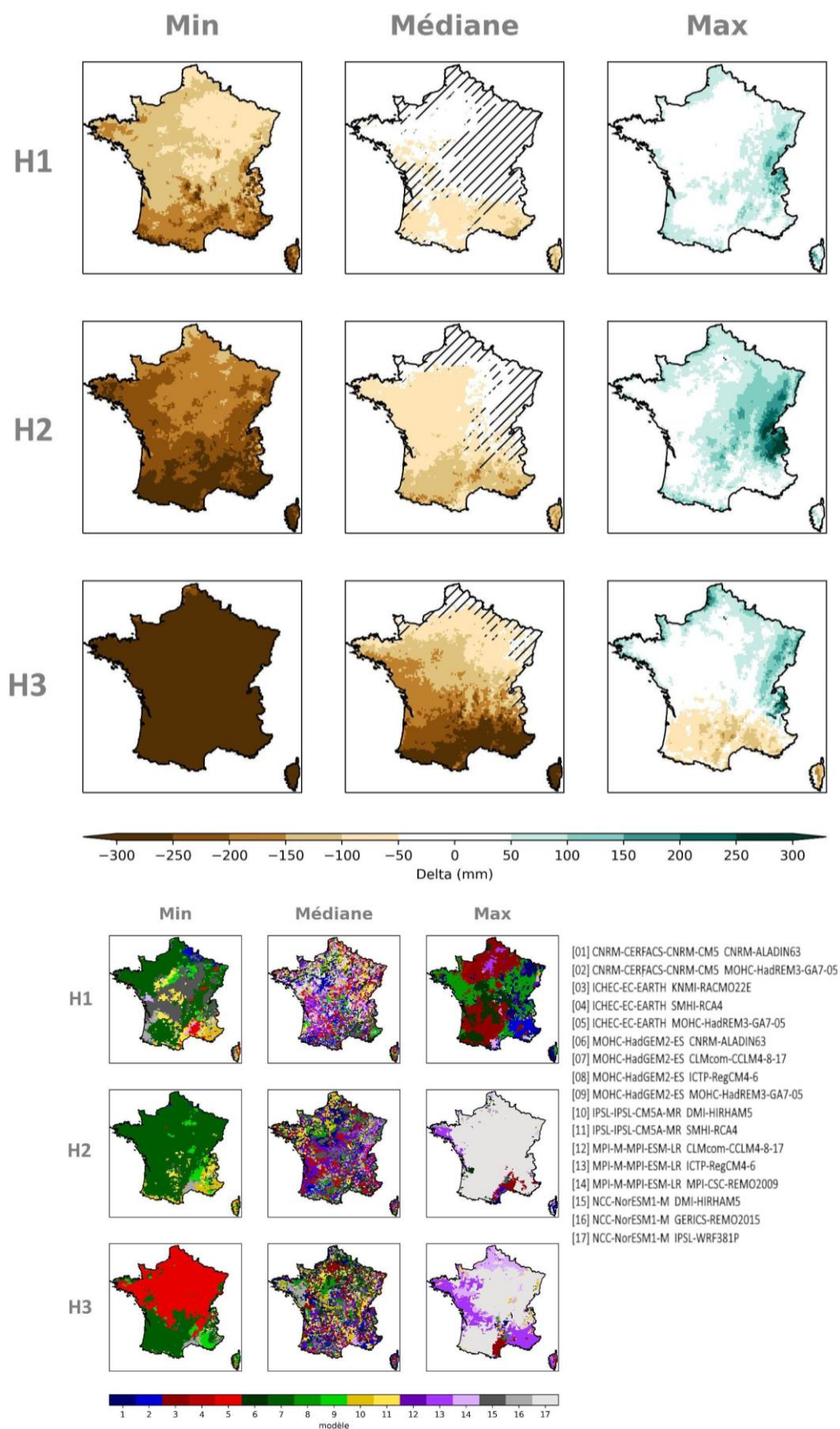
Figure 75 : Cartes des écarts du bilan hydrique par horizon selon le scénario RCP8.5 (multi-horizon, mosaïque, Explore2-2024, CDF-t).
