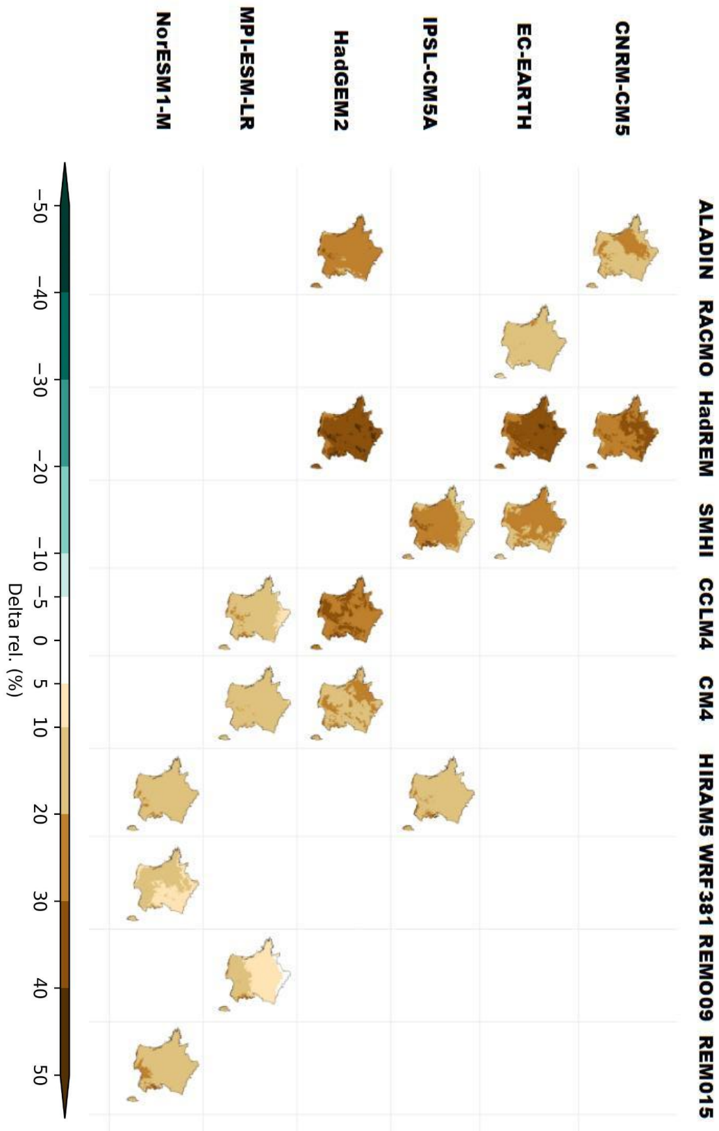
Figure 71 : Cartes des écarts de cumul annuel de l'évapotranspiration de référence à l'horizon lointain (H3, 2070-2099) pour le scénario RCP8.5 par rapport à la période de référence 1976-2005 pour chacun des 17 couples GCM/RCM de l'ensemble Explore2-2024. Les lignes correspondent aux GCMs, les colonnes aux RCMs (ensemble, Explore2-2024, CDF-t).
