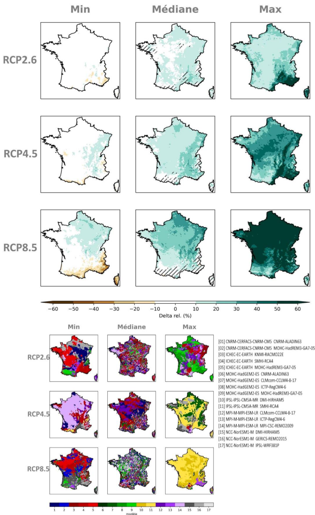
Figure 28 : Cartes des écarts relatifs de cumul hivernal de précipitations à la période de référence par scénario RCP à l'horizon lointain (H3, 2070-2099) (multi-scénario, mosaïque, Explore2-2024, ADAMONT).
