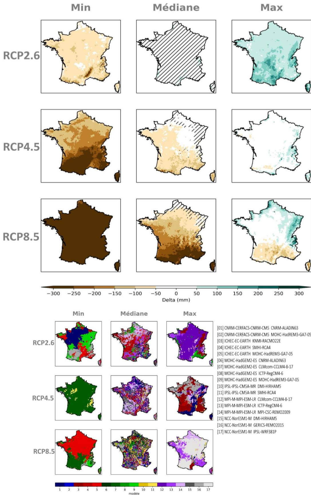
Figure 76 : Cartes des écarts du bilan hydrique à la période de référence par scénario RCP à l'horizon lointain (H3, 2070-2099) (multi-scénario, mosaïque, Explore2-2024, CDF-t).
