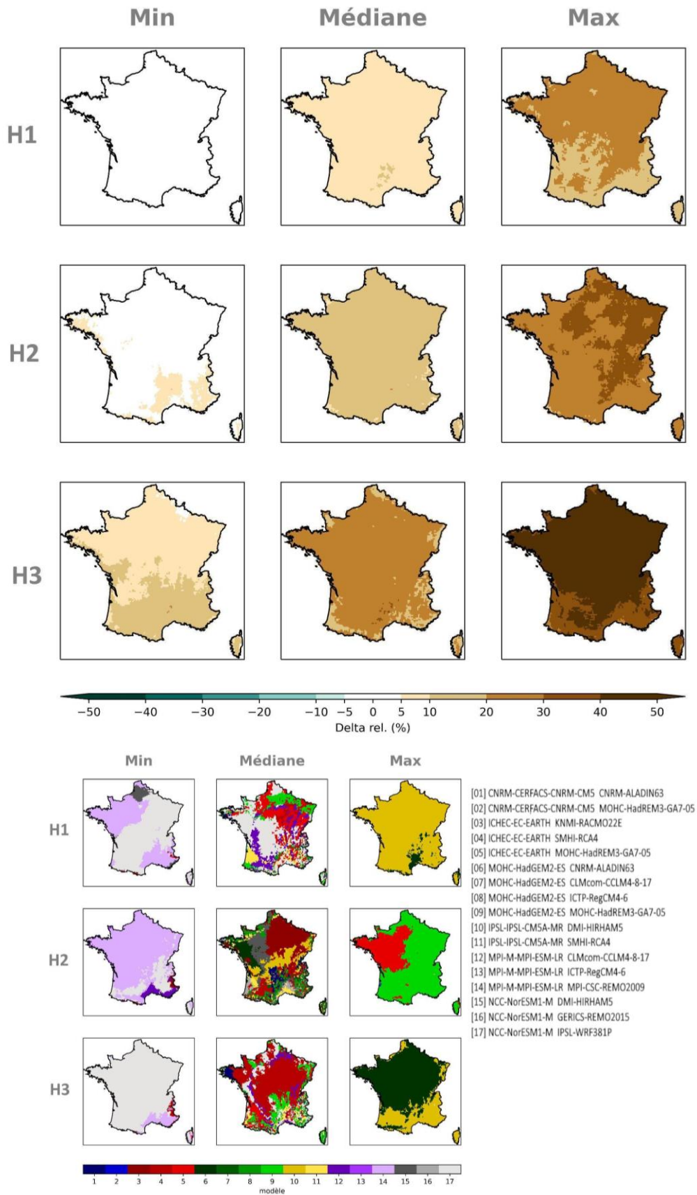
Figure 38 : Cartes des écarts d'évapotranspiration de référence annuelle à la période de référence par horizon selon le scénario RCP8.5 (multi-horizon, mosaïque, Explore2-2024, ADAMONT).
