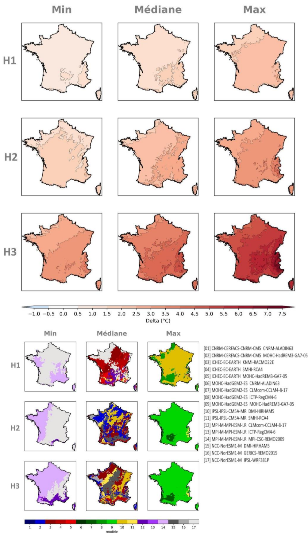
Figure 14 : Cartes des écarts de température moyenne annuelle à la période de référence par horizon selon le scénario RCP8.5 (multi-horizon, mosaïque, Explore2-2024, ADAMONT).
