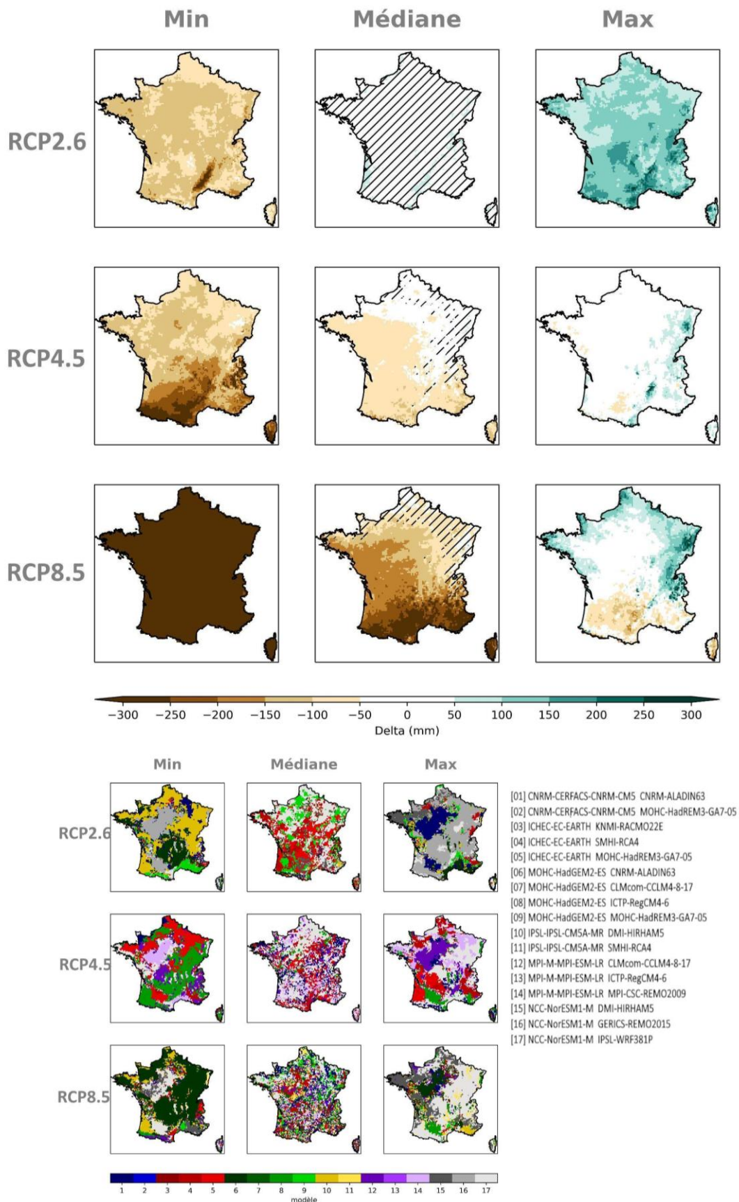
Figure 43 : Cartes des écarts de bilan hydrique annuel (p-eps) à la période de référence par scénario RCP à l'horizon lointain (H3, 2070-2099) (multi-scénario, mosaïque, Explore2-2024, ADAMONT).
