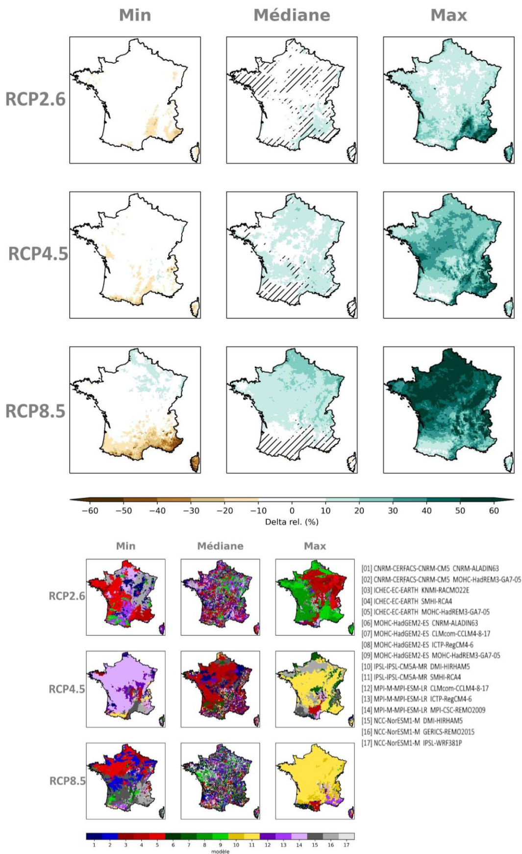
Figure 63 : Cartes des écarts de cumul hivernal de précipitations à la période de référence par scénario RCP à l'horizon lointain (H3, 2070-2099) (multi-scénario, mosaïque, Explore2-2024, CDF-t).
