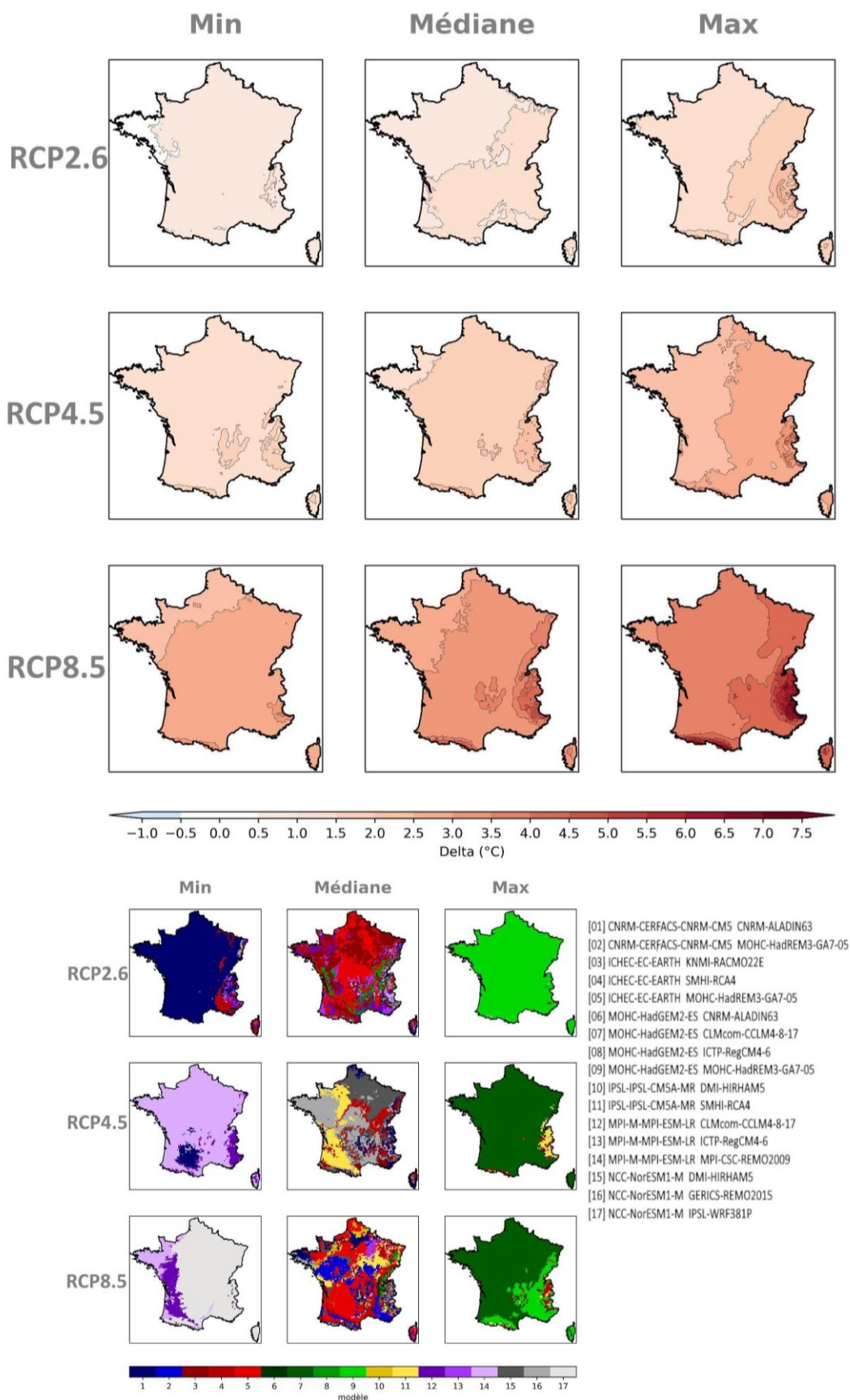
Figure 54 : Cartes des écarts de température moyenne en hiver annuelle à la période de référence par scénario RCP à l'horizon lointain (H3, 2070-2099) (multi-scénario, mosaïque, Explore2-2024, CDF-t).
