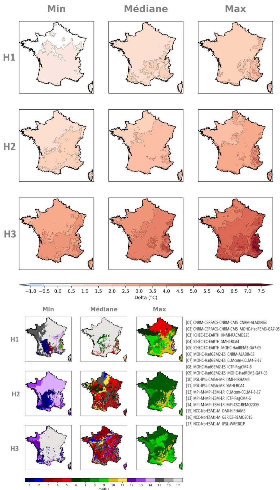
Figure 17 : Cartes des écarts de température moyenne en hiver à la période de référence par horizon selon le scénario RCP8.5 (multi-horizon, mosaïque, Explore2-2024, ADAMONT).
