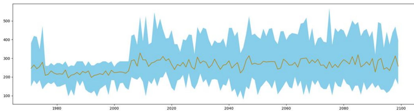
Figure 70 : Evolution du maximum absolu de précipitation journalière en France de l'ensemble Explore2-2024 sous RCP8.5 sur la période de simulation.
