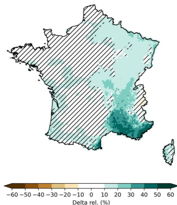
Figure 6 : Représentation des incertitudes liées à la variabilité interne dans les simulations individuelles. Les hachures indiquent les mailles où le changement n'est pas significatif au regard de la variabilité interne du climat.
