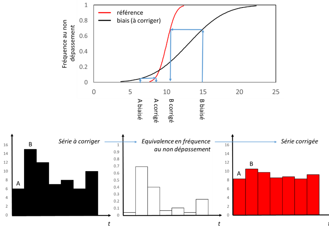
Figure 1 : Principe de la méthode « quantile mapping » (source :INRAE)
