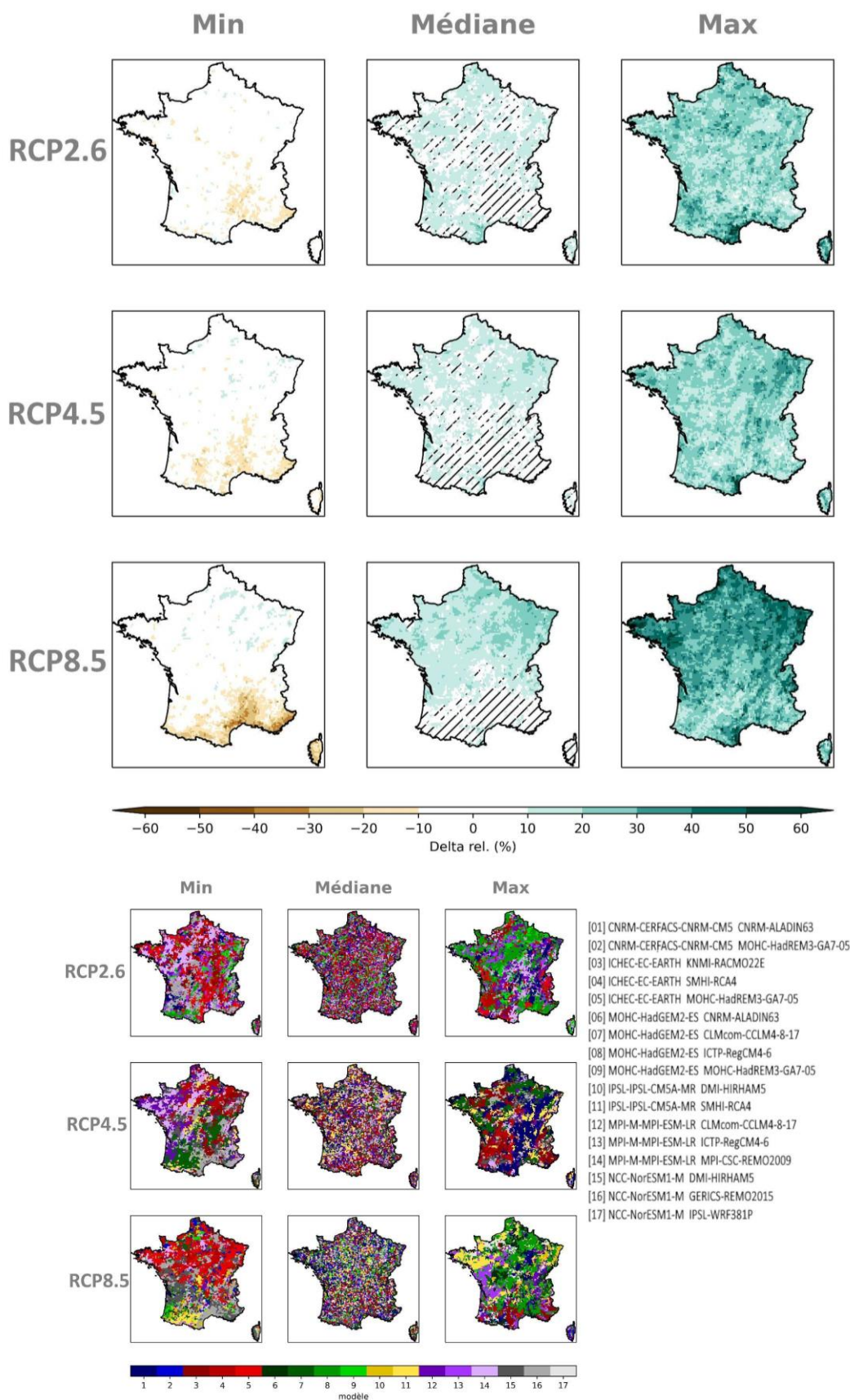
Figure 69 : Cartes des écarts des précipitations maximales annuelles journalières à la période de référence par scénario RCP à l'horizon lointain (H3, 2070-2099) (multi-scénario, mosaïque, Explore2-2024, CDF-t).
