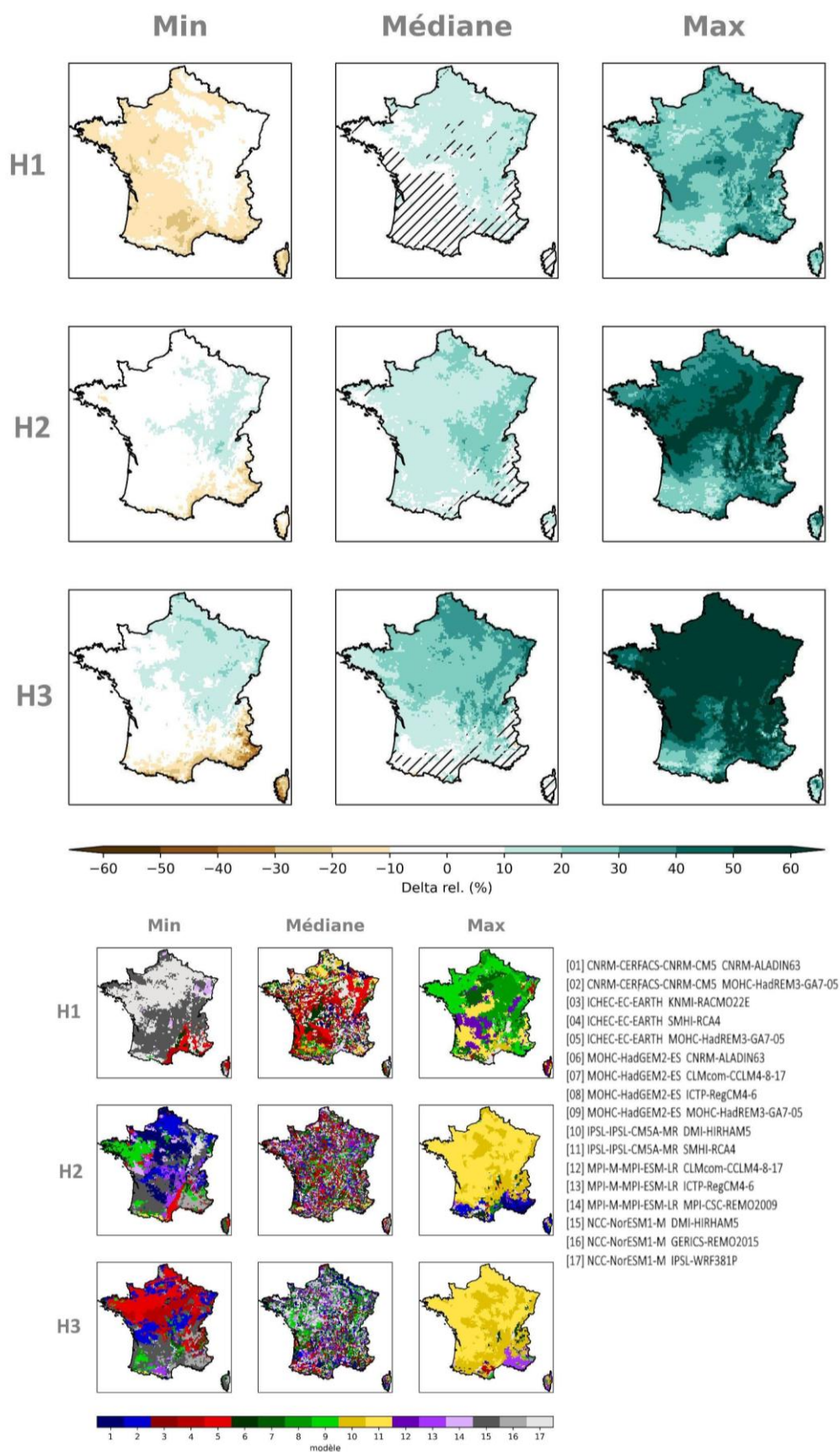
Figure 27 : Cartes des écarts relatifs de cumul hivernal de précipitations à la période de référence par horizon selon le scénario RCP8.5 (multi-horizon, mosaïque, Explore2-2024, ADAMONT).
