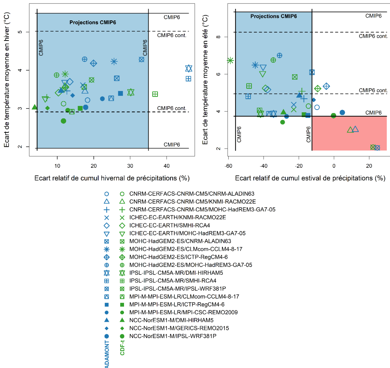
Figure 4 : Changements en température et précipitations sur la France des 19 simulations Explore2 corrigées par les méthodes ADAMONT et CDF-t sur les saisons hiver et été, comparés aux quantiles 5% et 95% (Q5 et Q95) de l'ensemble CMIP6 (« CMIP6 ») et CMIP6 contraint par les observations pour les températures selon la méthode de Ribes et al. (2022) (« CMIP6 cont. »).
