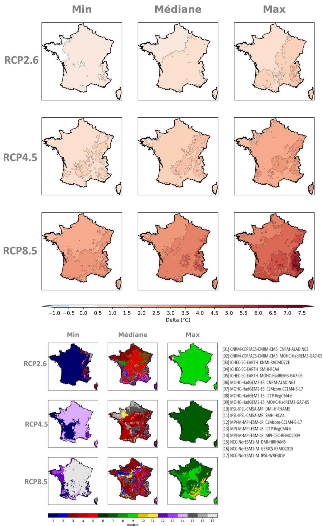
Figure 18 : Cartes des écarts de température moyenne en hiver à la période de référence par scénario RCP à l'horizon lointain (H3, 2070-2099) (multi-scénario, mosaïque, Explore2-2024, ADAMONT).
