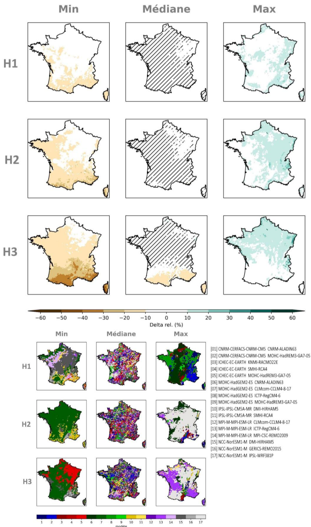
Figure 59 : Cartes des écarts de de cumul annuel de précipitations par horizon selon le scénario RCP8.5 (multi-horizon, mosaïque, Explore2-2024, CDF-t).
