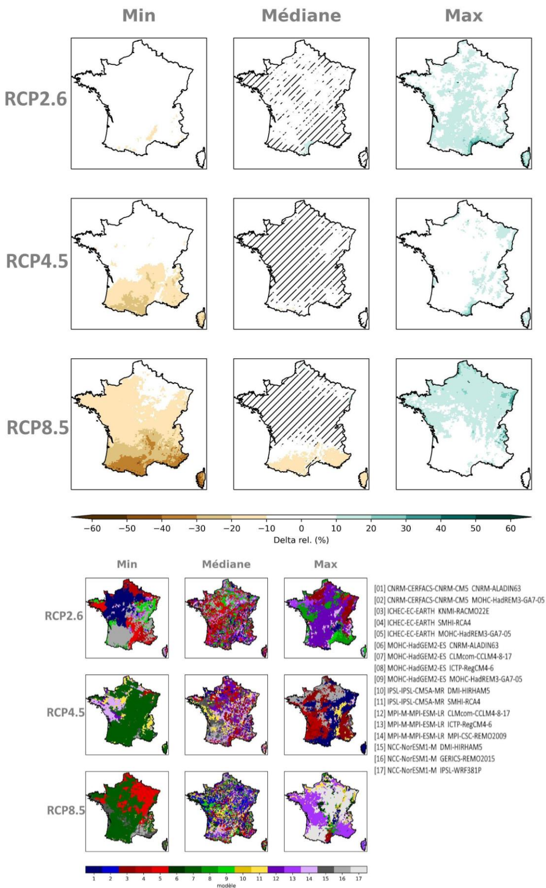
Figure 60 : Cartes des écarts relatifs de cumul annuel de précipitations à la période de référence par scénario RCP à l'horizon lointain (H3, 2070-2099) (multi-scénario, mosaïque, Explore2-2024, CDF-t).
