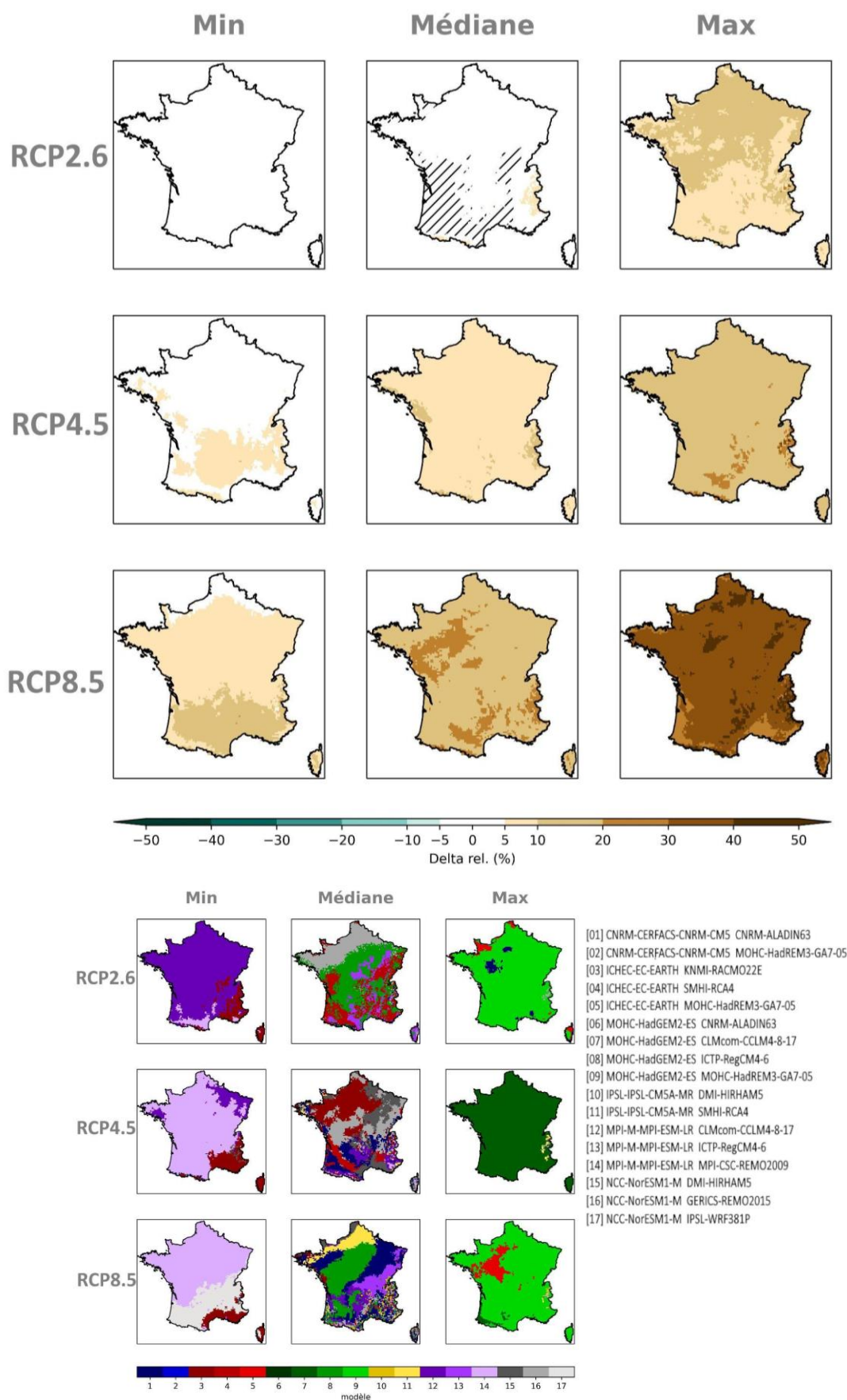
Figure 73 : Cartes des écarts de cumul annuel de l'évapotranspiration de référence à la période de référence par scénario RCP à l'horizon lointain (H3, 2070-2099) (multi-scénario, mosaïque, Explore2-2024, CDF-t).
