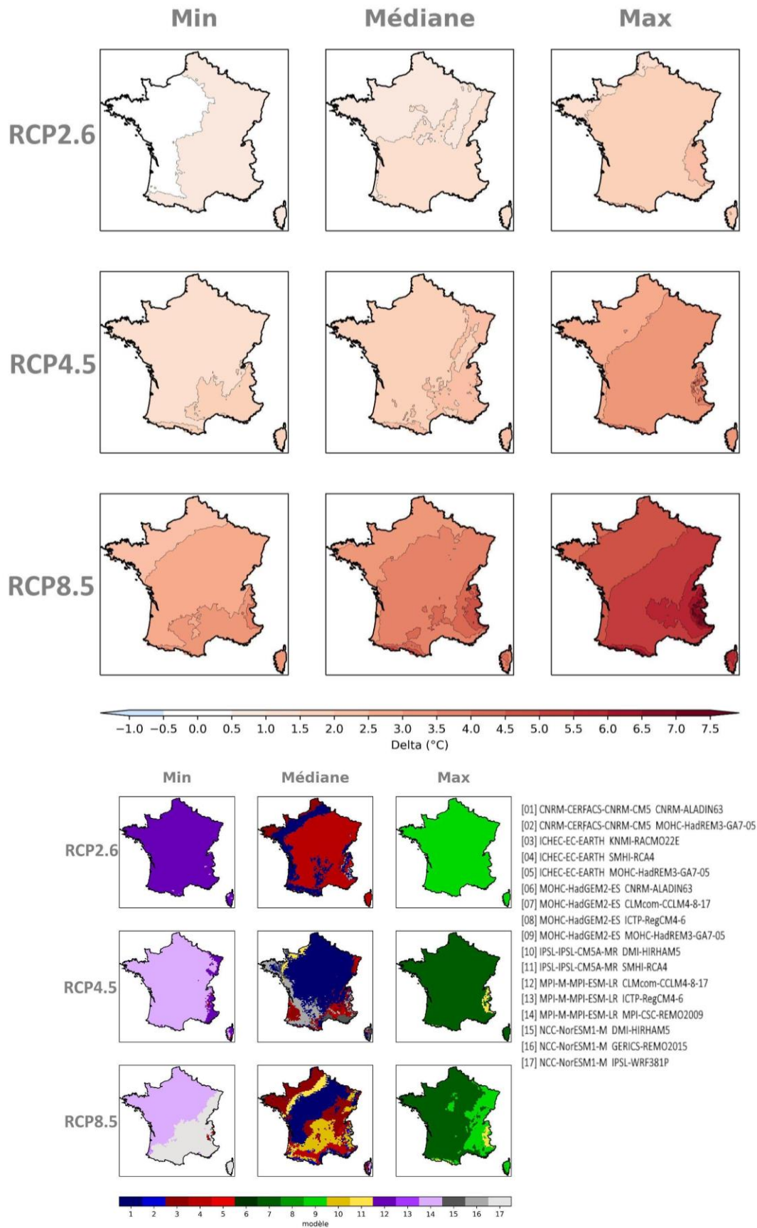
Figure 51 : Cartes des écarts de température moyenne annuelle à la période de référence par scénario RCP à l'horizon lointain (H3, 2070-2099) (multi-scénario, mosaïque, Explore2-2024, CDF-t).
