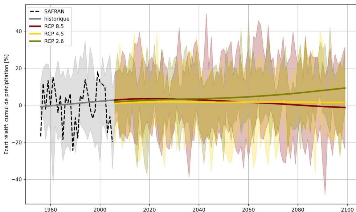
Figure 22 : Évolution de l'écart relatif de cumul annuel de précipitations en France Métropolitaine au cours du XXI e siècle, 2006-2100 (par rapport à la normale de référence 1976-2005) pour les trois scénarios RCP2.6 en rouge, RCP4.5 en jaune et RCP8.5 en vert. Le trait continu correspond à la médiane lissée (moyenne glissante sur 10 ans). L'enveloppe de couleur illustre l'intervalle entre l'écart minimal et l'écart maximal de la distribution de l'ensemble des simulations. Sur la période 1976-2005 l'écart par rapport à la normale de référence 1976-2005 ; le trait continu en gris correspond à la médiane lissée des simulations historiques ; l'enveloppe en gris illustre l'intervalle entre l'écart minimal et l'écart maximal de la distribution de l'ensemble des simulations ; le trait discontinu noir sont l'écart des valeurs annuelles non lissé SAFRAN par rapport à la normale SAFRAN 1976-2005.
