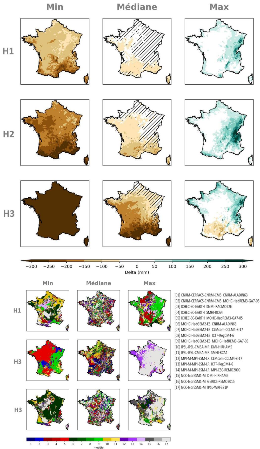
Figure 42 : Cartes des écarts de bilan hydrique annuel (p-eps) à la période de référence par horizon selon le scénario RCP8.5 (multi-horizon, mosaïque, Explore2-2024, ADAMONT).
