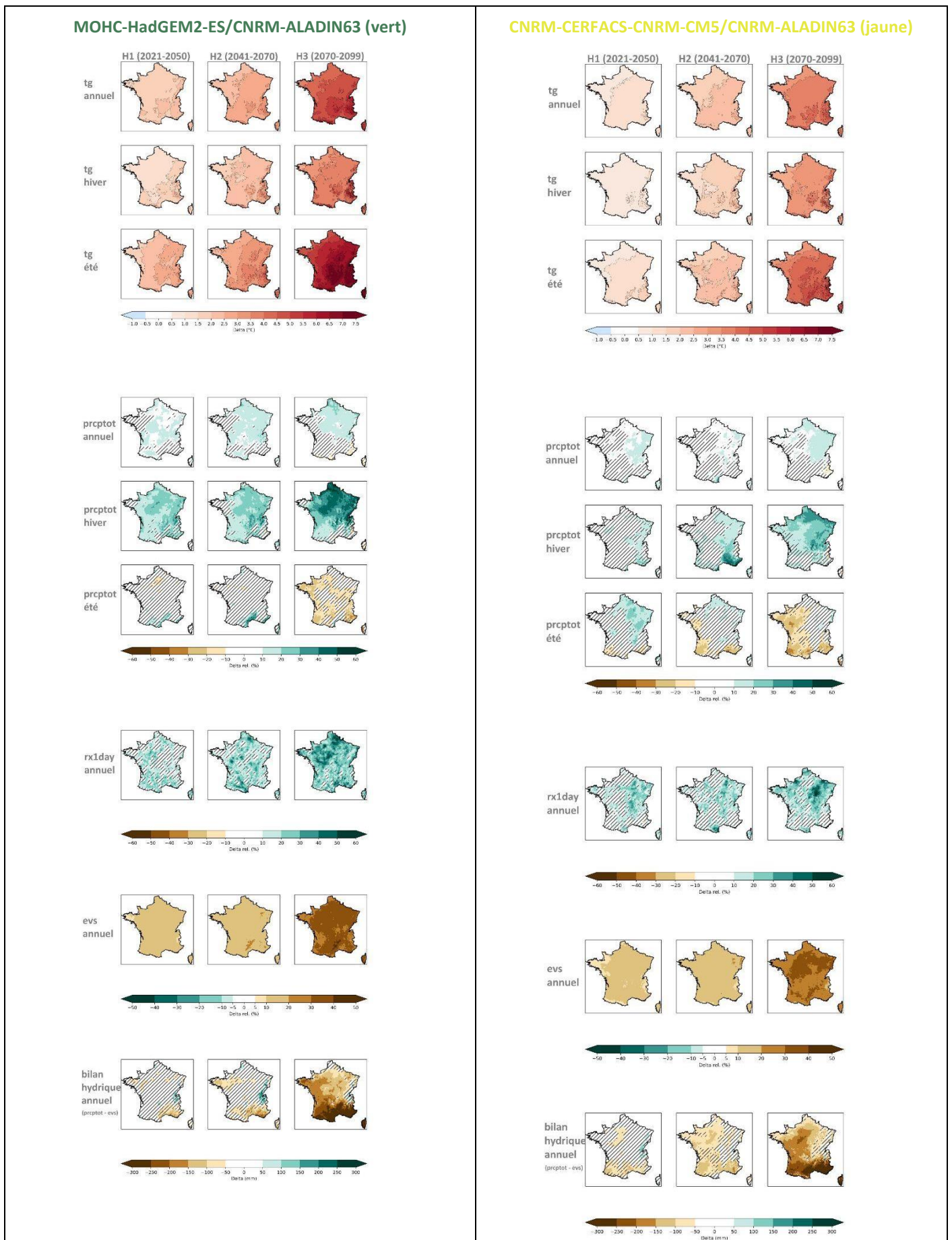
Figure 44 : Changements projetés par les quatre narratifs aux différents horizons.
