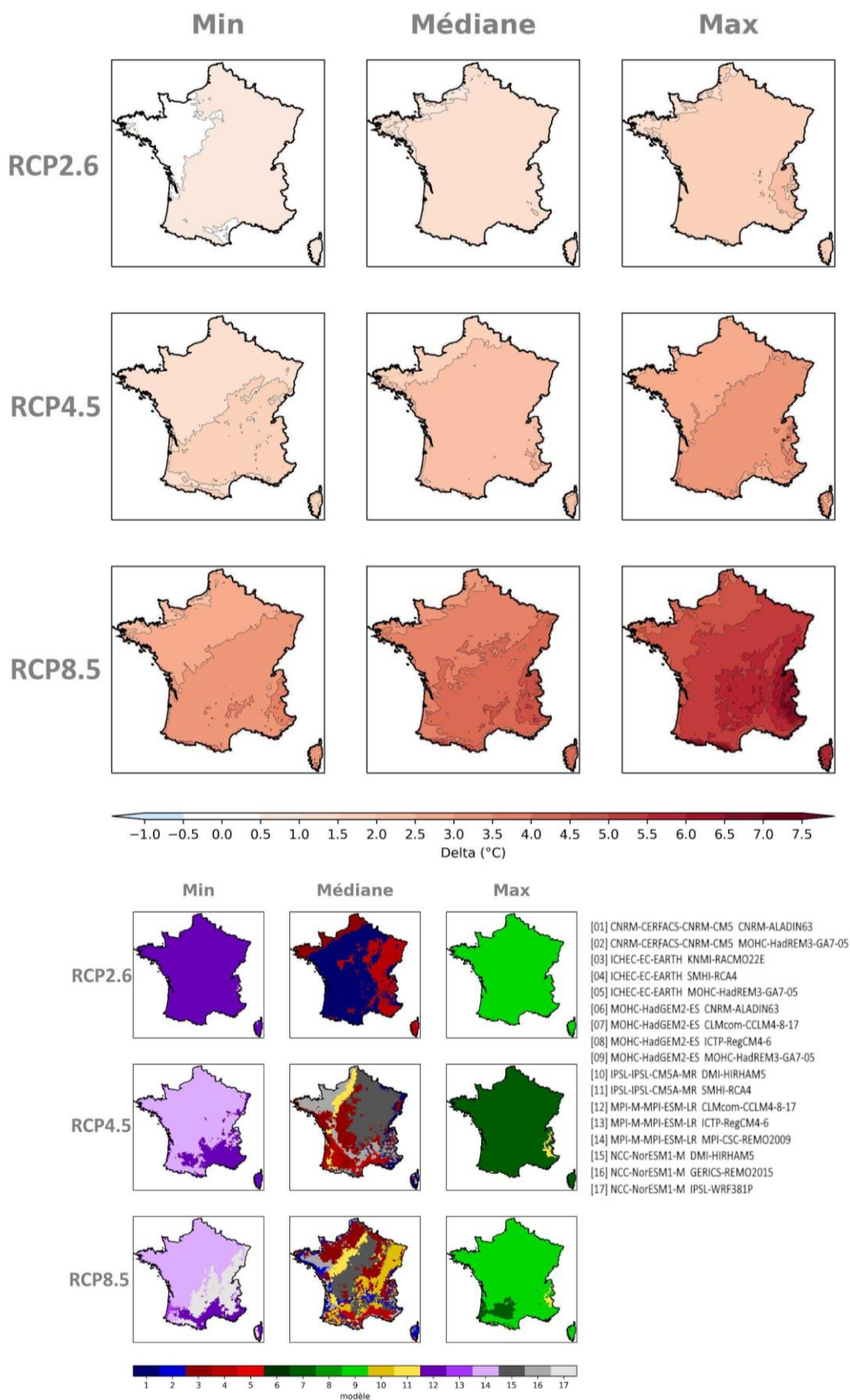
Figure 15 : Cartes des écarts de température moyenne annuelle à la période de référence par scénario RCP à l'horizon lointain (H3, 2070-2099) (multi-scénario, mosaïque, Explore2-2024, ADAMONT).
