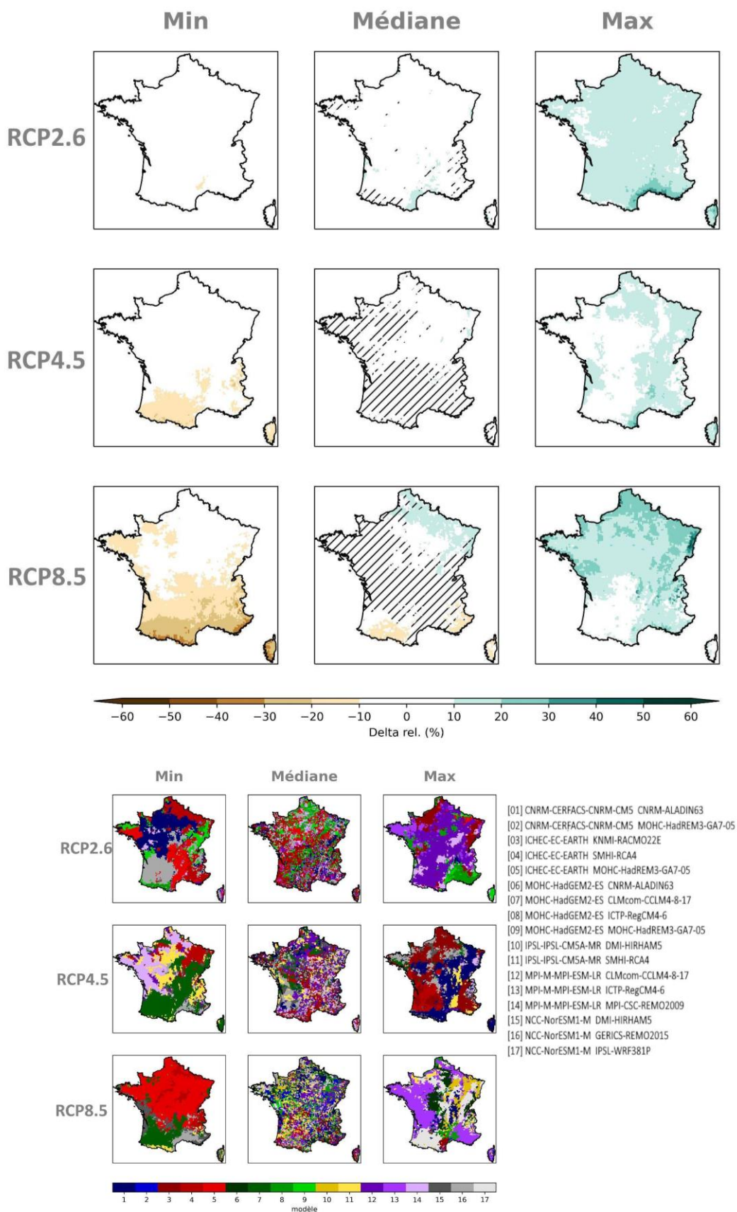
Figure 25 : Cartes des écarts relatifs de cumul annuel de précipitations à la période de référence par scénario RCP à l'horizon lointain (H3, 2070-2099) (multi-scénario, mosaïque, Explore2-2024, ADAMONT).
