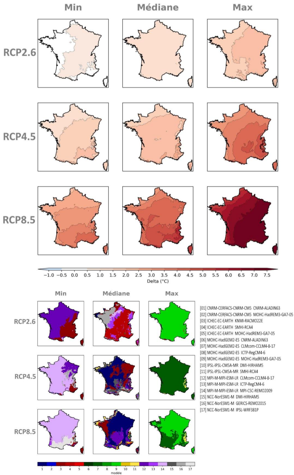
Figure 57 : Cartes des écarts de température moyenne en été à la période de référence par scénario RCP à l'horizon lointain (H3, 2070-2099) (multi-scénario, mosaïque, Explore2-2024, CDF-t).
