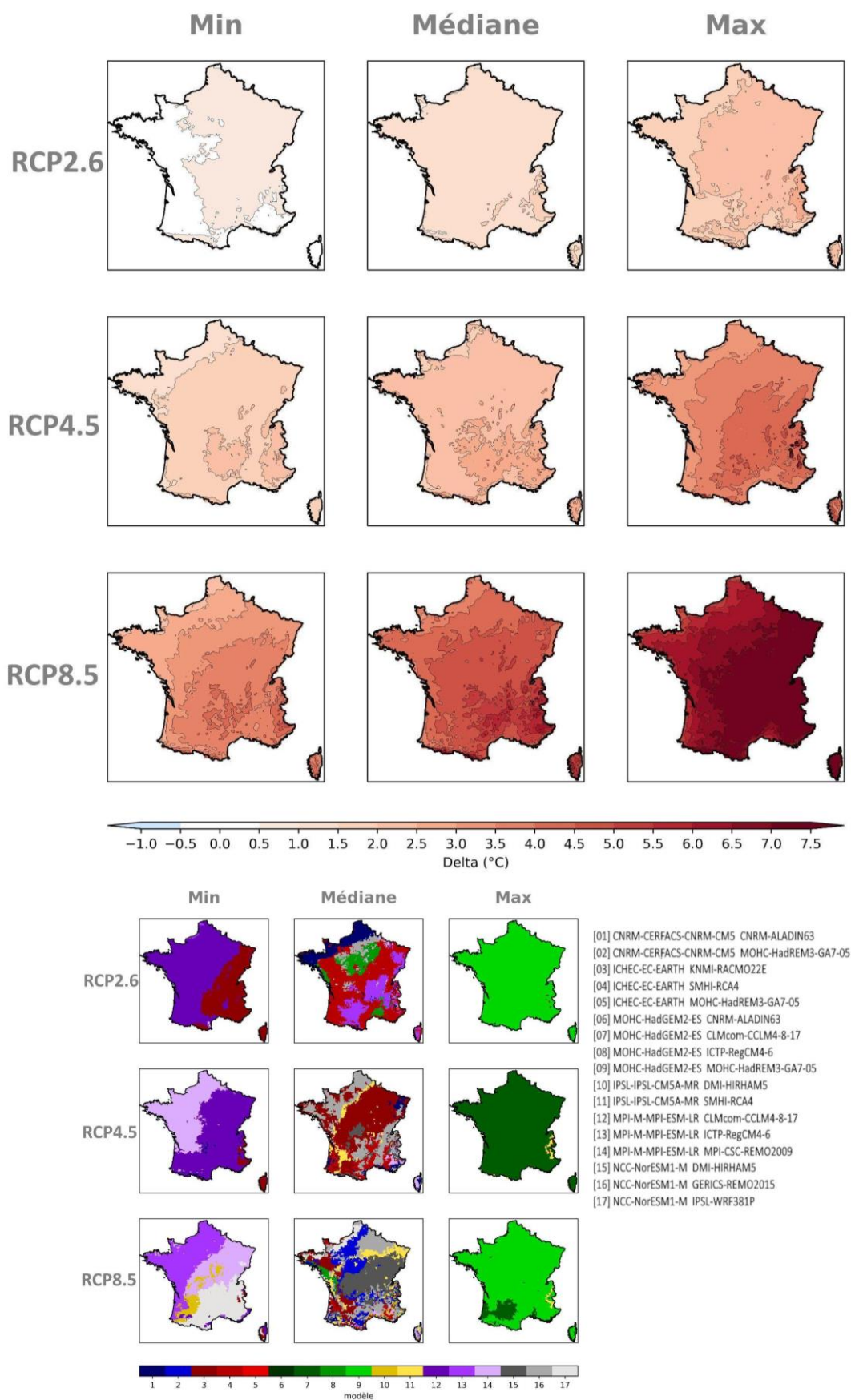
Figure 21 : Cartes des écarts de température moyenne en été à la période de référence par scénario RCP à l'horizon lointain (H3, 2070-2099) (multi-scénario, mosaïque, Explore2-2024, ADAMONT).
