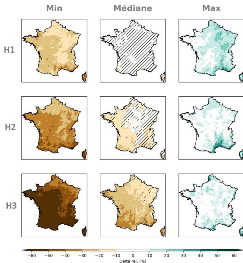
Figure 9 : Exemple de matrice multi-horizon : cartes des écarts relatifs de cumul estival de précipitations selon le scénario RCP8.5 entre l'horizon proche 2021-2050 (première ligne, H1), l'horizon moyen 2041-2070 (deuxième ligne, H2) et l'horizon lointain 2070-2099 (troisième ligne, H3), et la référence 1976-2005. La première colonne correspond par point grille à l'écart minimal dans l'ensemble, la deuxième à l'écart médian et la troisième à l'écart maximal, tous calculés sur l'ensemble Explore2-2024 (méthode ADAMONT).
