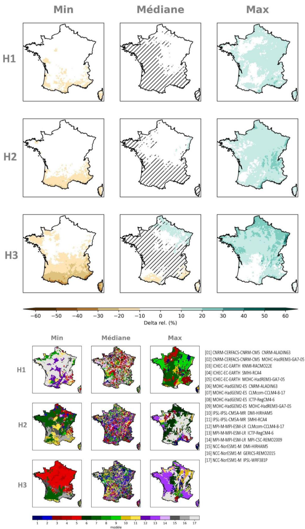
Figure 24 : Cartes des écarts relatifs de cumul annuel de précipitation à la période de référence par horizon selon le scénario RCP8.5 (multi-horizon, mosaïque, Explore2-2024, ADAMONT).
