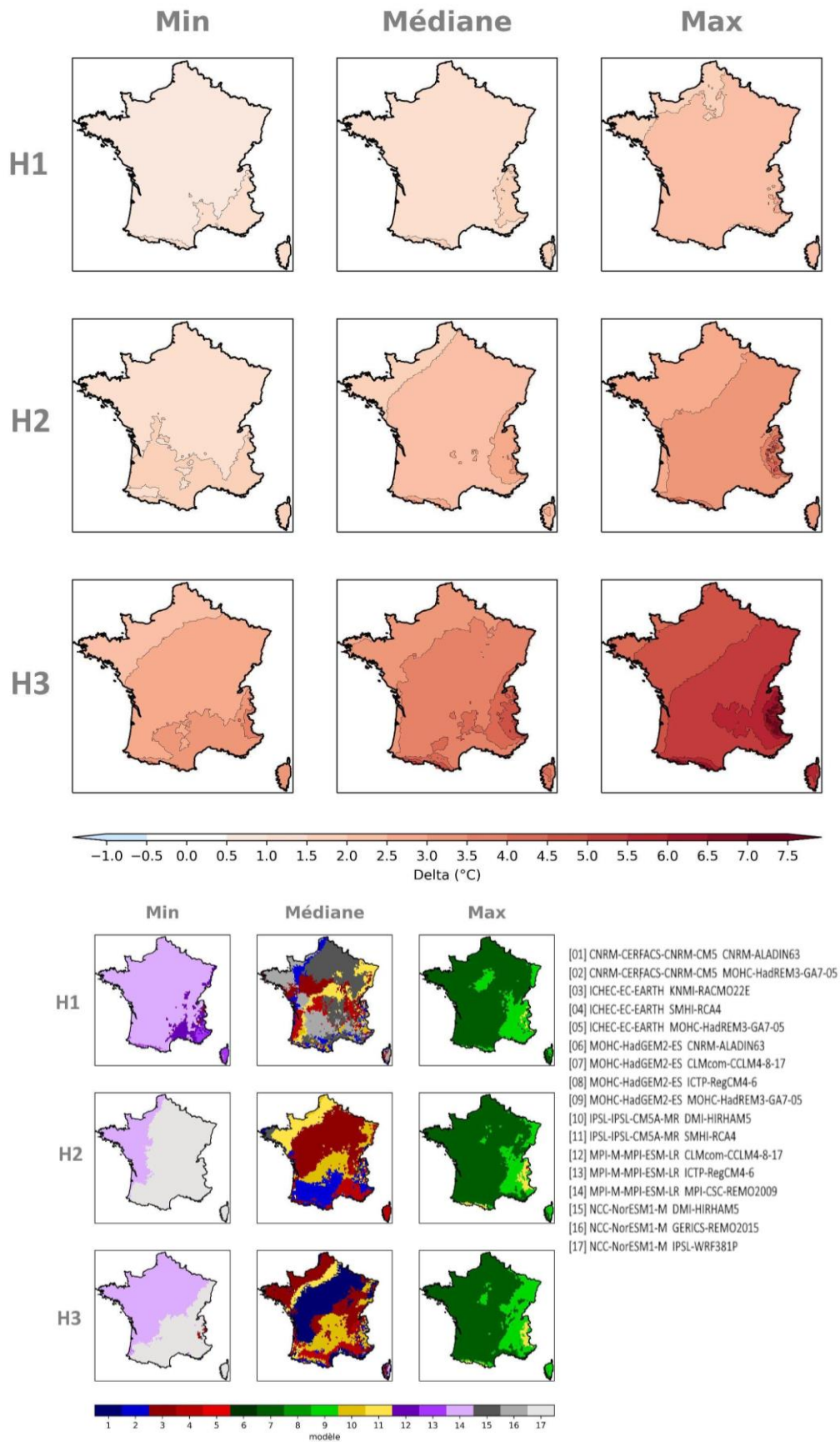
Figure 50 : Cartes des écarts de température moyenne annuelle à la période de référence par horizon selon le scénario RCP8.5 (multi-horizon, mosaïque, Explore2-2024, CDF-t).
