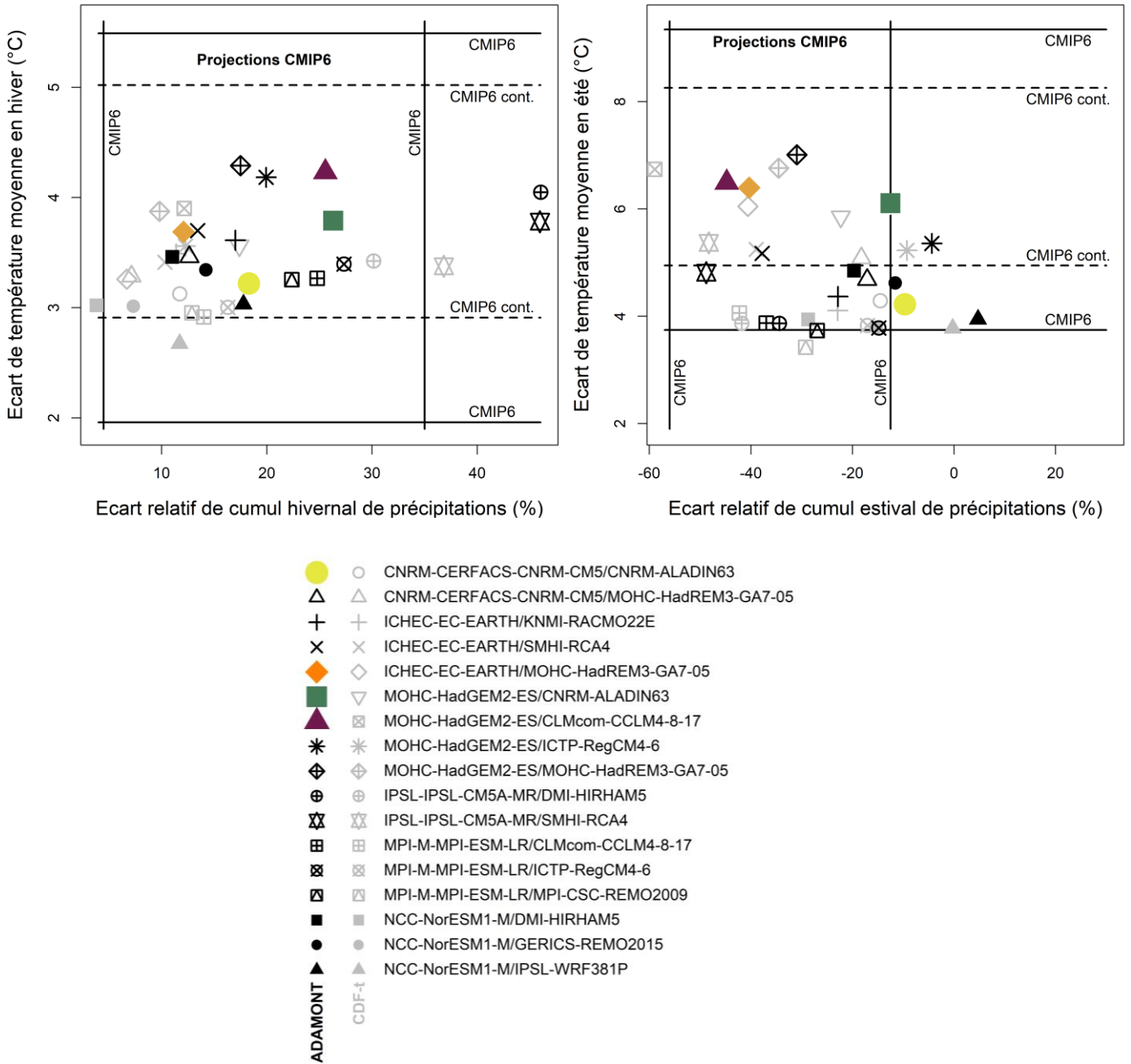
Figure 45 : Changements en température et en précipitations sur la France selon les 34 simulations Explore2-2024 avec identification des quatre narratifs sur les saisons hiver et été, comparés aux quantiles 5 % et 95 % (Q5 et Q95) de l'ensemble CMIP6 (« CMIP6 ») et CMIP6 contraint par les observations pour les températures selon la méthode de Ribes et al. (2022) (« CMIP6 cont. »).
