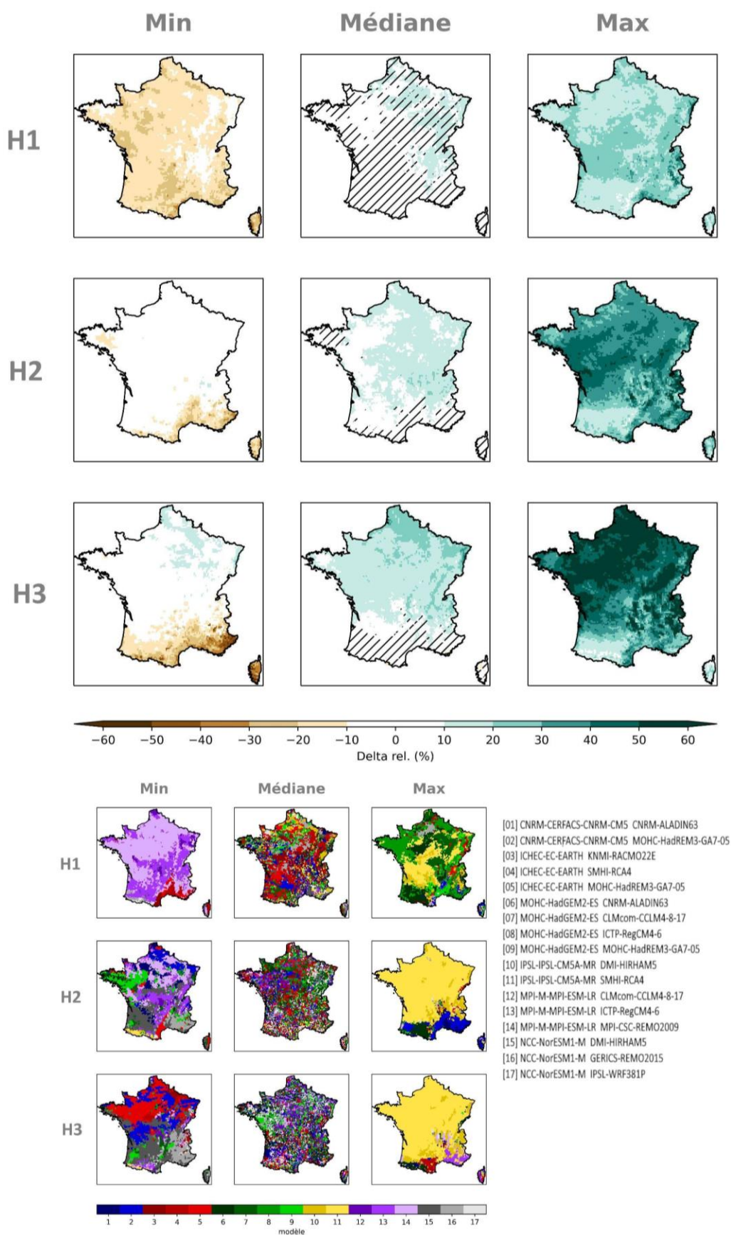
Figure 62 : Cartes des écarts de de cumul hivernal de précipitations par horizon selon le scénario RCP8.5 (multi-horizon, mosaïque, Explore2-2024, CDF-t).
