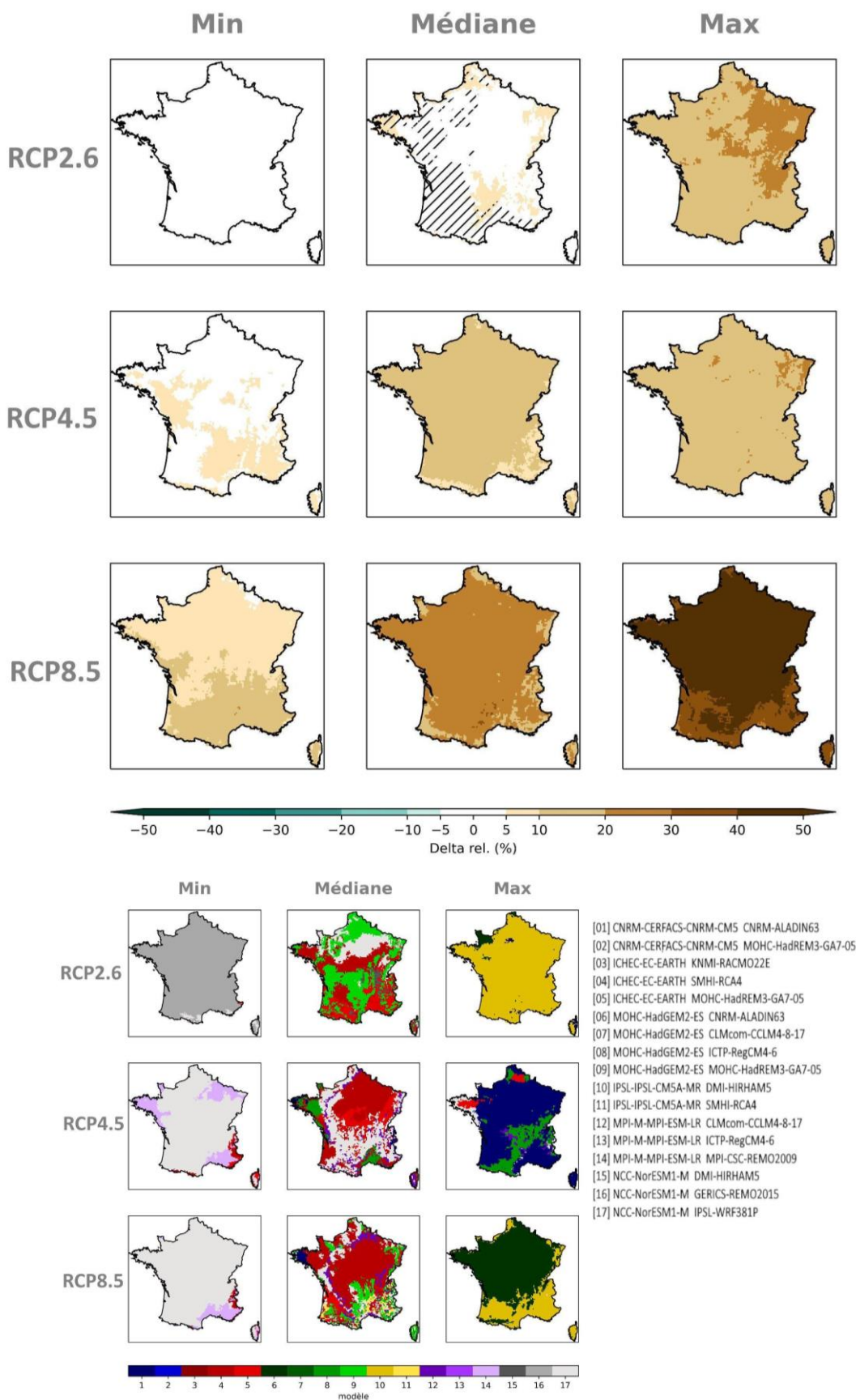
Figure 39 : Cartes des écarts d'évapotranspiration de référence annuelle à la période de référence par scénario RCP à l'horizon lointain (H3, 2070-2099) (multi-scénario, mosaïque, Explore2-2024, ADAMONT).
