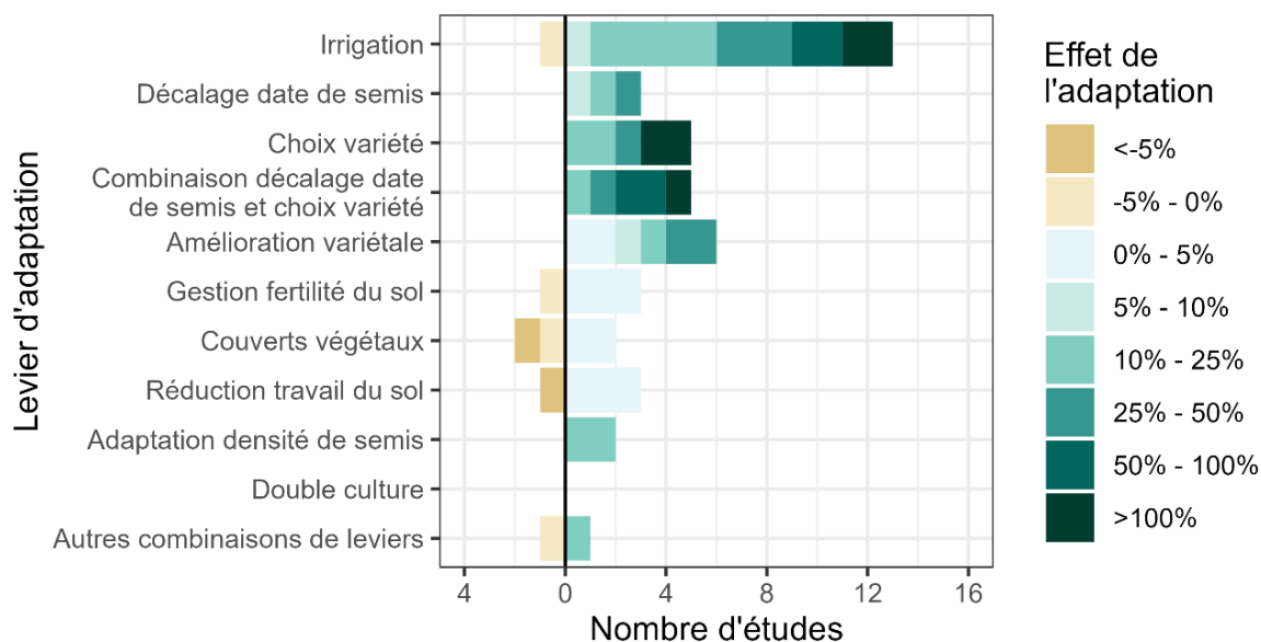
Figure 3 : Effet de différents leviers d'adaptation sur le rendement des légumineuses à graines. L'effet de l'adaptation est défini comme suit : \text{Effet de l'adaptation} = (\text{Rendement avec adaptation} - \text{Rendement sans adaptation}) / \text{Rendement sans adaptation} . Faute de données brutes accessibles, seules 34 études sur 53 ont pu être intégrées dans cette figure.
