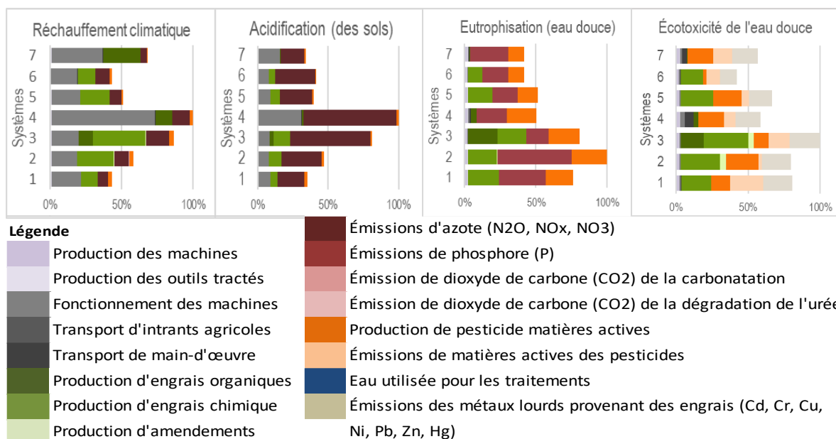
Figure 2 : Extrait des résultats de l'ACV comparative sur les parangons des 7 groupes d'itinéraires techniques cognacais 2019, méthode Recipe 2016, UF Hectare (Billaud, 2021)
