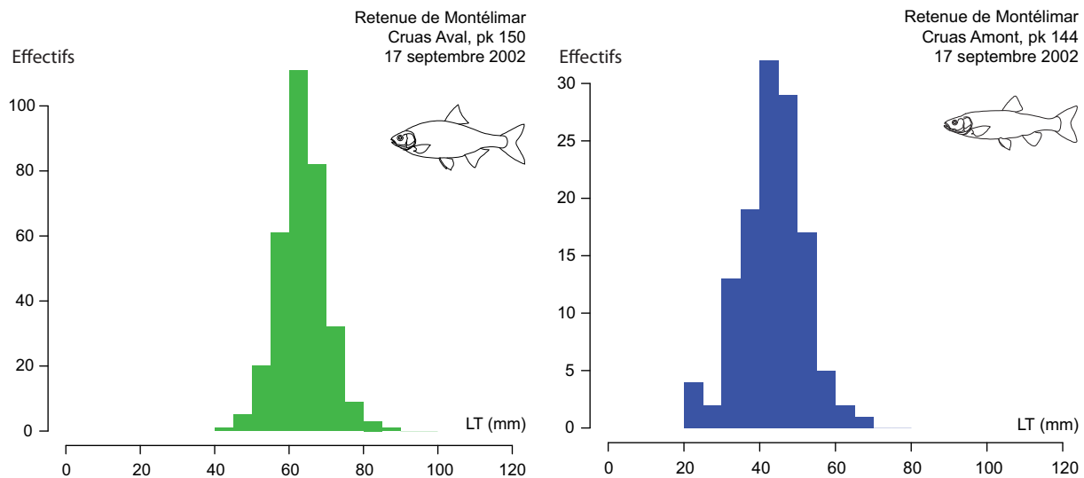
Figure 8 - Distribution en classes de taille du gardon (en vert) et du chevaîne (en bleu) montrant les effets potentiels de leur stratégie de ponte sur la forme de la distribution et son amplitude. Retenue de Montélimar le 17 septembre 2009.
