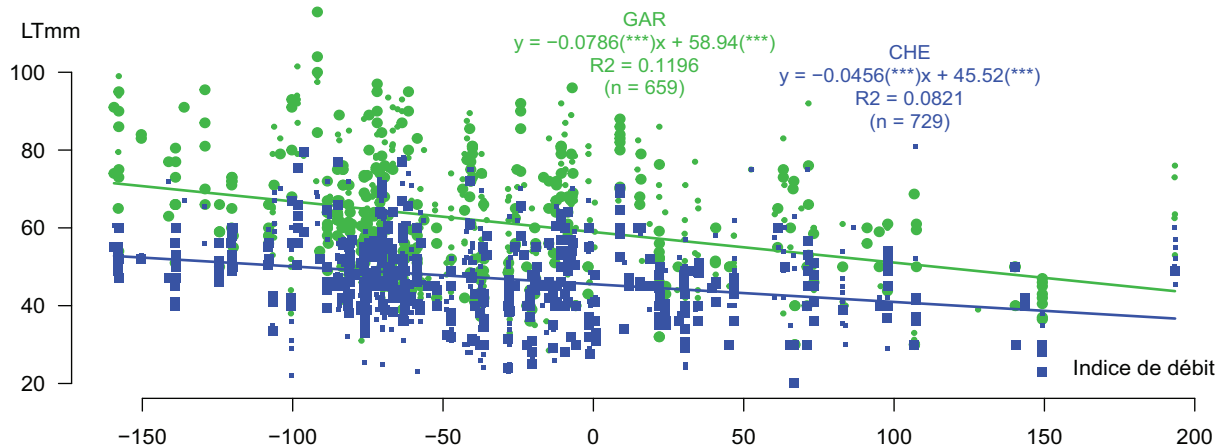
Figure 30 - Régression de la LT médiane de chaque pêche sur l'indice de débit pour le gardon (vert) et le chevaïne (bleu). La taille des points correspond à leur poids dans le modèle ( \times 0.5 lorsque le nombre d'individus dans la pêche est inférieur à 30 et \times 1 lorsqu'il est supérieur à 30). Les pêches faites à proximité des rejets de centrales ont été retirés des analyses.
