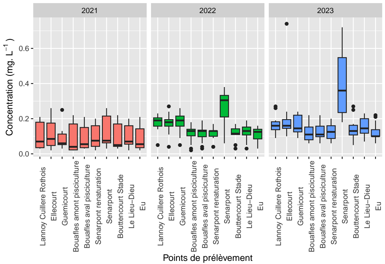
Figure II.11. Boxplot des concentrations en orthophosphates mesurées annuellement sur chaque point de prélèvement.
