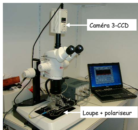
Figure 3 : a- loupe macroscopique binoculaire LEICA-MZ125 b- montage du banc micromécanique sous loupe binoculaire
