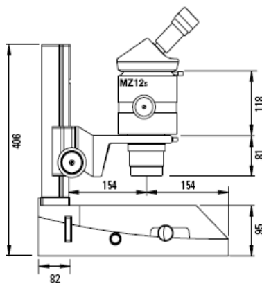
Figure 3 : a- loupe macroscopique binoculaire LEICA-MZ125 b- montage du banc micromécanique sous loupe binoculaire
