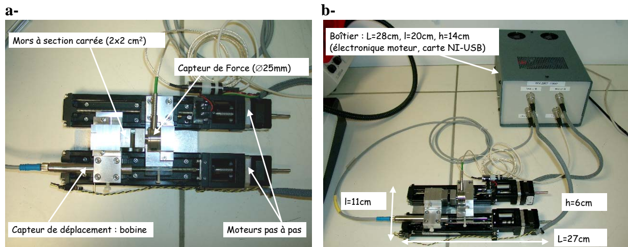
Figure 2 : a- banc instrumenté b- banc et boîtier électronique
