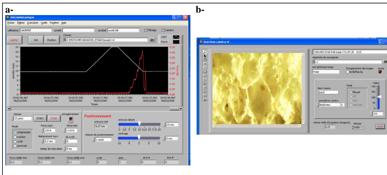
Figure 4 : face-avant du programme de pilotage et acquisition des données. a- banc micro-mécanique, b- acquisition des images (ici dans le cas de la compression d'une mie de pain)
