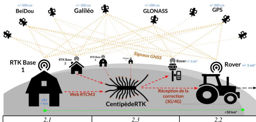
FIGURE 2. CentipedeRTK en 3 segments : 2.1 base ; 2.2 rover et 2.3 caster.
