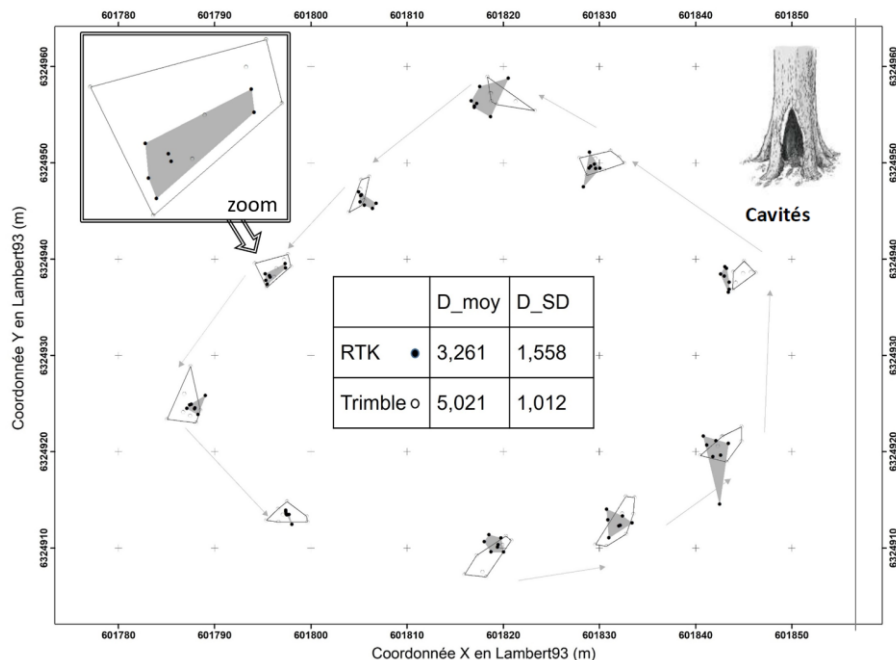
FIGURE 7. Visualisation des données de position d'arbres par le récepteur GNSS de poche Trimble Geo 7x (cercle blanc) et par CentipedeRTK (cercle noir). Chaque amas de points correspond à un arbre, collectés lors de passages successifs le long du parcours. Les enveloppes englobantes des 2 nuages de points par arbre ont été obtenues par SIG (en noir sur les acquisitions CentipedeRTK et en blanc sur celles du Trimble). Les caractéristiques géométriques des enveloppes ont été calculées à savoir la distance la plus longue entre deux sommets de l'enveloppe convexe notée D ( D_{moy} : moyenne et D_{SD} : écart-type en mètres) pour caractériser la dispersion des points (Forêt de Grésigne, France).
