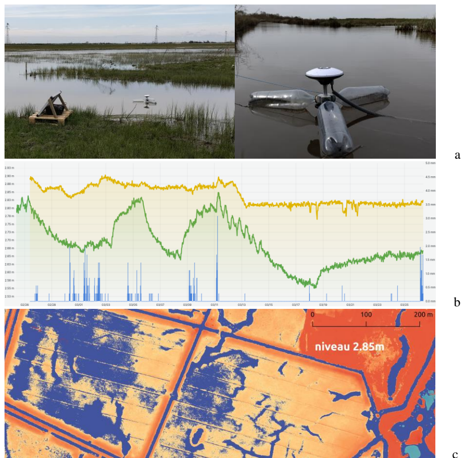
FIGURE 6. Bouées Physalia (a) déployées dans les marais littoraux atlantiques. Les données des niveaux hydrauliques sont disponibles en temps réel sur une interface web accessible par les gestionnaires (b) et permettent la modélisation informatique des surfaces ou volumes d'eau dans les canaux et sur les parcelles (c)
