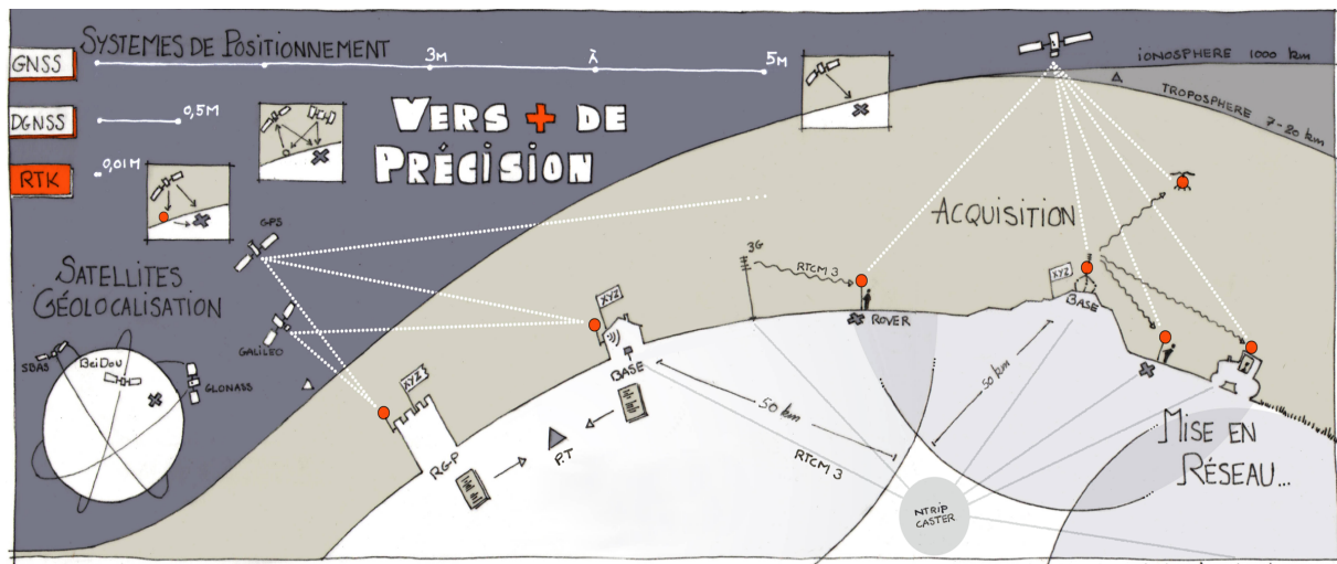
FIGURE 9 – Fonctionnement du système de positionnement par satellite et comparaison des précisions de mesure entre GNSS, DGNS et RTK (famille à laquelle CentipedeRTK appartient).
