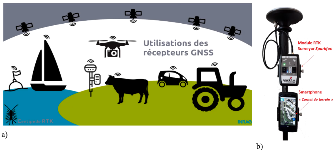
FIGURE 4 – Différents types de rover en fonction des cas d'utilisations (a) et rover de marque Sparkfun équipant une canne (b).
