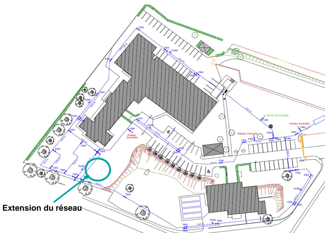
FIGURE 28 : SCHEMA DU RESEAU DE L'OFFICE
