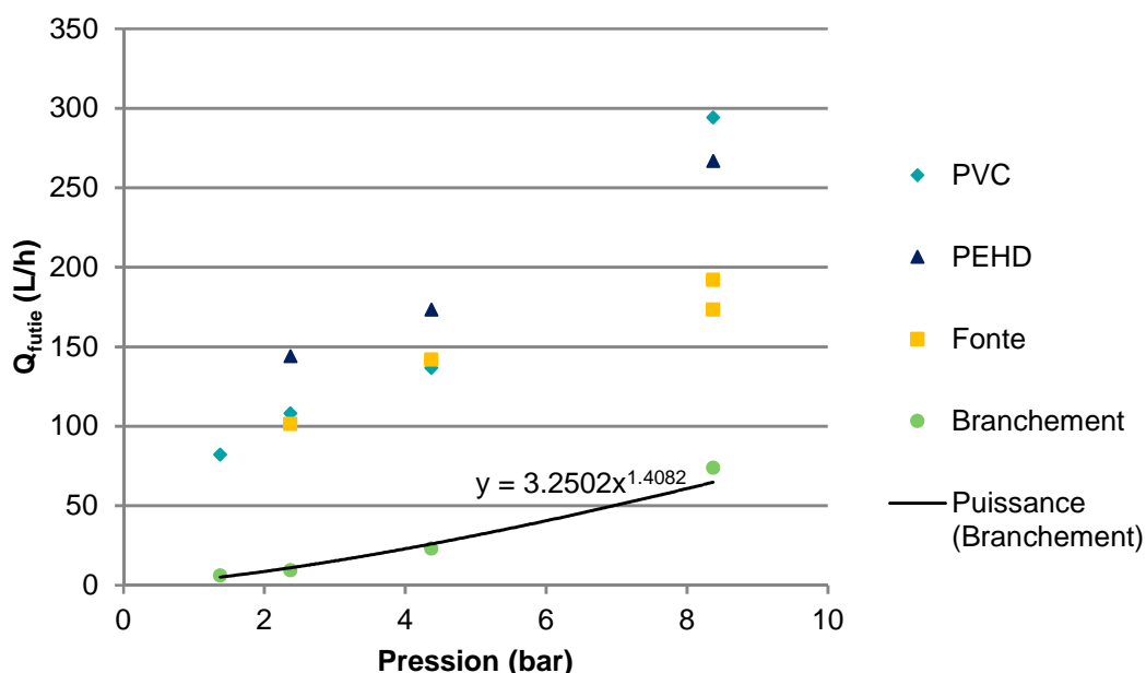
FIGURE 32 : COMPARAISON DE DEBIT DE FUITE A PRESSIONS VARIABLES
