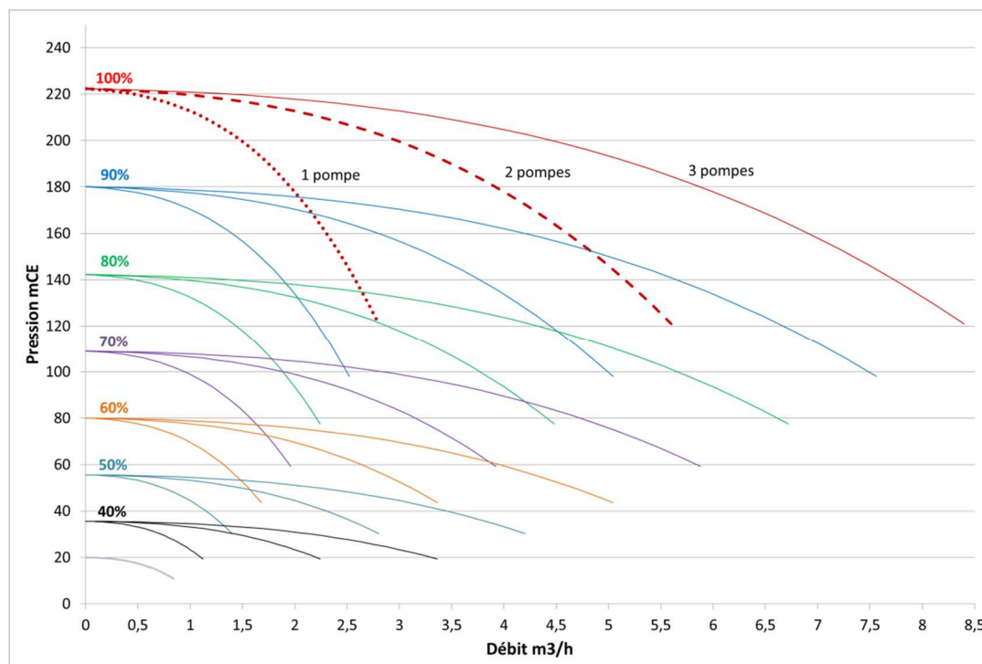
FIGURE 6 : COURBE CARACTERISTIQUE DU SYSTEME DE POMPAGE ASSOCIEE AU PILOTE
