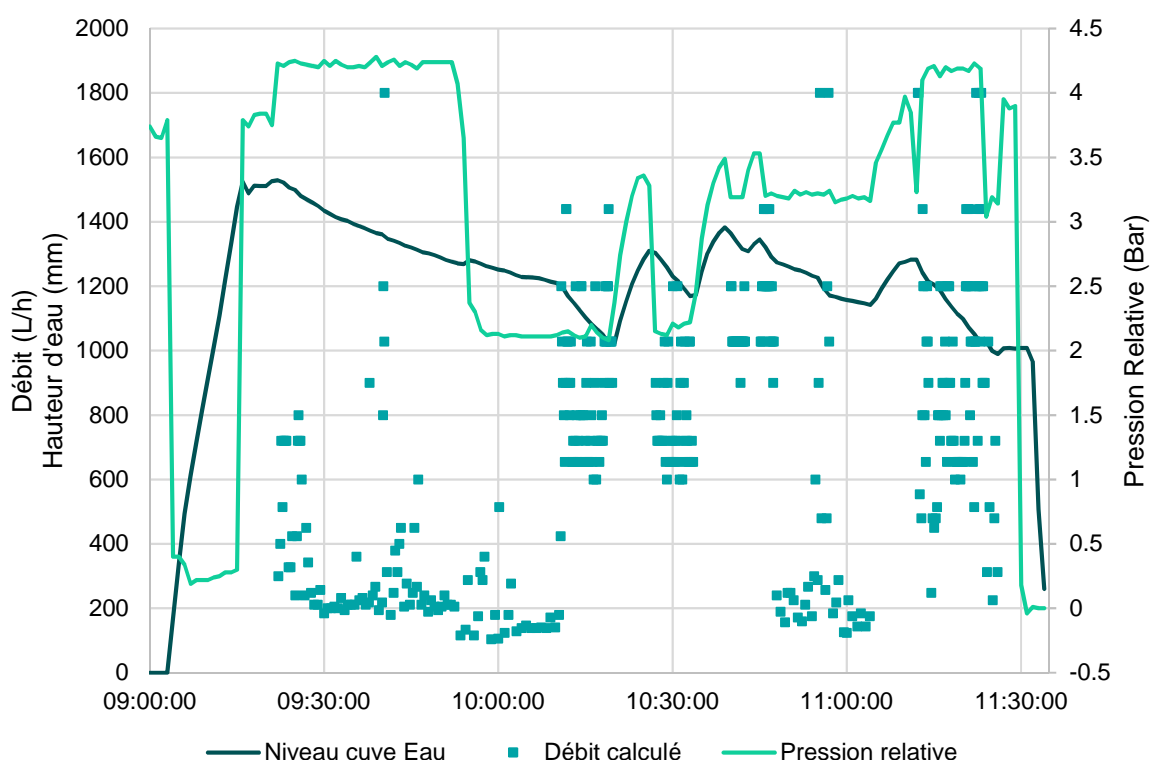
FIGURE 41 : DEBIT DE FUITE DU SECTEUR S2 GARE SUD COUSSAC
