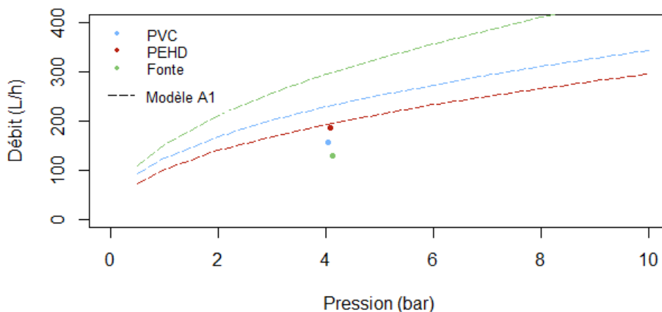
FIGURE 31 : VALEURS DES DEBITS MESURES EN COMPARAISON DU MODELE
