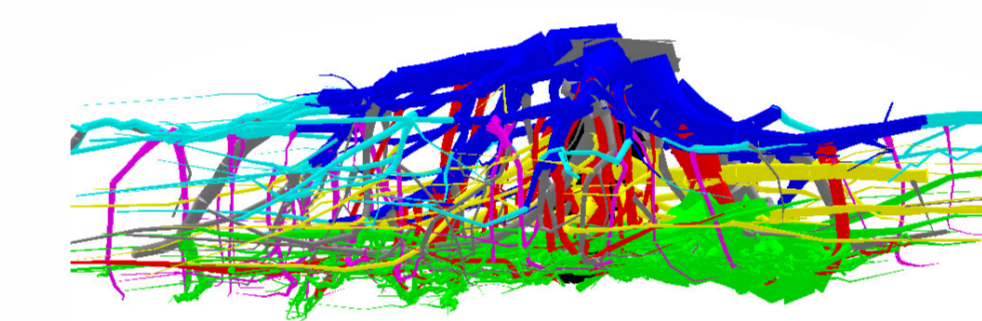
Architecture d'un système racinaire d'un pin maritime âgé de 50 ans sur un sol sableux avec un horizon induré. Les racines sont colorées par type racinaire. On observe une forte acclimatation vis à vis des vents dominants et la limitation de croissance en profondeur liée au type de sol
