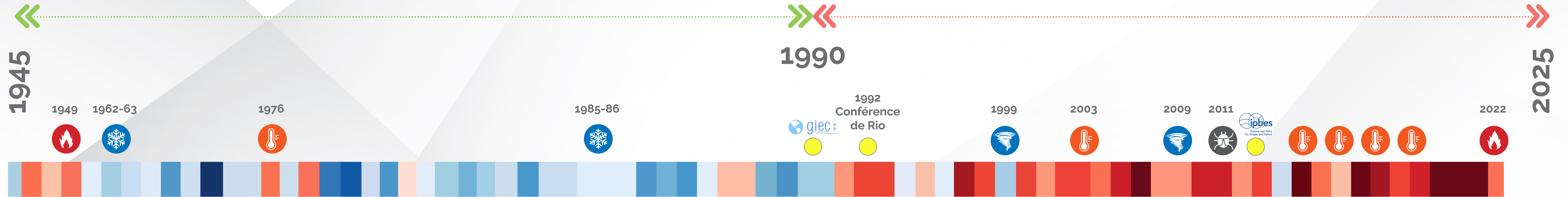
Évolution de la température de la France métropolitaine depuis 1945
