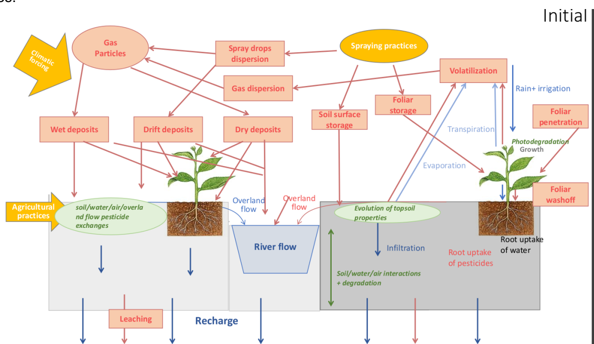
Figure 2 : Principaux processus simulés dans MIPP.
