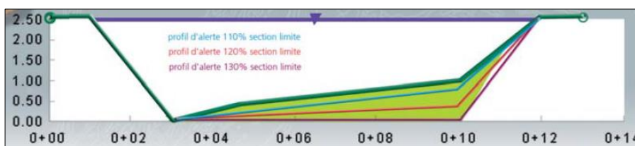
Figure 101 : Exemple de diverses possibilités de choix d'un profil d'alerte. Le choix le plus pertinent n'est possible que si l'on possède une bonne connaissance des apports solides moyens en ce point et des probabilités d'alluvionnement en période de crue (in Malavoi et al., 2011)
