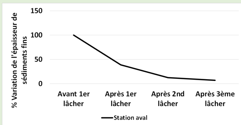
Figure 97 : évolution du colmatage dans le tronçon court-circuité de la Selves après les différents lâchers morphogènes testés (10, 15 et 20 m³/s, Loire et al., 2019).
