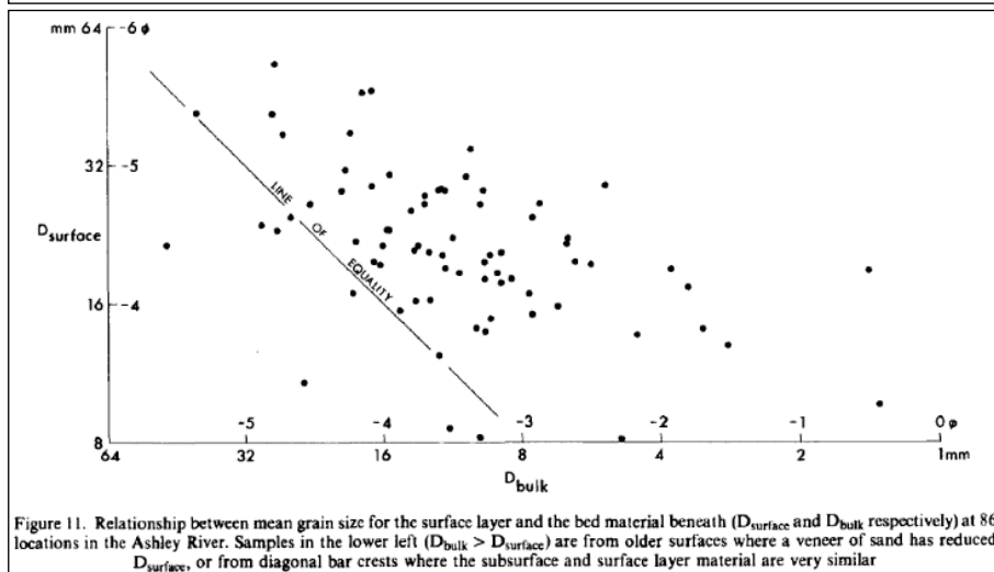
Figure 42 : Illustration de la très grande variabilité granulométrique dans un lit mineur de rivière en tresse. Figures extraites de Mosley et Tindale (1985)
