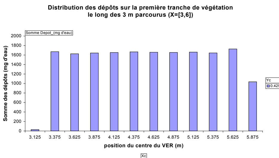
Figure IV-19 : Distribution des dépôts sur la première tranche de VE, le long des 3m parcourus par le tracteur : X_c représente la position du VE dans le sens d'avancement du tracteur et Y_c=0.425 m est la position du centre de la première tranche de VE.
