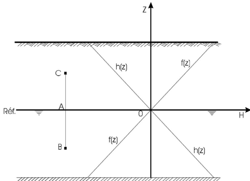
Figure I-1 : Diagramme des potentiels d'un système en équilibre hydrostatique
