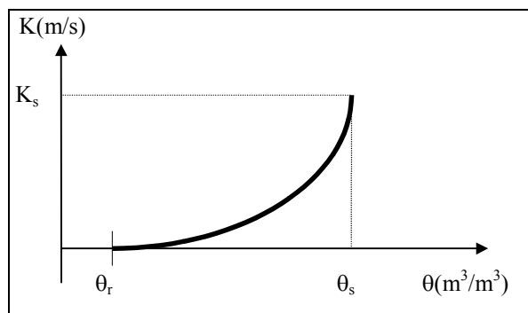
Figure I-5: Variation de la conductivité hydraulique K avec la teneur en eau
