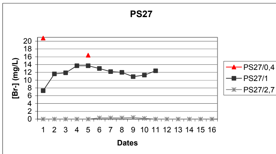
Figure III-35 : Concentrations en bromure en boîtes S27
