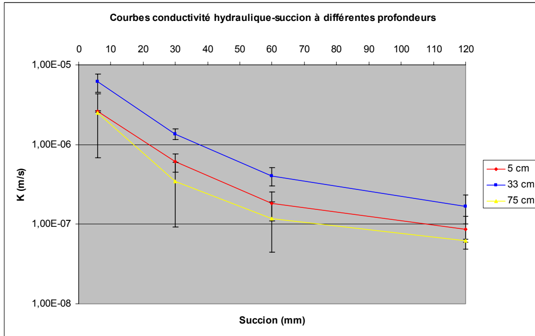
Figure II-21 : Courbes de conductivité hydraulique aux différentes profondeurs
