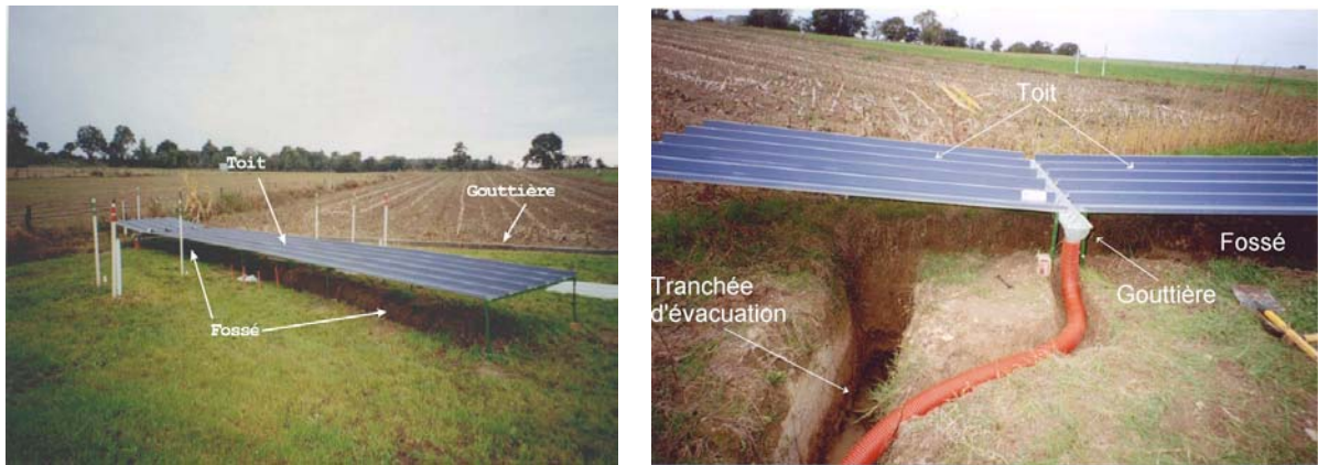
Figure II-8 : a - Toit du fossé, et b - Détail du système d'évacuation de l'eau pluviale.
