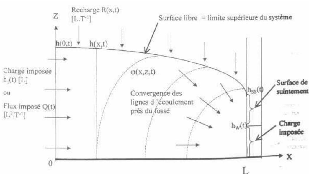
Figure I-14 : Ecoulement saturé bi-dimensionnel. h_{ss}(t) représente la hauteur de la surface de suintement
