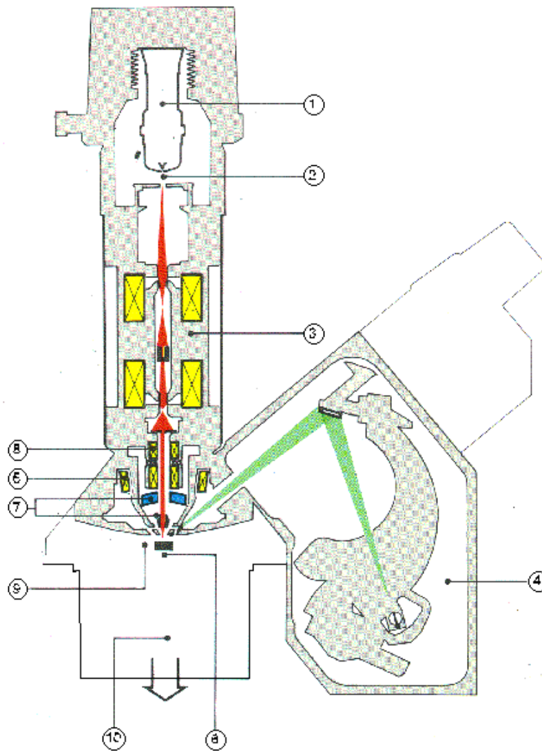
Figure 13: coupe de microsonde X montrant les différentes parties de l'instrument.
