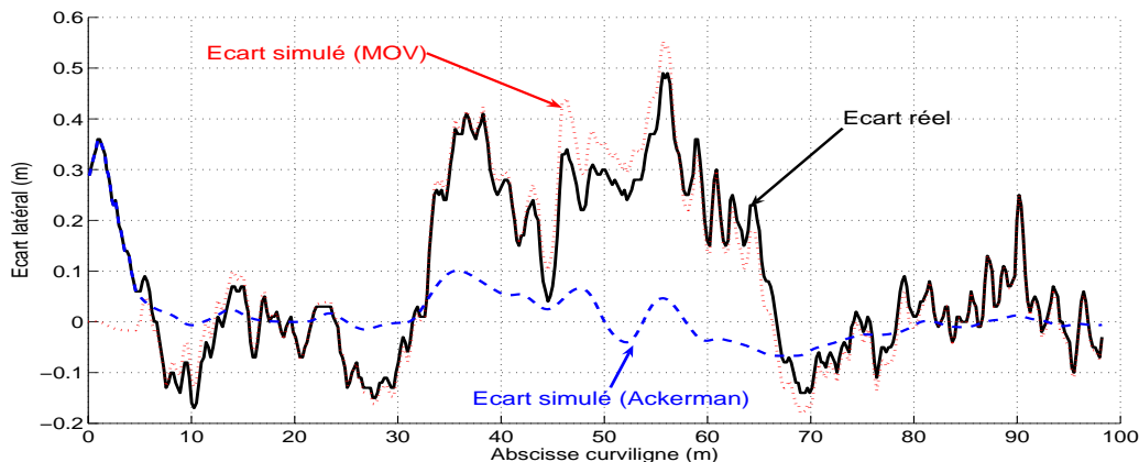
FIG. 3.16 – Écart latéral fourni par MOV en virage
