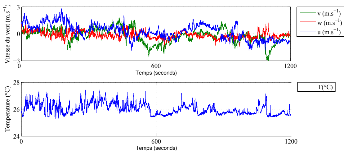
FIG. 3.8 – Série de données acquises par l’anémomètre pendant 20 minutes de mesures. Composantes du vitesse du vent u , v et w et température de l’air, T
