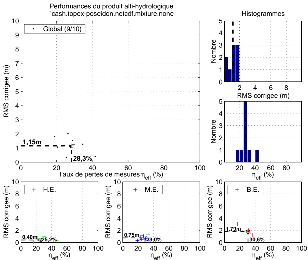
FIG. 7.9: Figure de synthèse pour le produit alti-hydrologique CASH (Topex/Poseidon).
