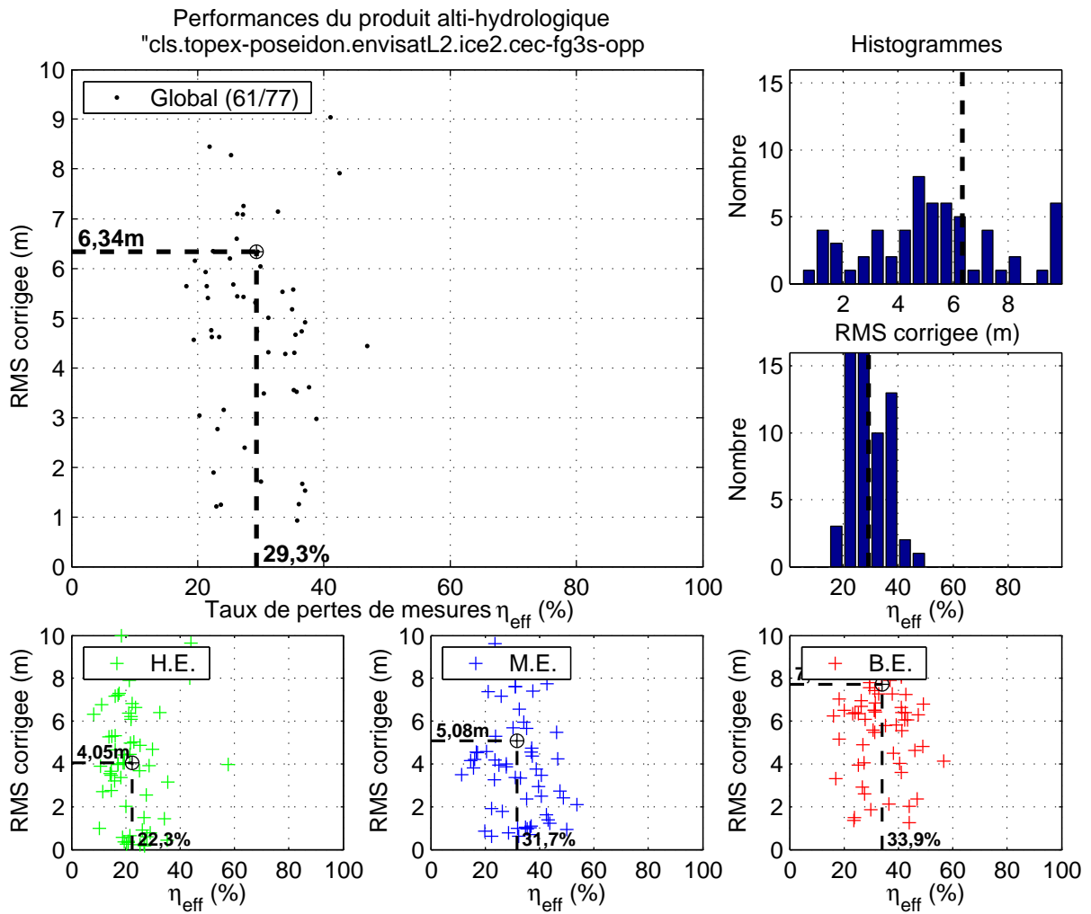
FIG. B.37: Figure de synthèse pour le produit alti-hydrologique « cls.topex-poseidon.envisatL2.ice2.cec-fg3s-opp ».
