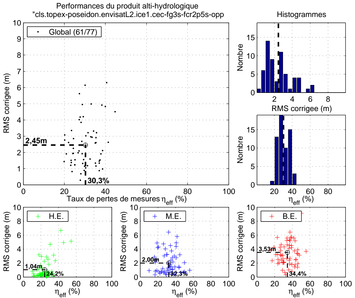
FIG. B.31: Figure de synthèse pour le produit alti-hydrologique « cls.topex-poseidon.envisatL2.ice1.cec-fg3s-fcr2p5s-opp ».
