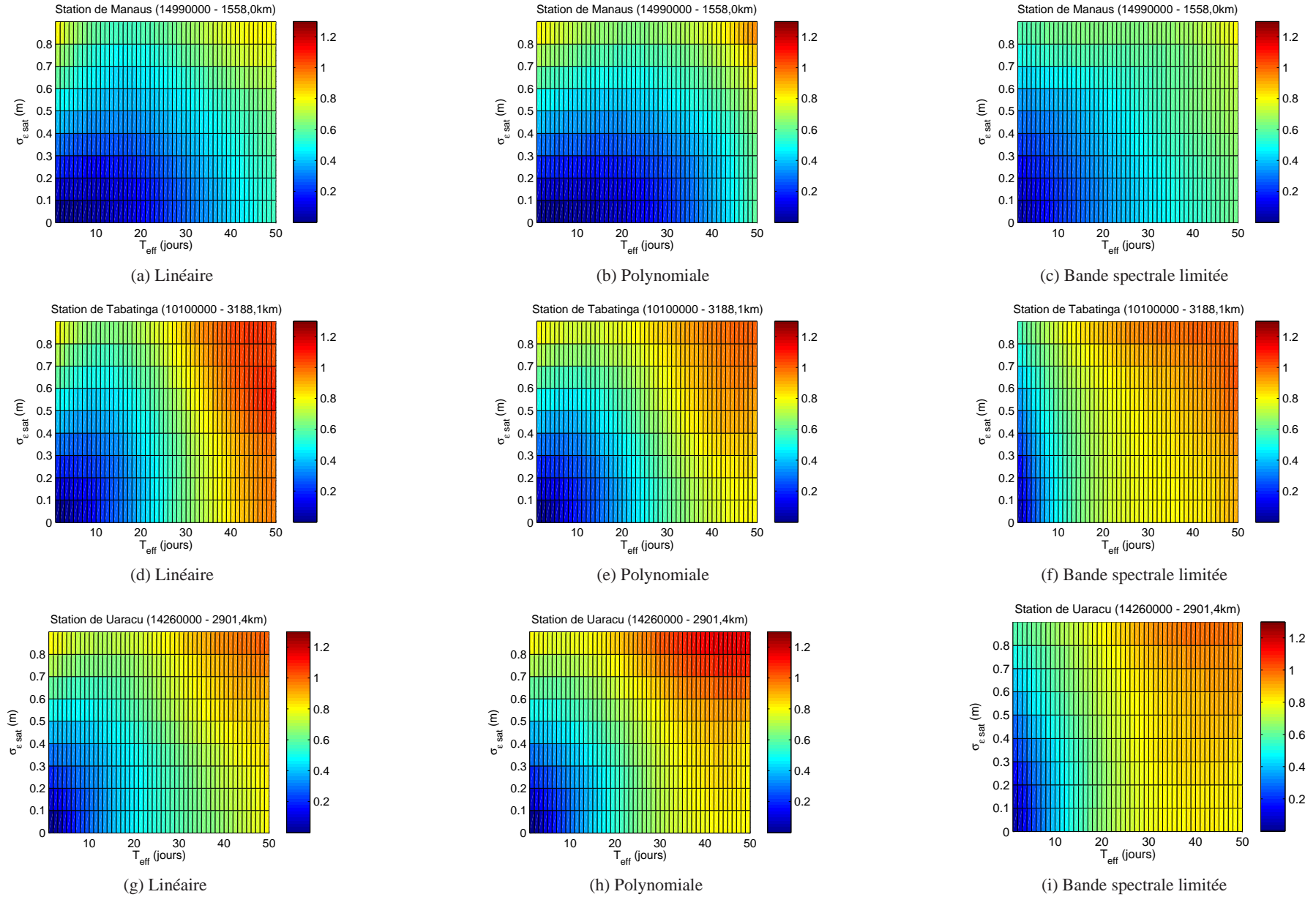
FIG. 9.6: Illustration des effets couplés, sur l'écart-type de l'erreur d'une série temporelle alti-hydrologique suréchantillonnée, d'une technique de suréchantillonnage, d'un bruit de mesure (gaussien centré) pour différentes valeurs de variance et d'un sous échantillonnage pour différentes périodes.
