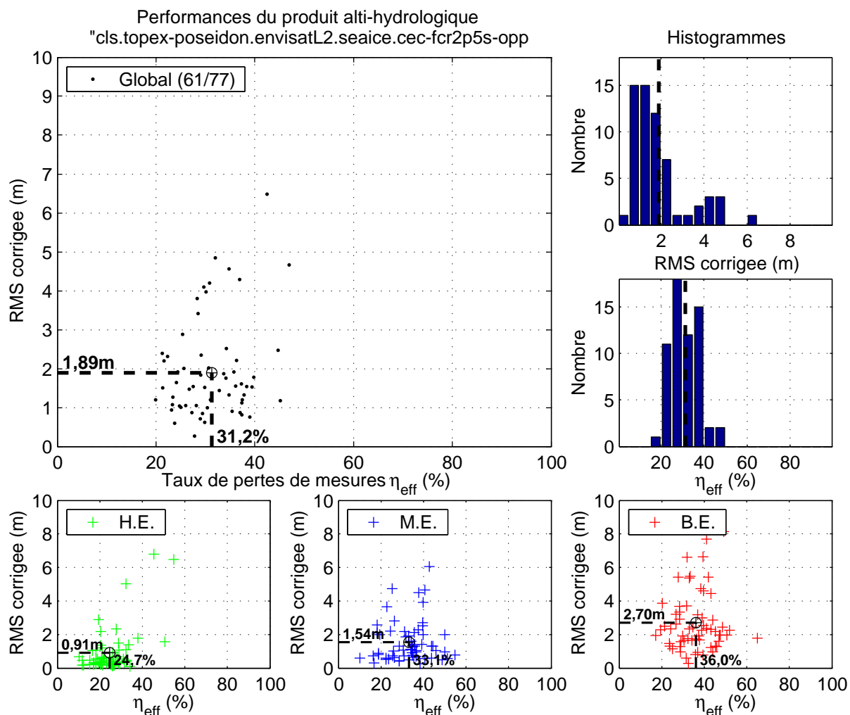
FIG. B.46: Figure de synthèse pour le produit alti-hydrologique « cls.topex-poseidon.envisatL2.seaice.cec-fcr2p5s-opp ».
