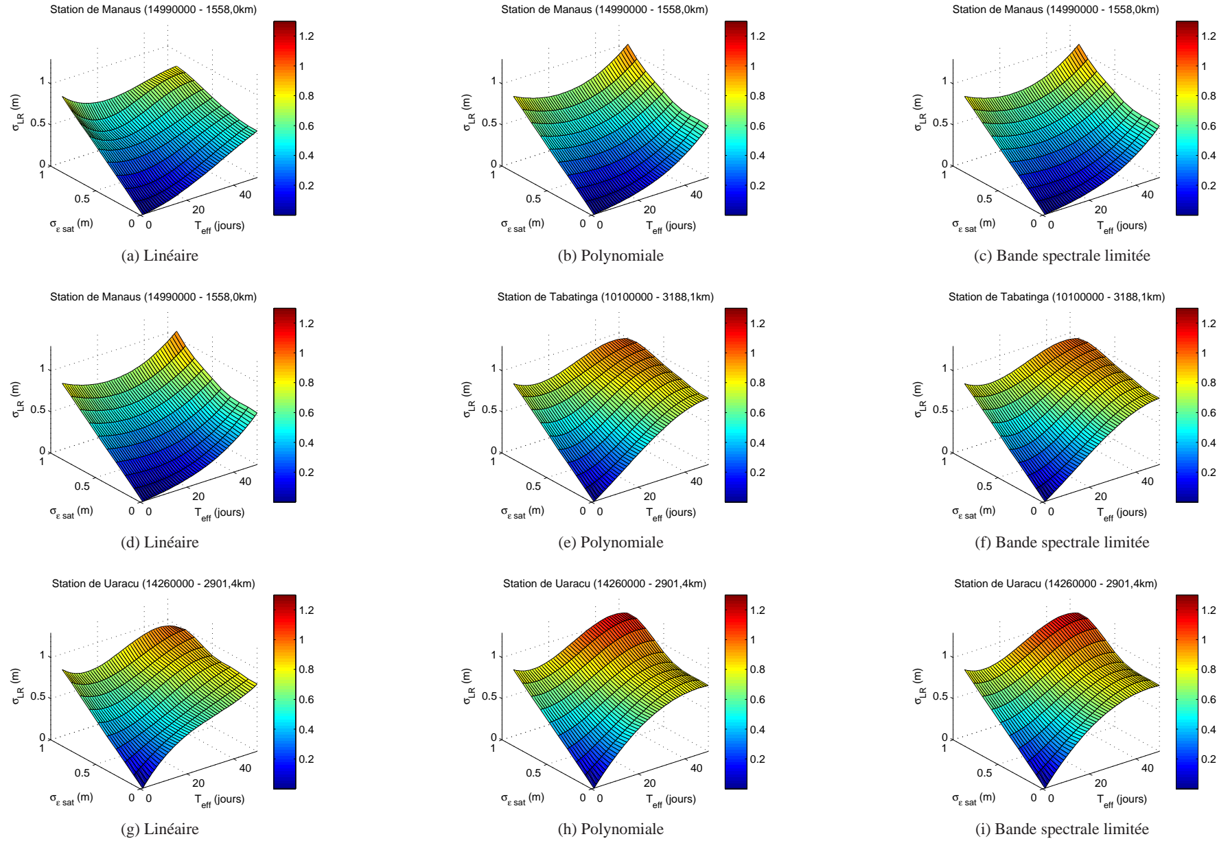
FIG. 9.7: Illustration des effets couplés, sur l'écart-type de l'erreur d'une série temporelle altimétrique suréchantillonnée, d'une technique de suréchantillonnage, d'un bruit de mesure (gaussien centré) pour différentes valeurs de variance et d'un sous échantillonnage pour différentes périodes.
