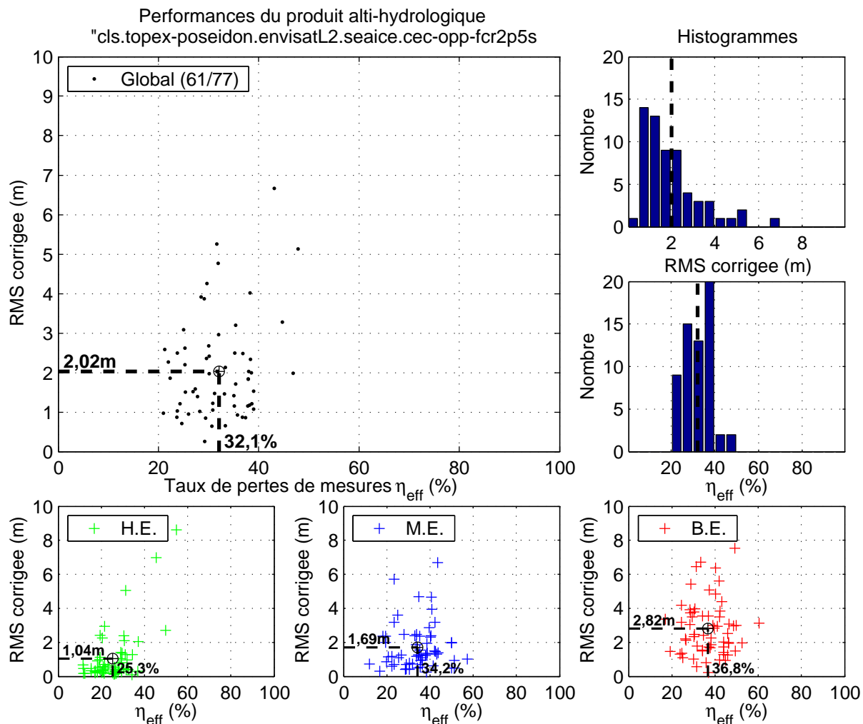
FIG. B.43: Figure de synthèse pour le produit alti-hydrologique « cls.topex-poseidon.envisatL2.seaice.cec-opp-fcr2p5s ».
