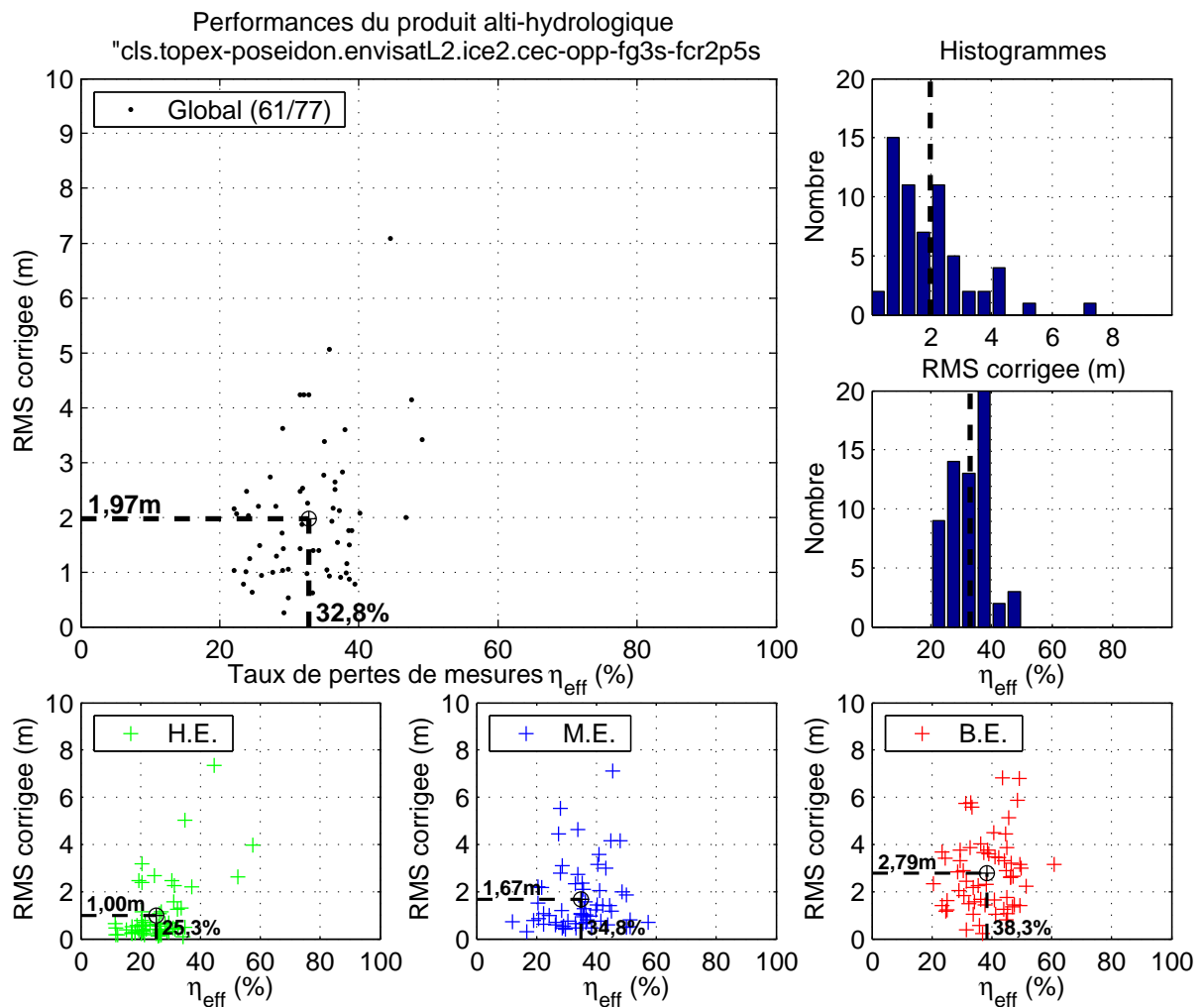
FIG. B.35: Figure de synthèse pour le produit alti-hydrologique « cls.topex-poseidon.envisatL2.ice2.cec-opp-fg3s-fcr2p5s ».
