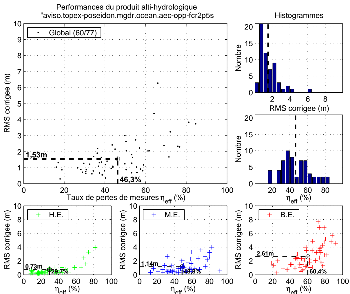
FIG. B.8: Figure de synthèse pour le produit alti-hydrologique « aviso.topex-poseidon.mgdr.ocean.aec-opp-fcr2p5s ».
