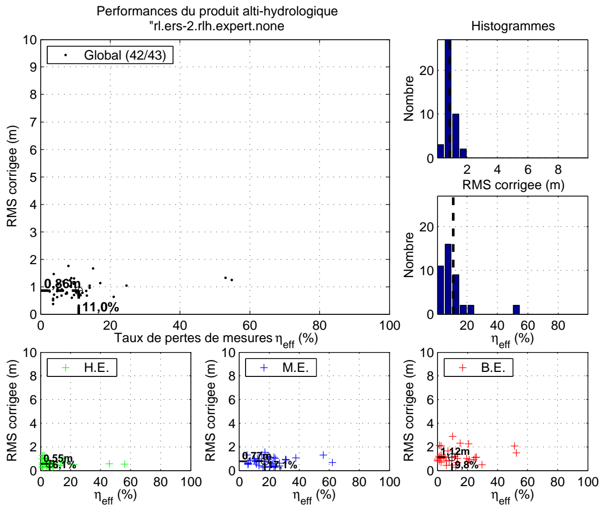
FIG. 7.11: Figure de synthèse pour le produit alti-hydrologique River &amp; Lake Hydrology/ERS-2.
