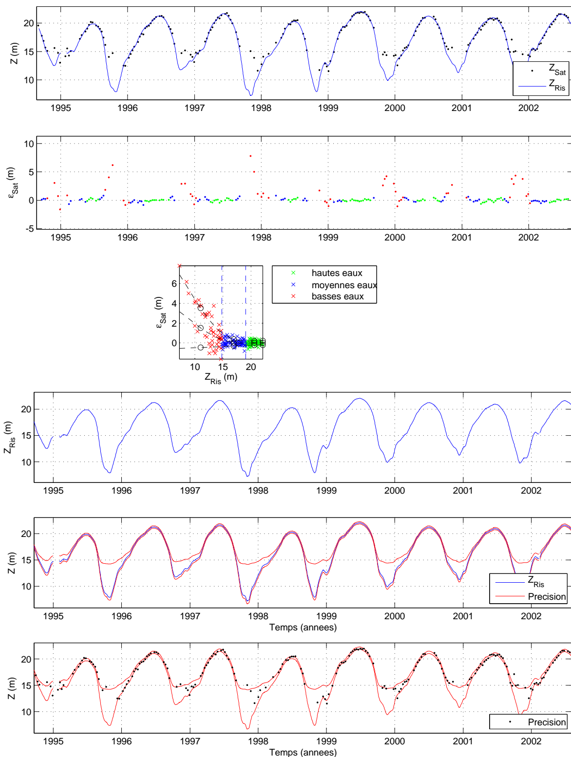
FIG. 8.9: Illustration de la construction d'un modèle de précision des mesures alti-hydrologiques et de son application. L'exemple s'appuie sur une station virtuelle à l'intersection entre la trace 63 de Topex/Poseidon et le fleuve Solimões. De haut en bas : (1) Les deux séries temporelles alti-hydrologique et in-situ reconstituée permettent de construire la série temporelle de l'erreur des mesures altimétriques (2). (3) Le modèle de précision \mathcal{M}_p ( \hat{\mu}_{\mathcal{M}_p} et \hat{\sigma}_{\mathcal{M}_p} ) est construit à partir des indicateurs de précision de l'erreur des mesures alti-hydrologiques par ajustement de courbes (noires en pointillé) sur les points de contrôle (ronds noirs). (4) Série temporelle in-situ reconstituée Z_{Ris} , à laquelle (5) on superpose les limites de précision [\hat{\mu}_{\mathcal{M}_p}(Z_{Ris}) \pm \hat{\sigma}_{\mathcal{M}_p}(Z_{Ris})] . (6) On vérifie que les mesures alti-hydrologiques sont, dans de bonnes proportions ( \sim 91\% des cas), situées dans l'intervalle de précision.
