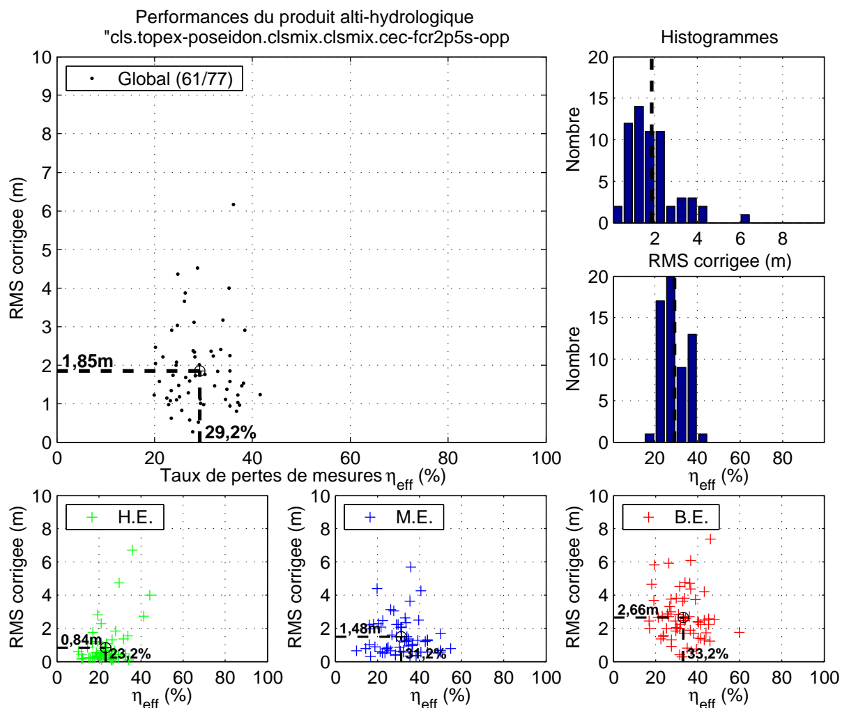
FIG. B.18: Figure de synthèse pour le produit alti-hydrologique « cls.topex-poseidon.clsmix.clsmix.cec-fcr2p5s-opp ».
