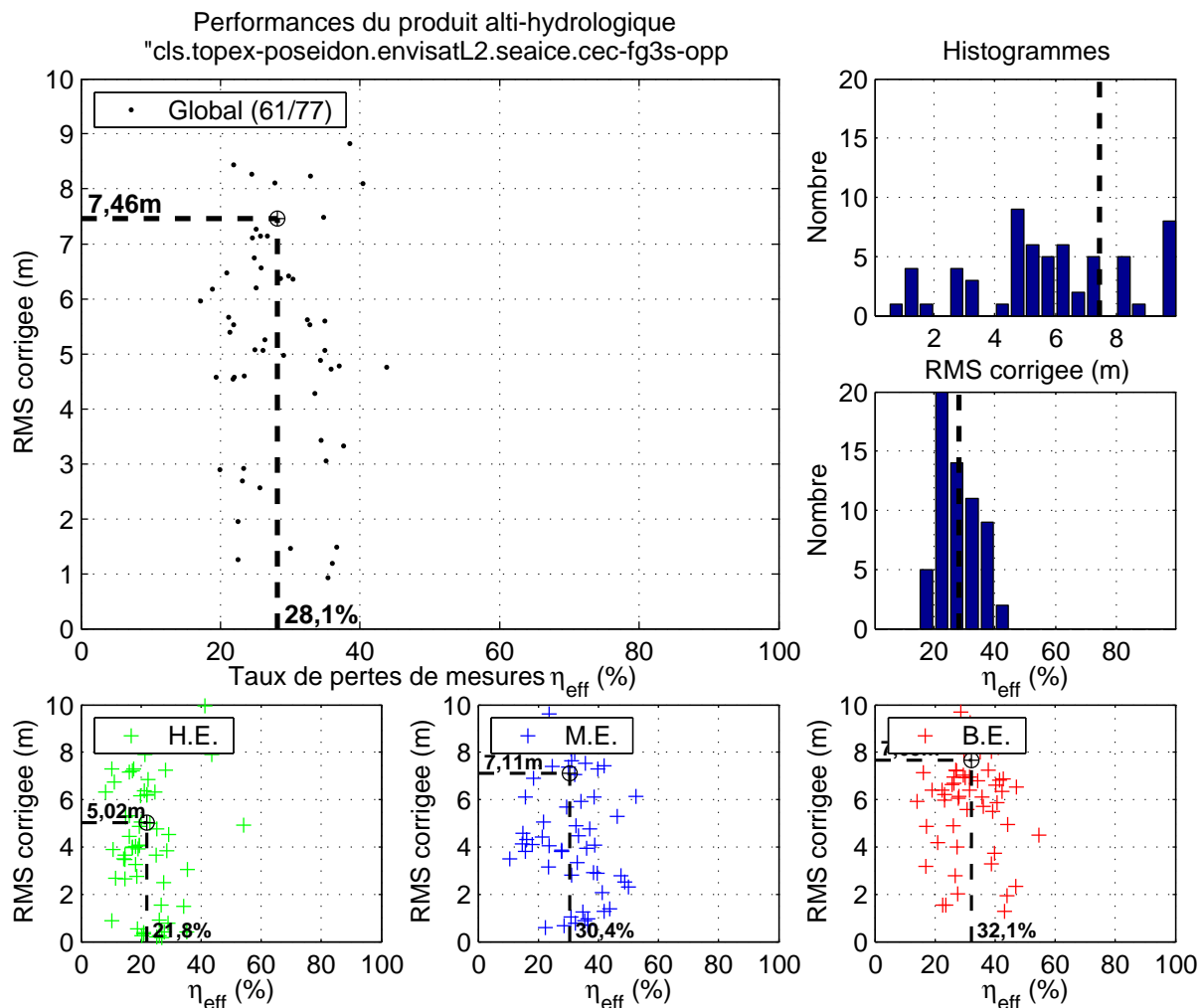
FIG. B.44: Figure de synthèse pour le produit alti-hydrologique « cls.topex- poseidon.envisatL2.seaice.cec-fg3s-opp ».
