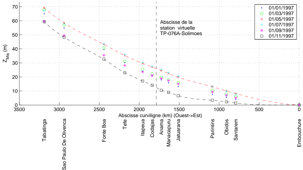
FIG. 5.2: Illustration du profil de la ligne d'eau en fonction de l'abscisse curviligne des fleuves Solimões et Amazone à différentes dates de l'année 1997. Les mesures sont issues de douze stations limnimétriques in-situ dont le nivellement a été réalisé à partir de mesures d'altimétrie radar [Kosuth et al., 2006]. La ligne verticale en pointillés est positionnée sur l'abscisse de la station virtuelle « TP-076A-Solimoes » pour laquelle un exemple de série temporelle in-situ reconstituée est donné à la figure 5.4.
