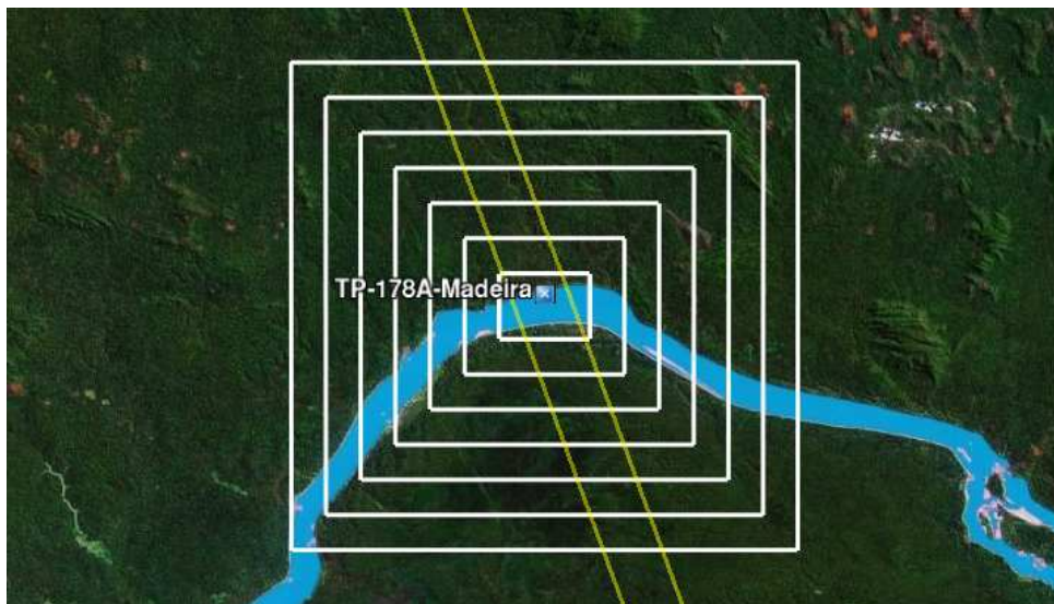
FIG. 7.21: Illustration des 7 options de fenêtrage pour la station virtuelle « TP-178A-Madeira ». Chaque fenêtre est 2km plus large que la précédente, la plus étroite étant ajustée sur les berges du cours d'eau.
