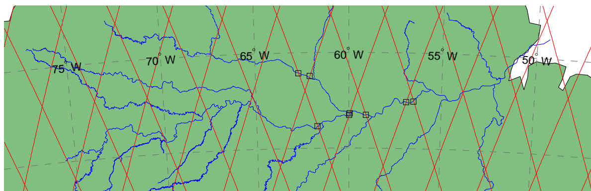
FIG. 7.25: Carte des 8 stations virtuelles sur lesquelles sont comparés les 9 produits alti-hydrologiques CASH, AVISO, CLS et River & Lake Hydrology.
