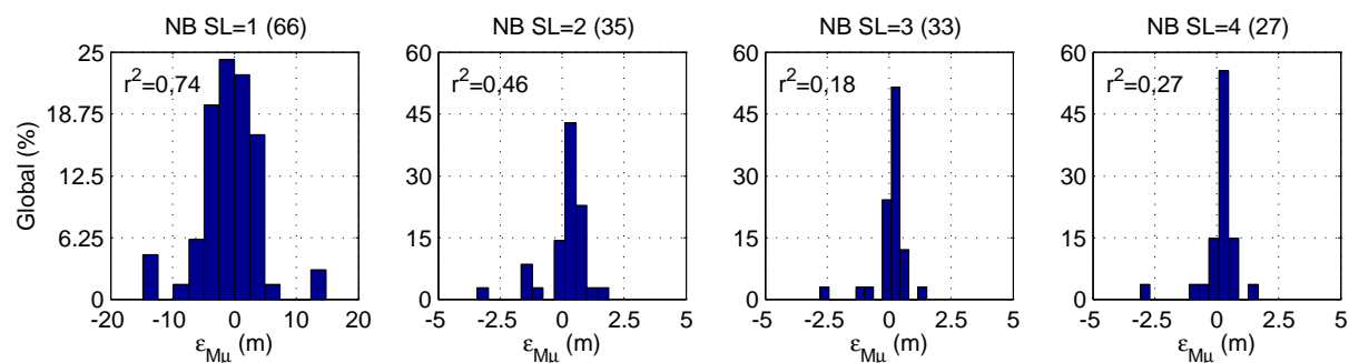
FIG. 6.5: Histogrammes de l'erreur résiduelle ( \varepsilon_{\mathcal{M}} ) des quatre modèles d'estimation de \mu_{\varepsilon_{Rec}} .
