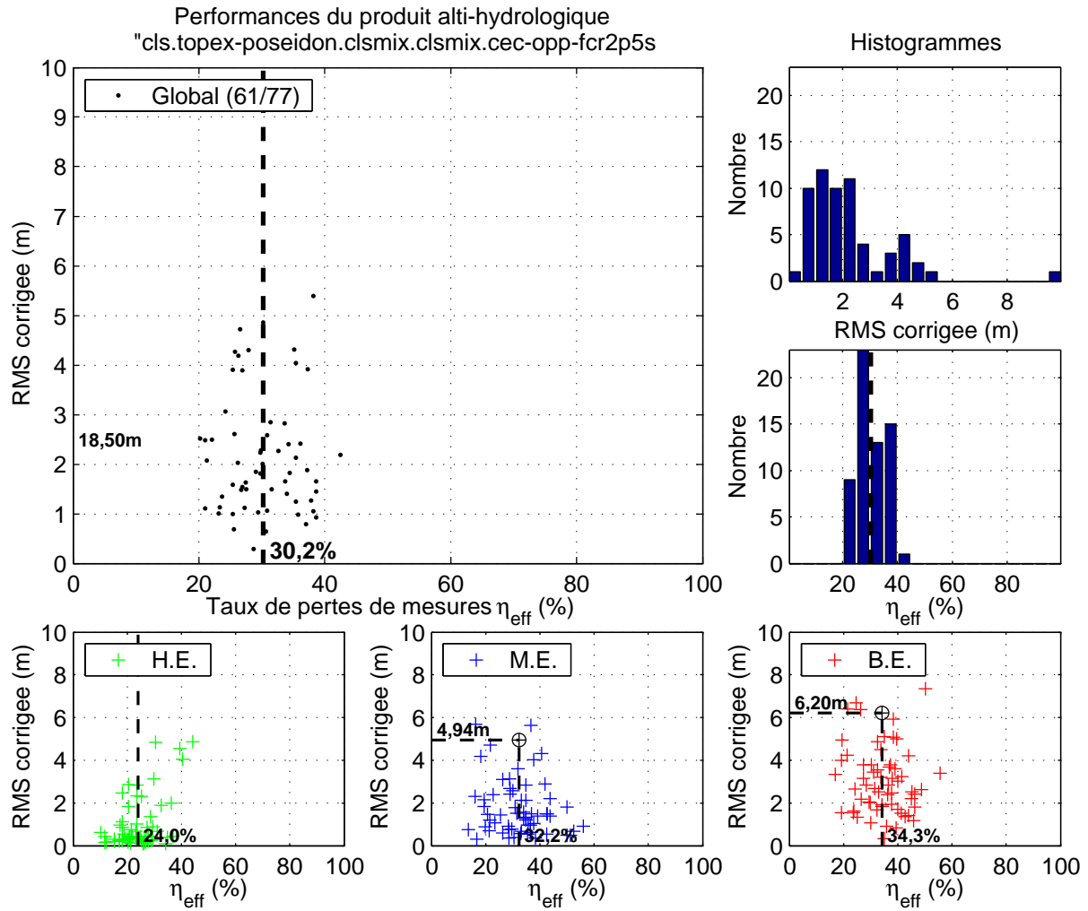
FIG. B.15: Figure de synthèse pour le produit alti-hydrologique « cls.topex-poseidon.clsmix.clsmix.cec-opp-fcr2p5s ».
