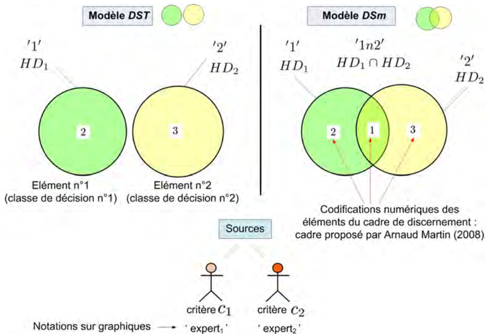
FIGURE 8.32 – Modèles DST et DSmT pour les cas de test du facteur d'affaiblissement d'importance
