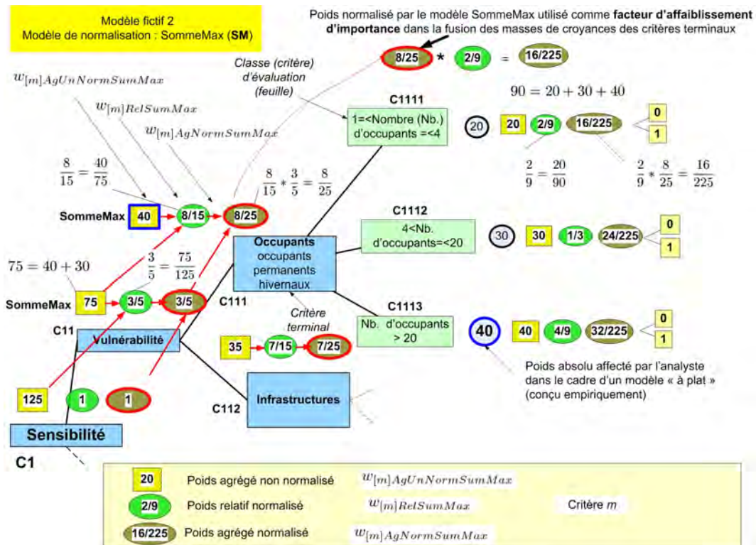
FIGURE 9.4 – Passage du poids agrégé normalisé ( SommeMax ) au facteur d'affaiblissement d'importance - critère C111
