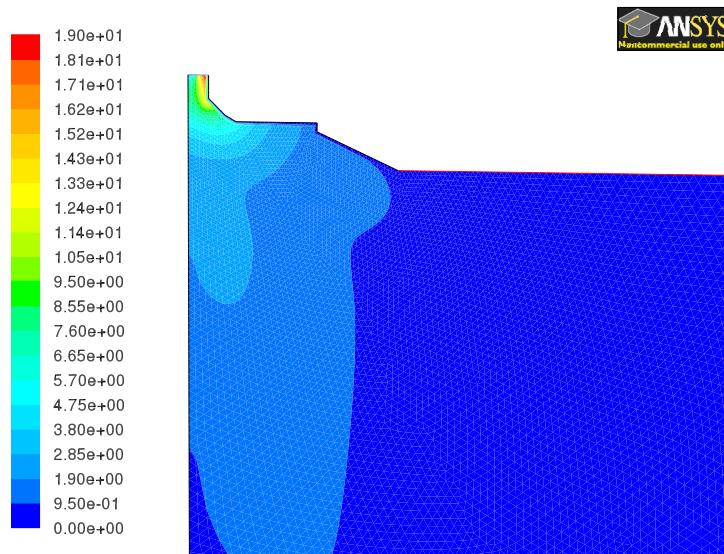
FIG. V.11 : Zoom de la figure (V.10)
