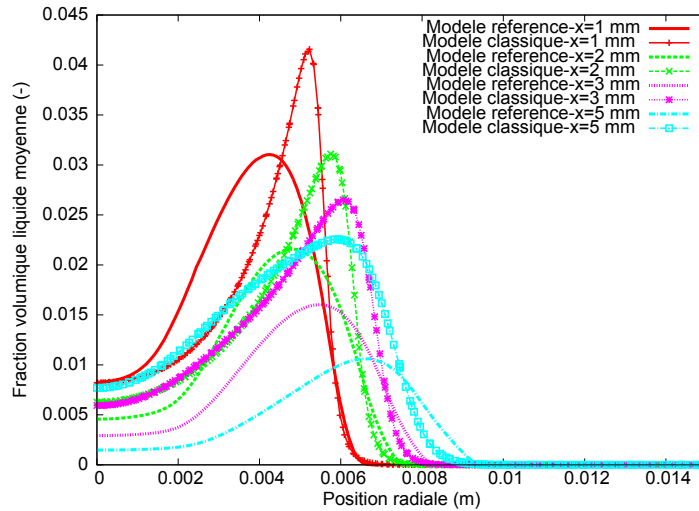
FIG. V.18 : Comparaison des profils transversaux de la fraction volumique liquide moyenne \bar{\gamma} (-) près de la sortie de buse : modèle de référence et modèle classique
