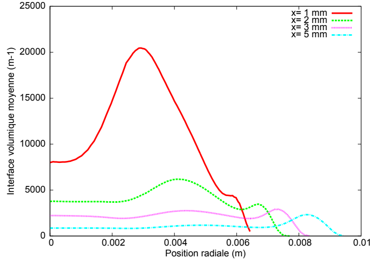
FIG. V.23 : Profils transversaux de l'aire interfaciale par unité de volume \bar{\Sigma} ( \text{m}^{-1} ) près de la sortie de buse
