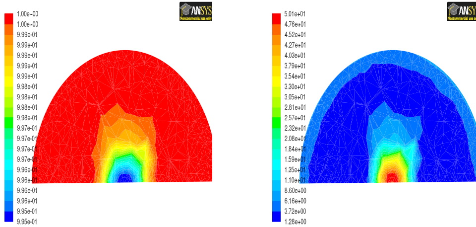
(a) Champ de la fraction massique \tilde{Y} à l'entrée du col dans un plan yz (b) Champ de l'énergie cinétique turbulente (m^2 \cdot s^{-2}) à l'entrée du col dans un plan yz
