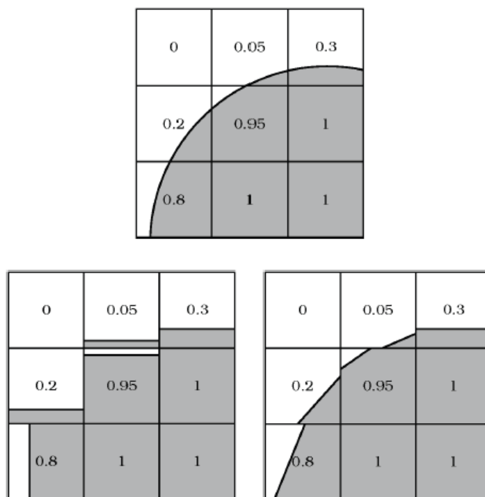
FIG. II.6 : Modèle VOF ; (en haut) Interface réelle et C associée ; (en bas à gauche) reconstruction par SLIC et C associée ; (en bas à droite) reconstruction par PLIC et C associée
