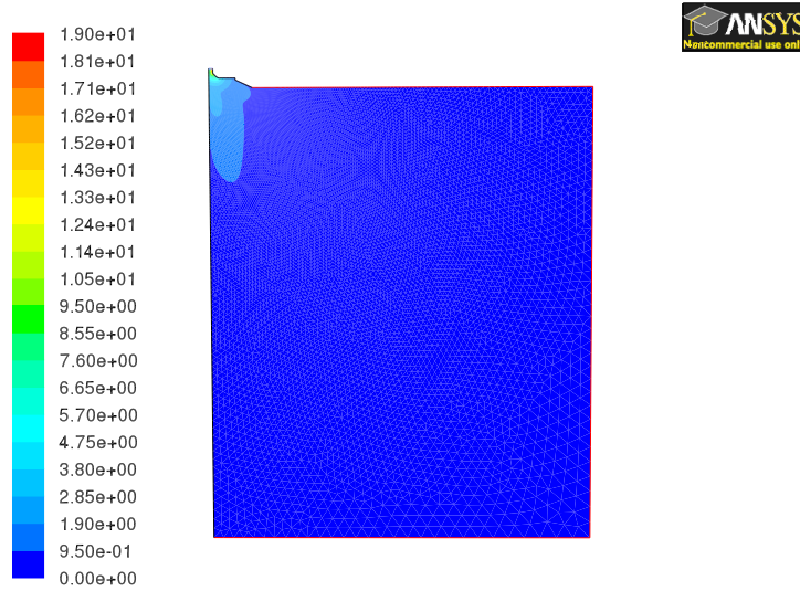
FIG. V.10 : Champ de la vitesse de swirl ( m \cdot s^{-1} )
