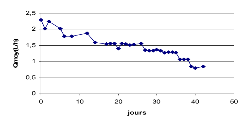
Figure IV-34 : Evolution du débit moyen de la ligne dans le temps (charge particulaire de l'eau = 0.2g/L^* ; [NaCl] = 0M )
