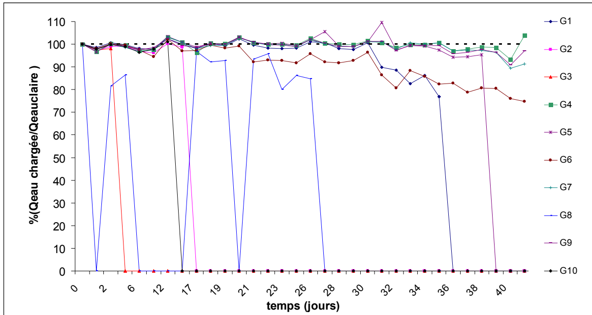
Figure IV-33 : Evolution du débit pour chaque goutteur par rapport au débit en eau claire durant toute la période des tests, pour [NaCl]= 0 M (8h/jour)
