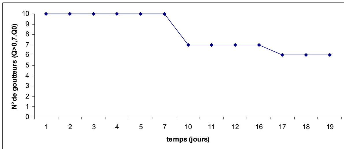
Figure IV-28 : Nombre de goutteurs dont le débit est supérieur à 70% du débit en eau claire ( Q_0 )
