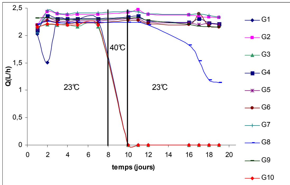
Figure IV-27 : Evolution temporelle du débit des goutteurs
