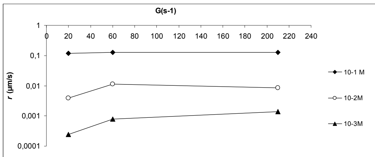
Figure IV-15: la cinétique d'agrégation exprimée en échelle logarithmique en fonction du cisaillement à 10^{-1} , 10^{-2} et 10^{-3} M de NaCl.
