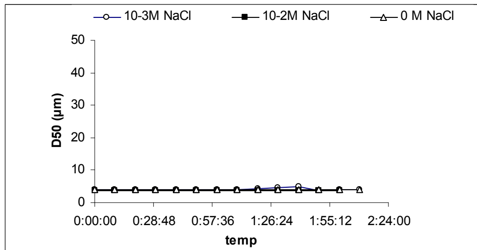
Figure IV-11 : Effet de la force ionique sur la taille des particules du mélange argilo-calcaire
