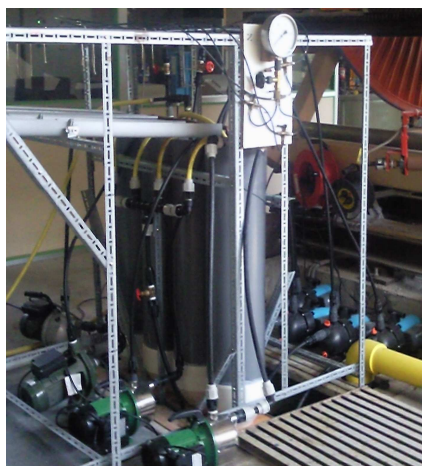
Figure IV-18 : Banc d'essai pour le mélange argilo-calcaire
