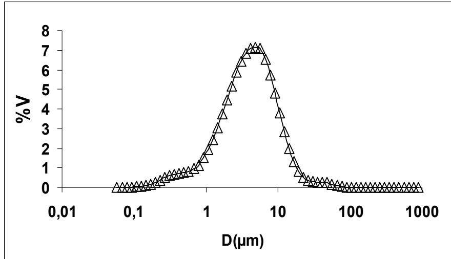
Figure IV-10 : Distribution volumique de la taille des particules du mélange argilo-calcaire sans adjonction de sel.
