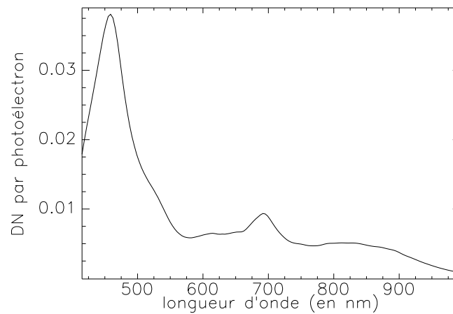
Figure 2.4: Sensibilité du capteur de la caméra Hypspec.
