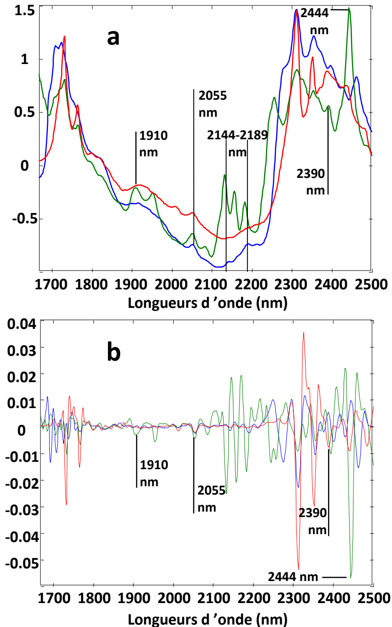
Figure 31 : Spectres de différents plastiques pris dans les échantillons.
