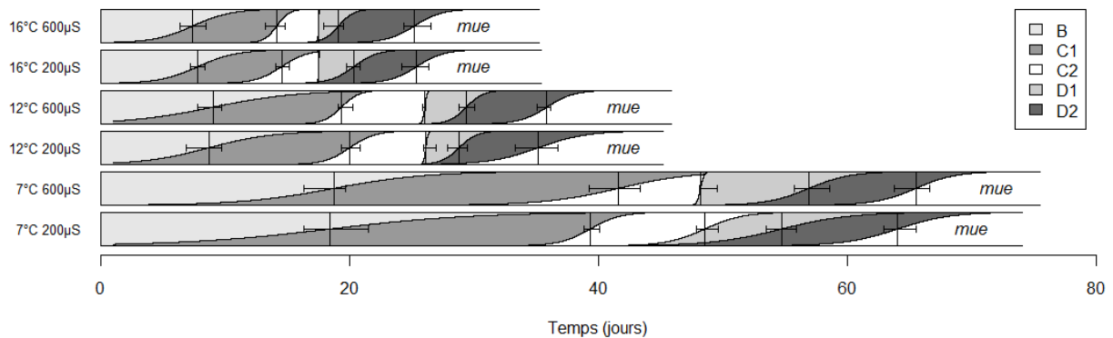
Figure III-2 : Durée (jours) des différents stades du cycle de mue de G. fossarum pour les trois températures : 7,0 (0,05) °C ; 12,1 (0,01) °C et 16,4 (0,3) °C et les deux conductivités : 200 (50) µS.cm -1 et 600 (50) µS.cm -1 du début du cycle jusqu'à la mue, durée estimée avec un modèle par stade, par température et par conductivité.
