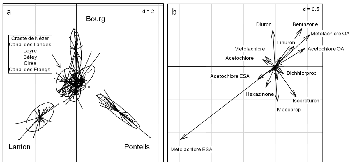
Figure 32. Analyse linéaire discriminante des profils de contamination des neuf tributaires du Bassin d'Arcachon. Projection des couples date-site groupés par site (a) et projection des contaminants les plus discriminants (b). Eigen values : 0,803 ; 0.605 (logiciel R).
