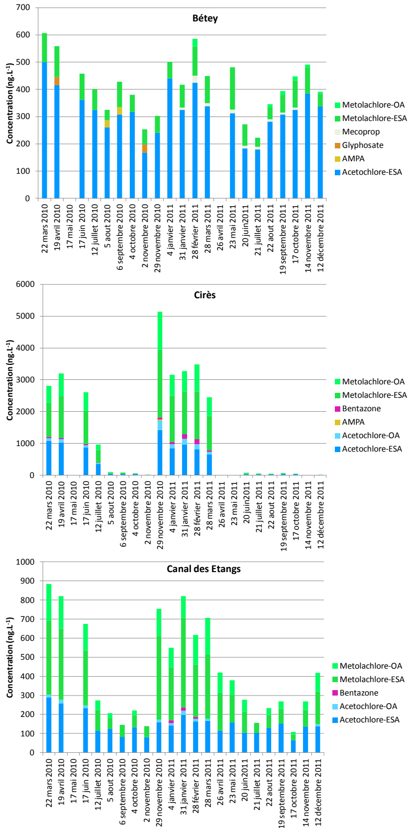
Figure 24. Suivi de la contamination en 21 herbicides acides dans les neuf principaux tributaires du Bassin d'Arcachon. Les astérisques marquent les dates auxquelles les données sont inexploitable, hormis pour le glyphosate et l'AMPA.
