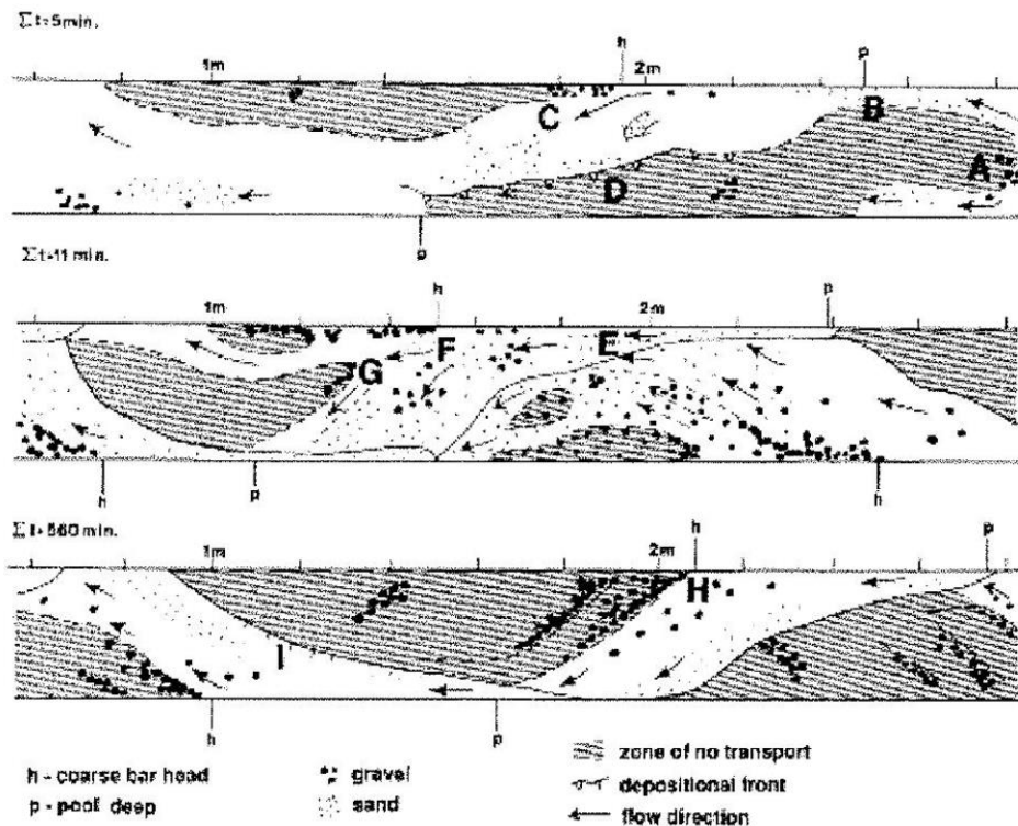
FIGURE 2.12 – Schéma de formation des bancs alternés d'après Lisle et al. 1991
