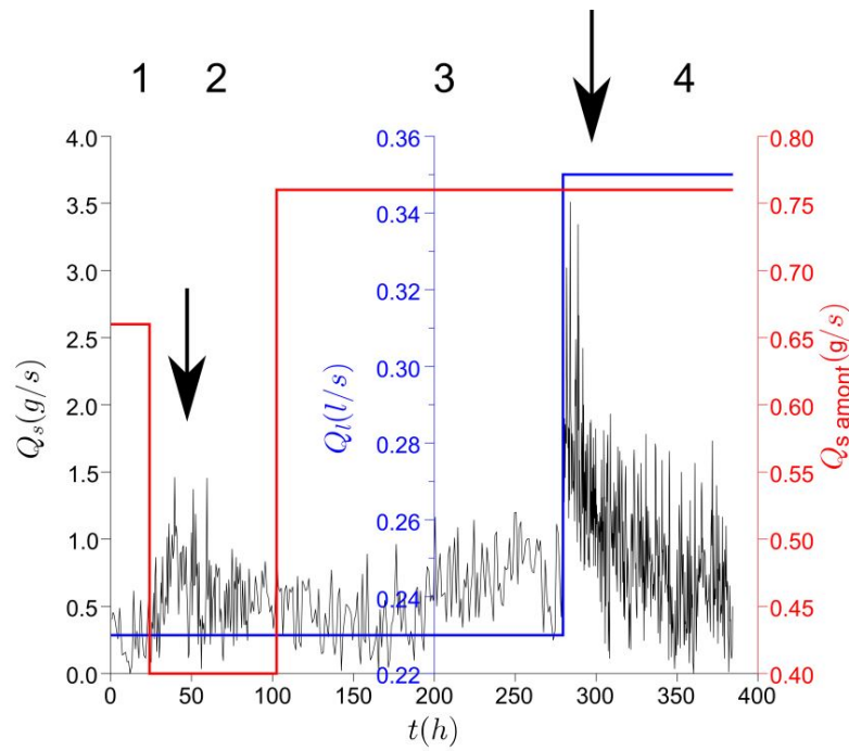
FIGURE 5.9 – Évolution du transport solide en sortie dans l’expérience en granulométrie uniforme - Les chiffres correspondent aux run, en rouge le transport solide en entrée ( Q_{s\text{ amont}} ), en bleu le débit liquide ( Q_l ), et en noir le débit solide en sortie ( Q_s )
