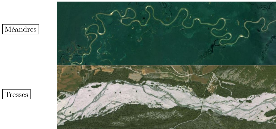
FIGURE 2.2 – Illustration de rivière à méandre (Amazonie, au Brésil) et de rivière en tresses (Nouvelle-Zélande) image Google Earth
