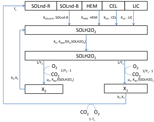
Figure 7 : Schéma du modèle de biodégradation aérobie de la matière organique
