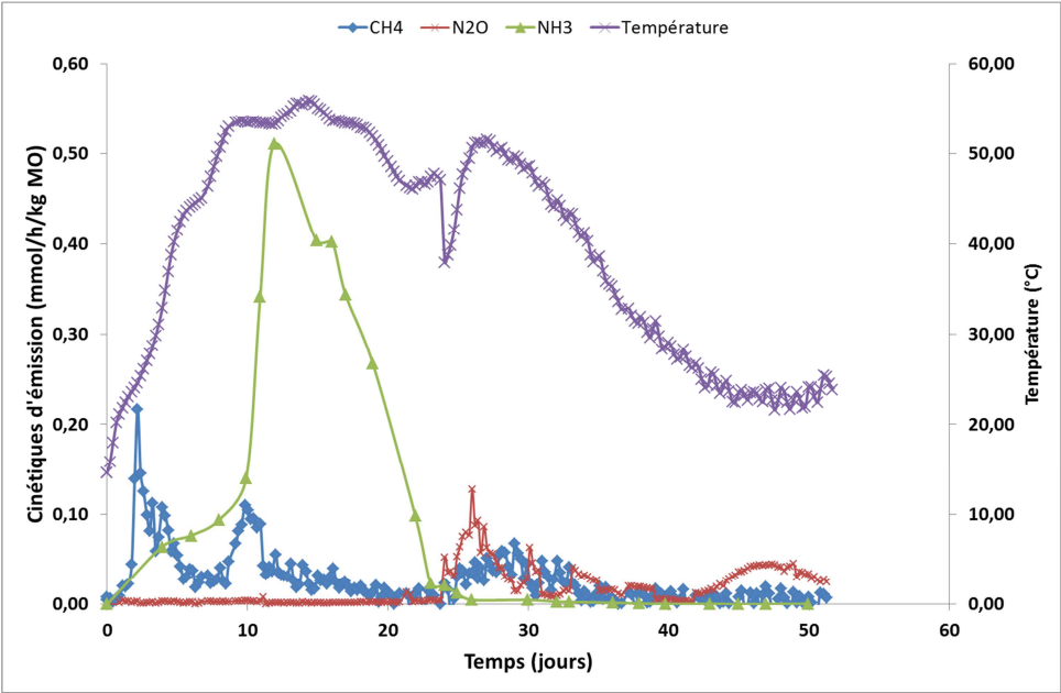
Graphique 18 : Dynamique des émissions gazeuses lors du compostage d'un digestat solide de fumier bovin
