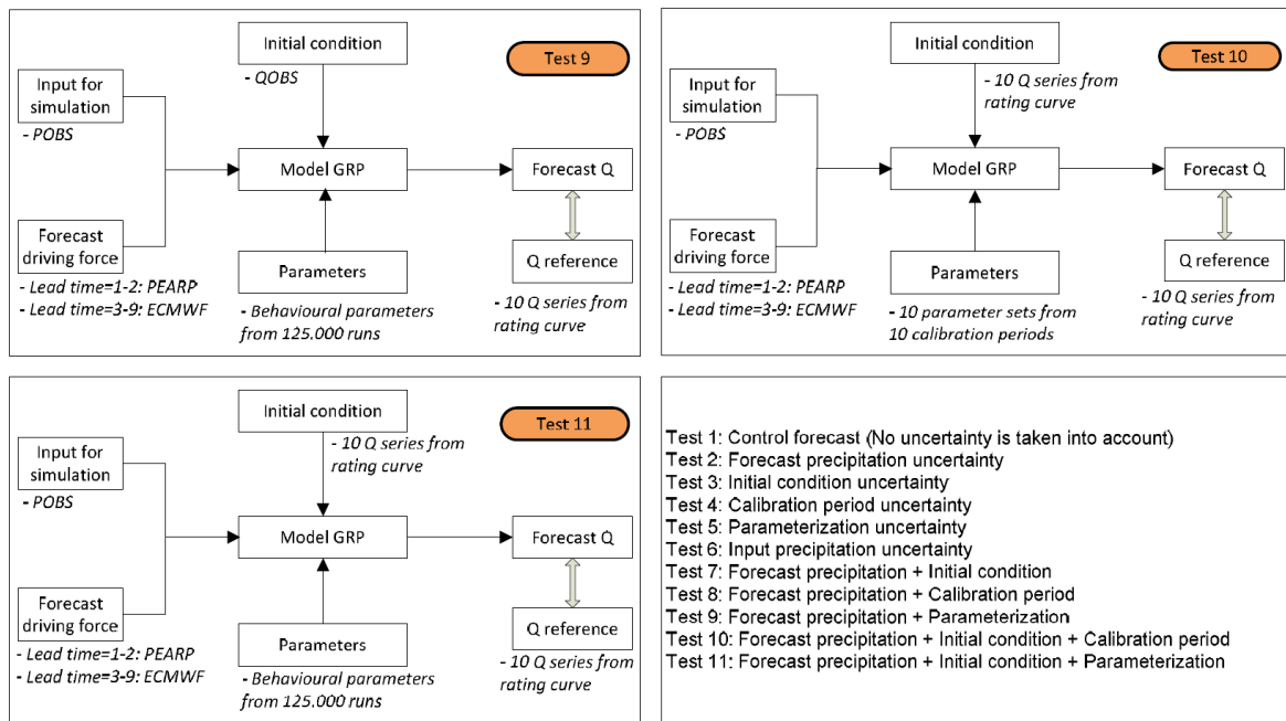
Figure 20 : Tests effectués pour la prise en compte explicite des différentes sources d'incertitude et leur propagation dans la chaîne de prévision de débit (dans : van Pham, 2011)
