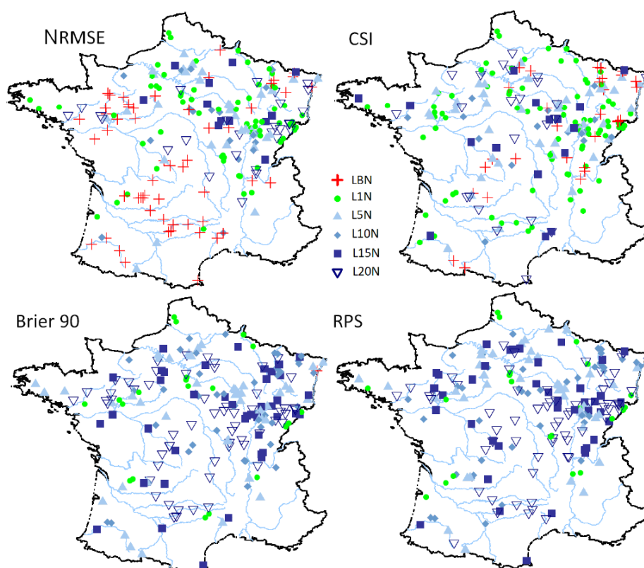
Figure 7 : Meilleurs donneurs des paramètres du modèle GR3P parmi les voisins (LBN, L1N,...L20N) du site non jaugé selon quatre critères de la qualité des prévisions hydrologiques d'ensemble (NRMSE, CSI, Brier 90 et RPS). Les paramètres sont transférés des sites voisins mais la mise à jour à l'instant de prévision est locale (dans : Randrianasolo, 2012)
