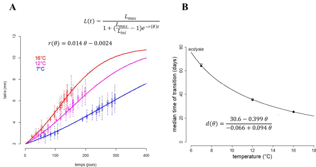
Figure 12. Quantification de l'influence de la température (A) sur la croissance et (B) la durée d'intermue (=inter-ponte) chez Gammarus fossarum . Trois températures ont été testées lors d'expérimentations au laboratoire. L longueur corporelle (mm), L_{max} taille maximale, L_{ini} taille initiale, r taux de croissance, t temps (jours), \theta température (°C), d durée d'intermue.
