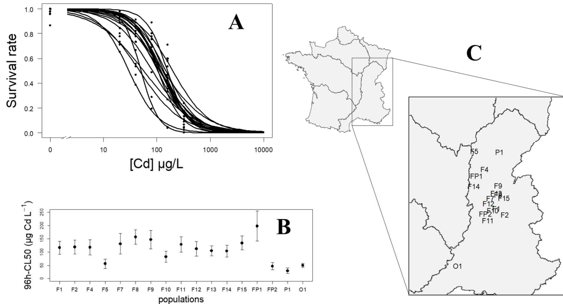
Figure 31. Comparaison entre populations de la sensibilité au cadmium. (A) courbes dose-réponse de mortalité à 96h d'exposition au laboratoire (une courbe par population). (B) CL50 (concentration létale pour 50% des organismes) après 4 jours d'exposition au Cd (moyenne \pm intervalle de confiance à 95%). (C) Les gammarès mâles testés ont été prélevés dans 17 populations non contaminées par le cadmium (présentées sur la Figure 29). F: G. fossarum ; P: G. pulex ; O: G. orinos .
