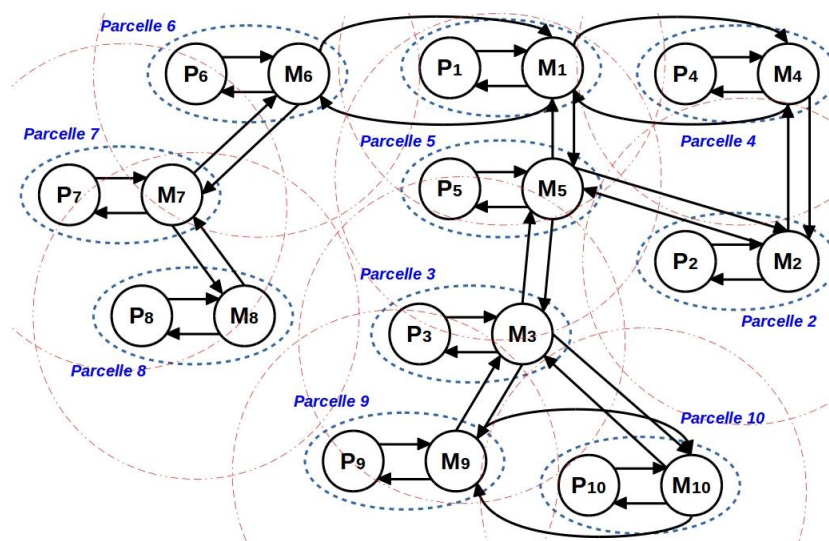
FIGURE 5.18 – Exemple de graphe issu d'une simulation de propagation de mildiou sur un parcellaire de taille 10. Dans cet exemple, la puissance du vent est faible, ce qui explique le faible rayon de contamination.
