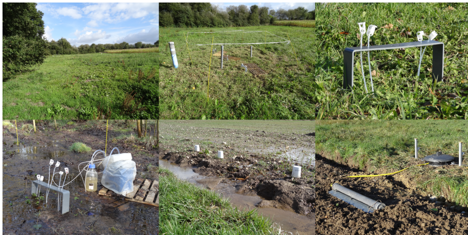
FIGURE 2.10 – Haut : bande enherbée de Guériniec ; piézomètres et pièges à eau en place ; piège à eau en place. Bas : prélèvement dans un piège à eau ; mini-piézomètre à l'interface entre la parcelle et la bande enherbée de Guériniec ; dispositif de collecte des eaux de ruissèlement.
