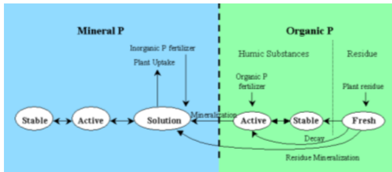
FIGURE 1.8 – Représentation des processus et des pools de phosphore dans le modèle SWAT (extrait du manuel de l'utilisateur)
