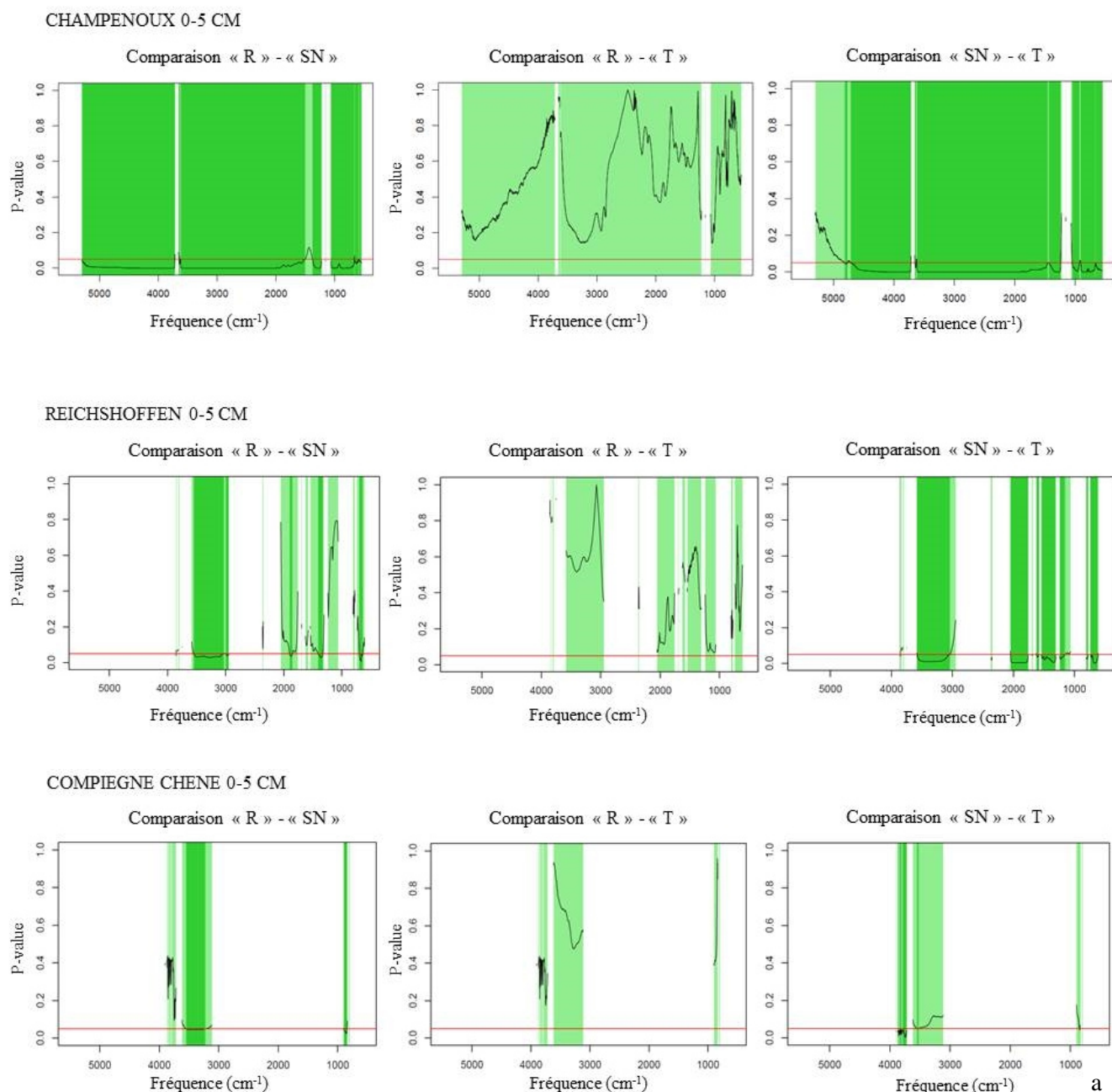
Figure 1a : Sortie du script R de comparaison de moyennes sur les données MIR pour l'horizon 0-5 cm des trois sites chênes. Lorsque l'effet est significatif, la courbe des p-values passe sous la barre rouge indiquant la valeur seuil de 0.05. Les gammes de fréquence d'onde pour lesquelles les effets « traitement » sont significatifs sont en vert vif. Les zones en blanc correspondent aux fréquences d'onde pour lesquelles il n'y a aucun effet significatif. Le vert pâle indique l'existence de différences significatives pour d'autres modalités que celles illustrées sur le graphe en question.
