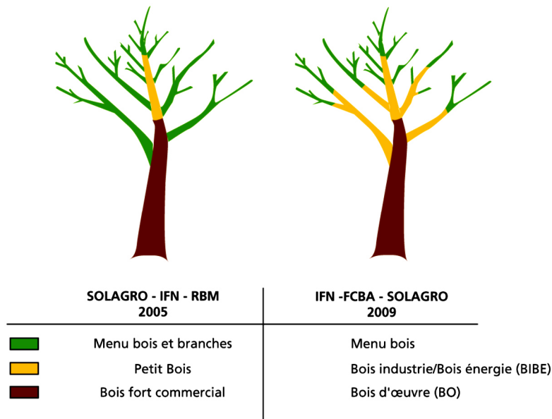
Figure 1.4 : Evolution de la définition des compartiments de biomasse par l'ADEME entre 2005 et 2009 (Landmann et al., 2009)
