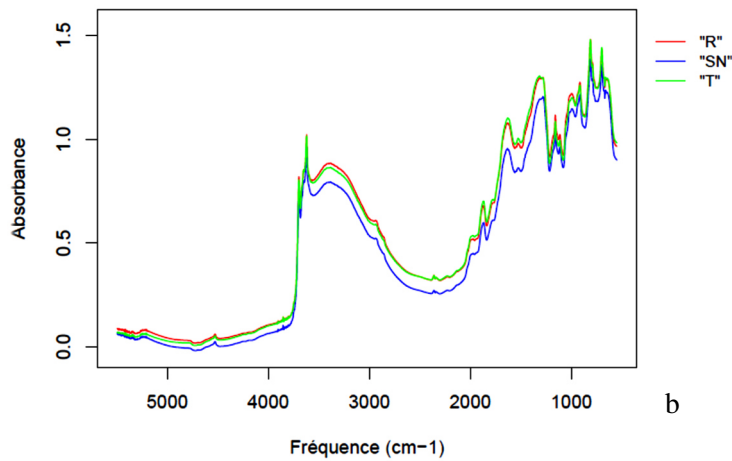
Figure 1b : Représentation des spectres MIR par traitement pour l'horizon 0-5cm du site de Champenoux
