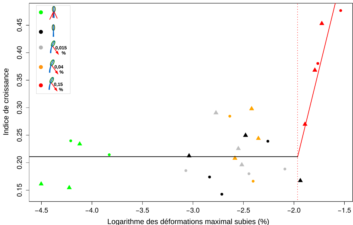
Figure 5.1: Prédications du modèle mécano-perceptif quantitatif (lignes) et observations ayant servis à son ajustement statistique.
