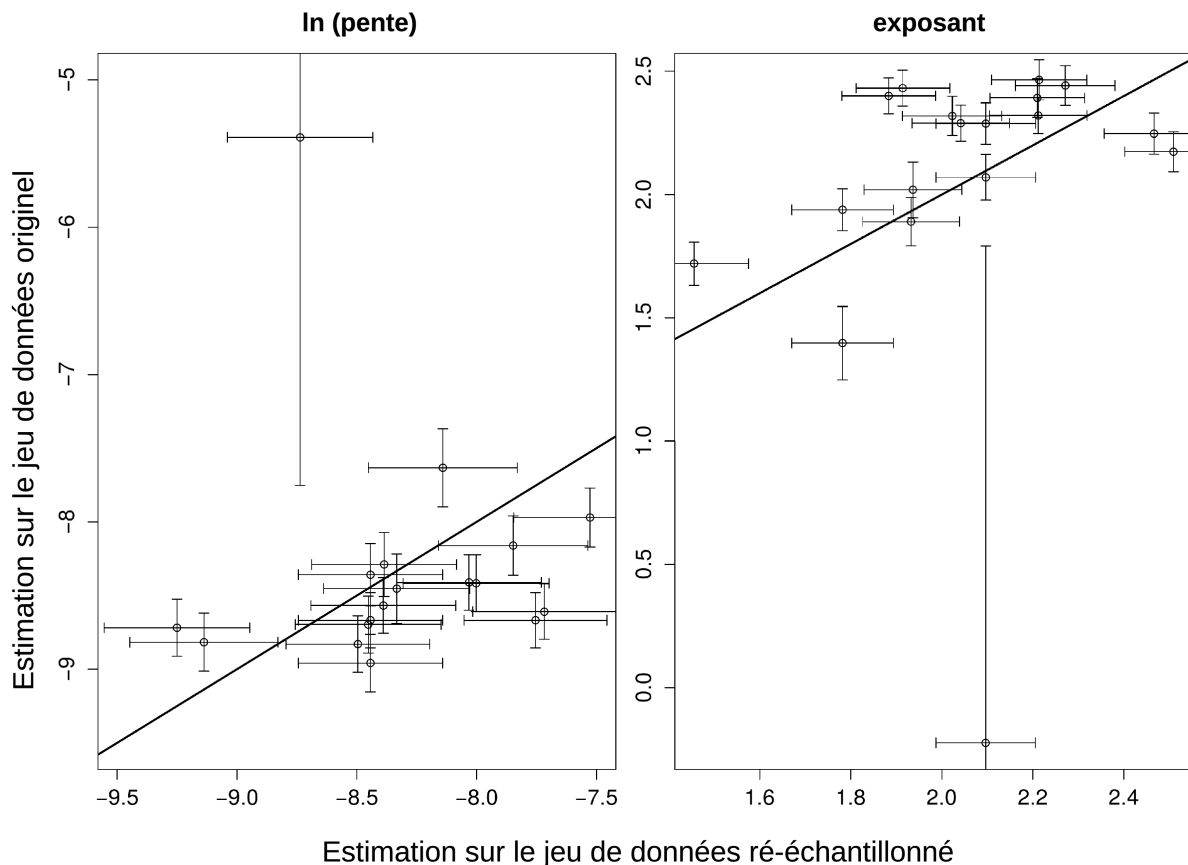
Figure 4.8: Comparaison de l'estimation des paramètres du logarithme de la pente (panneau de gauche) et de l'exposant (panneau de droite) du modèle ajusté sur les jeux de données originel et ré-échantillonné.
