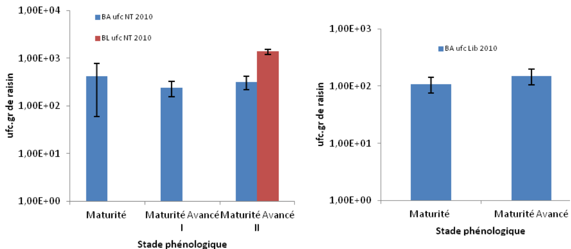
Figure 27: Evolution des populations BA et BL pour la parcelle d'expérimentale INRA-Grande Ferrade (à gauche), et pour les six parcelles de la région de Libournais (à droite). Les résultats présentés pour le Libournais sont la moyenne des valeurs obtenues pour les 6 parcelles. Les valeurs représentent la moyenne de 9 dénombrements maximum par échantillons.
