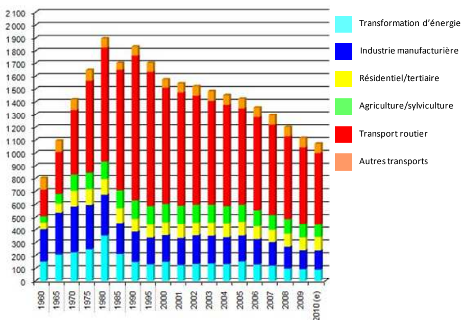
Figure 1.4. Emissions atmosphériques de NO x en France métropolitaine en kt avec une estimation préliminaire (e) pour 2010 (Serreau et al., 2011).
