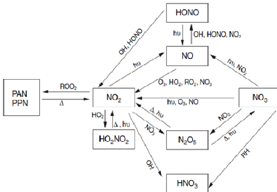
Figure 1.5. Interactions principales entre les différents composés oxydés de l'atmosphère ( \Delta : énergie thermique ; h\nu : photolyse ; \text{RH} : hydrocarbure ; PAN : peroxy acetyl nitrate ; PPN : peroxy propionyl nitrate) (Derwent & Hertel, 1998).
