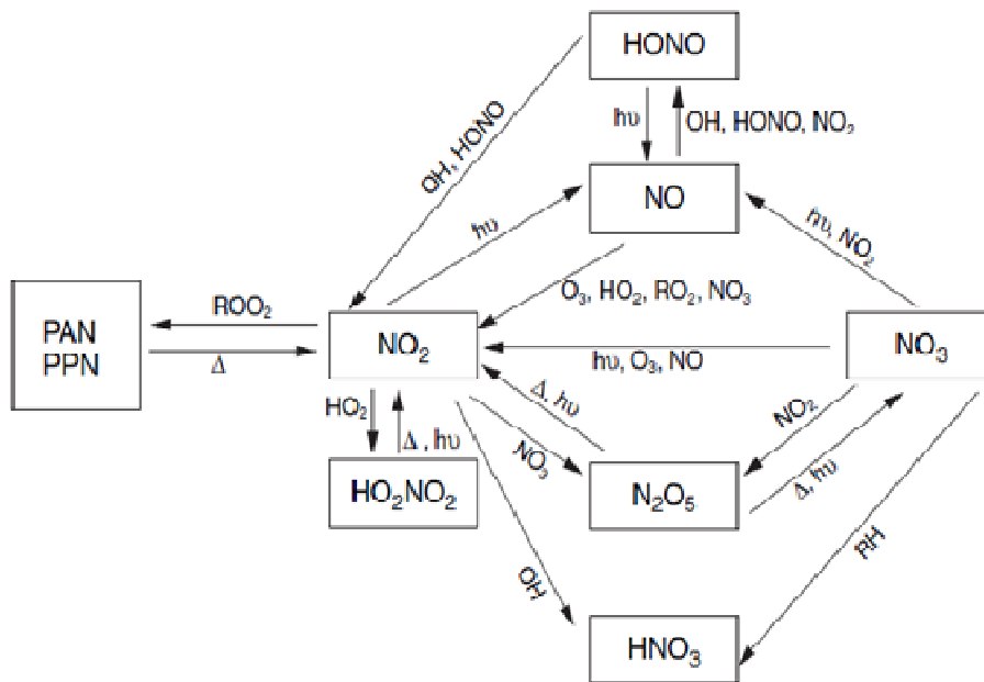
Figure 1.5. Interactions principales entre les différents composés oxydés de l'atmosphère ( \Delta : énergie thermique ; h\nu : photolyse ; RH : hydrocarbure ; PAN : peroxy acetyl nitrate ; PPN : peroxy propionyl nitrate) (Derwent & Hertel, 1998).
