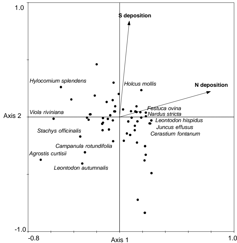
Figure 2.5. Diagramme d'ordination de la CCA (Canonical Correspondence Analyses) des axes 1 et 2 pour toutes les espèces avec les variables de dépôts de N et S utilisées comme variables environnementales et les variables de climat et de sol utilisées comme co-variables. Les espèces représentées sont présentes dans plus de 10% des sites (les espèces rares ont une faible contribution) et celles nommées sont associées positivement ou négativement aux dépôts de N, selon leur position dans le diagramme (Stevens et al. , 2010, article 2, annexe 2).
