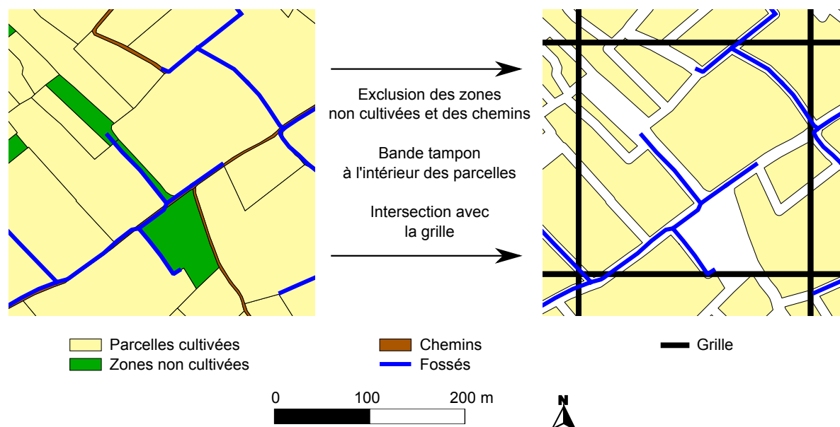
Figure 5.4 – Schéma d'agrégation utilisé pour la spatialisation du stream power index.
