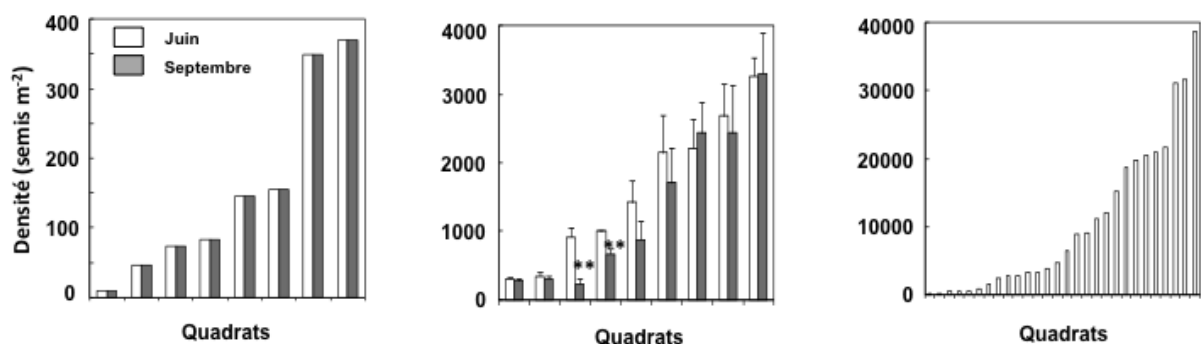
Fig. 6. Densité de semis par quadrat (m -2 ) à Paglia (a), Mareau-aux-Prés (b) et Arrault (c). Les histogrammes représentent les valeurs de densité mesurées à chaque date de collecte (blanc pour juin ; gris pour septembre) ; les valeurs de densité présentées à Mareau-aux-Prés correspondent à la moyenne \pm ES des trois quadrats adjacents (Chamaillard et al. en préparation)
