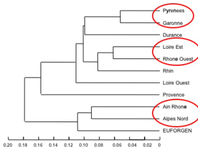
Fig. 14. Dendrogramme réalisé à partir des distances génétiques D de Nei (1978). Méthode UPGMA, Mardare (2004)
