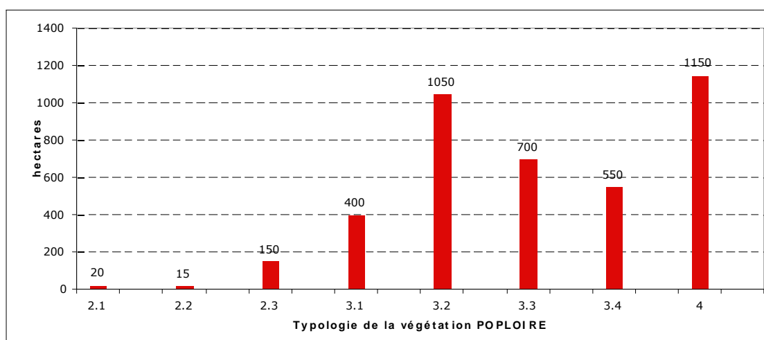
Fig. 9. Surfaces occupées par les différents écotopes le long de la Loire. Les écotopes sont définis dans la figure 8.
