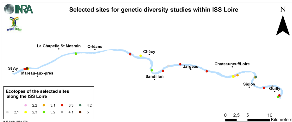
Fig. 12. Répartition spatiale et par écotope des 400 échantillons peuplier noir de l'ISS Loire, dont l'ADN est stocké de façon pérenne au 'Repository Centre' à Vienne en Autriche (dans le cadre du réseau d'excellence européen Evoltree).
