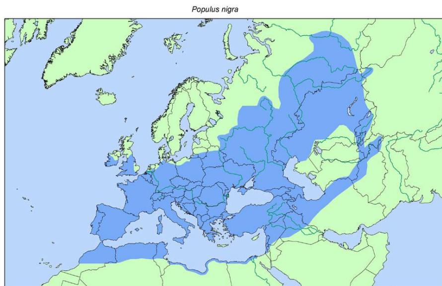
Fig. 1 : carte de répartition du peuplier noir, EUFORGEN 2009, www.euforgen.org
