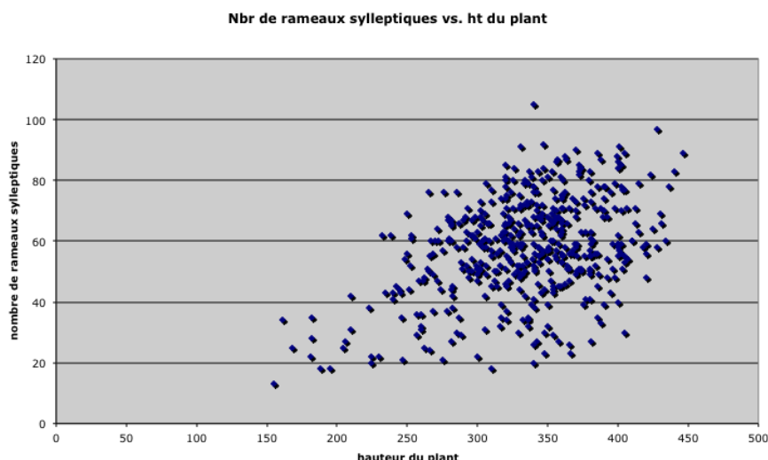
Fig. 18. Relation nombre de rameaux sylleptiques / hauteur de 90 géotypes de trois populations naturelles (dispositif 6 blocs randomisés mon arbre). Croissance en hauteur exceptionnelle de l'année sur le dispositif de Curcay-sur-Dive (données décembre 2010, Vienne)
