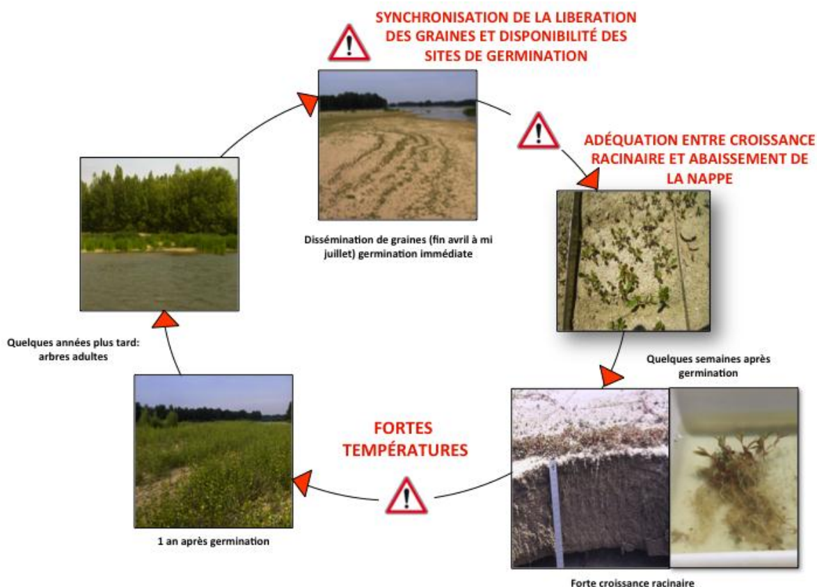
Fig. 5. Cycle de reproduction de Populus nigra . Les trois étapes critiques sont figurées en rouge et sont développées dans ce chapitre. Adapté de Chamailard (2011).
