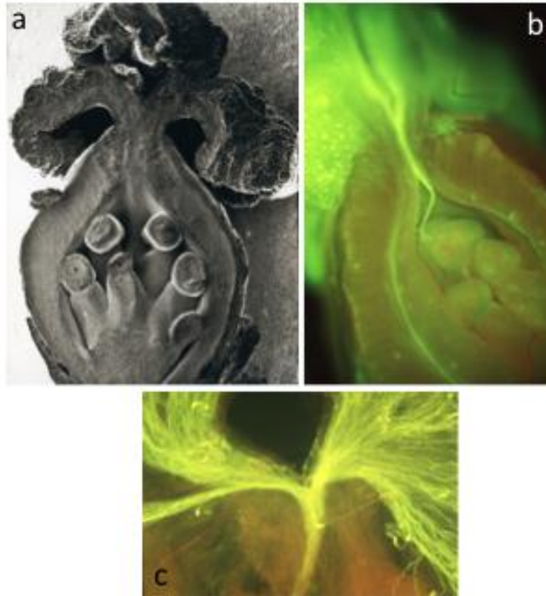
Fig. 2. Fleur de peuplier noir et interactions pollen-pistil.
