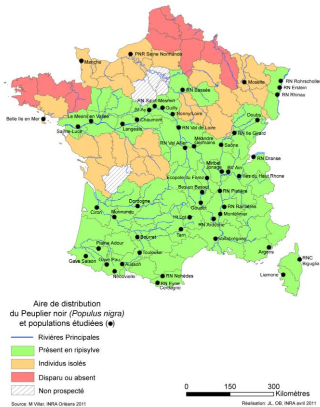
Fig. 22 Localisation des 50 populations naturelles, bases du programme de conservation des ressources génétiques du peuplier noir
