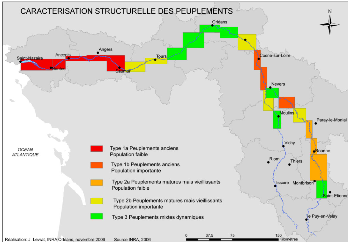
Fig. 10. Caractérisation structurelle des peuplements de la forêt alluviale : synthèse basée sur la surface et la typologie des peuplements mis en place dans le projet POPLOIRE
