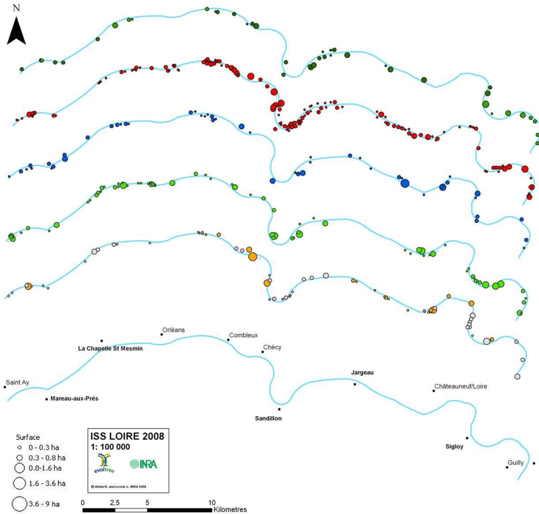
Fig 11. Répartition spatiale des écotopes sur les 53 km de l'ISS Loire. Les écotopes sont figurés comme suit : de haut en bas, 4.2 ; 3.3 ; 3.1 ; 3.2 et le dernier profil regroupe les écotopes 2.1/2.2/2.3
