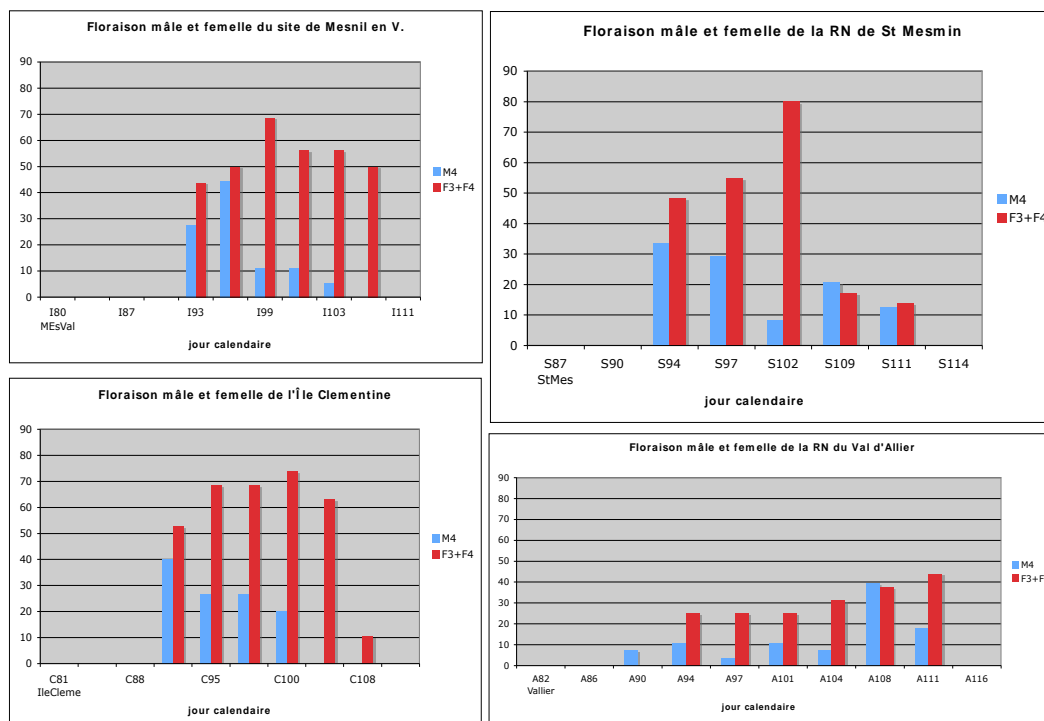
Fig. 3. Pourcentage de floraison de peupliers noirs femelles (rouge) et peupliers noirs mâles (bleu) de quatre des 13 populations de Loire. Les deux populations de gauche (populations proches de Nantes) présentent une floraison mâle plus précoce, les deux populations de droite (proche d'Orléans pour la RNN de St-Mesmin et de Moulins pour la RNN du Val d'Allier) présentent une meilleure synchronisation de floraison.
