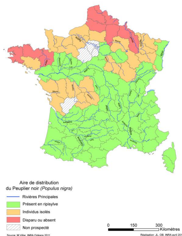
Fig. 7. Aire de répartition du peuplier noir en France
