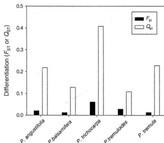
Fig. 15. Différenciation intrapopulation pour des marqueurs neutres ( F_{st} ) et son équivalent pour des caractères quantitatifs Q_{st} , calculé pour le débourrement végétatif chez cinq espèces de peuplier (tiré de Slavov GT et Zhelev P. 2010).
