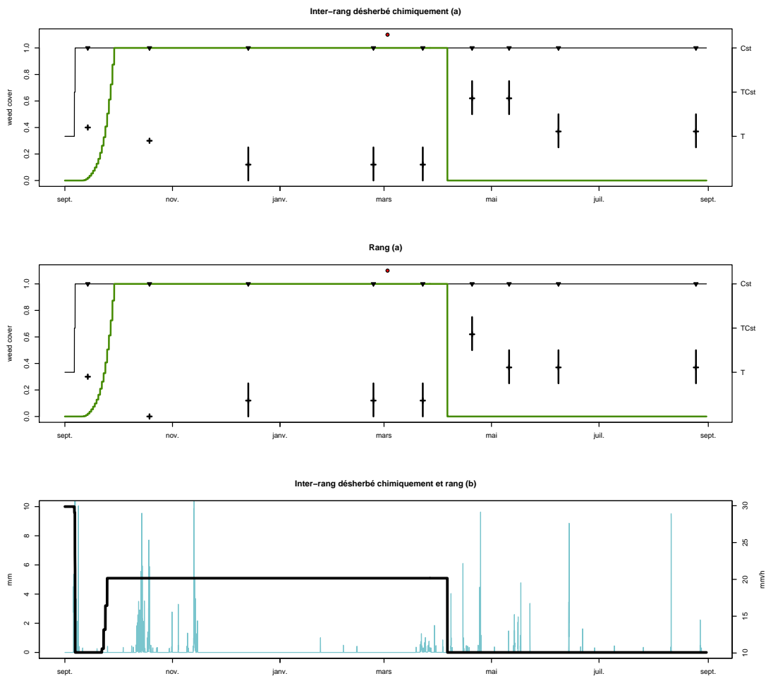
FIGURE 10.9 – Evolution de la couverture herbacée (courbe verte), des états de surface sur sols nus (courbe noire grasse) et de l'infiltrabilité (courbe noire grasse) modélisée pour les deux types de rangées de la parcelle NP06_03
