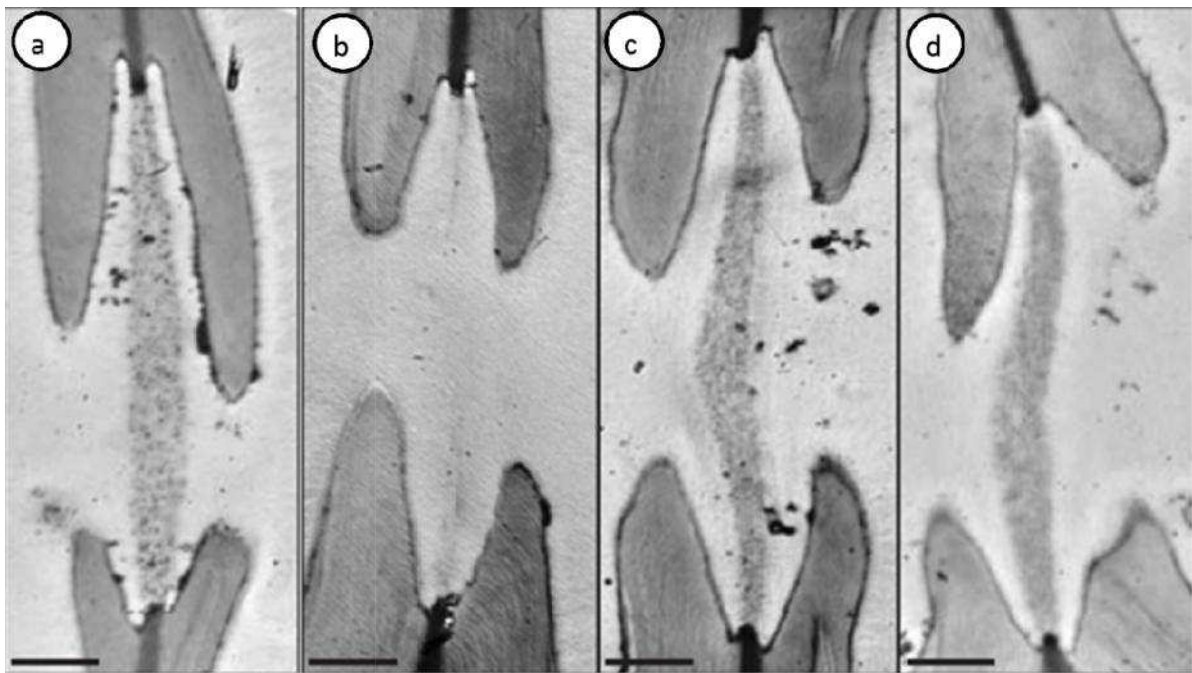
Figure 58 : Effets de traitements enzymatiques sur les punctuations de Fagus sylvatica . Des segments de tiges sont perfusés avec une solution témoin (a) ou avec une solution contenant une cellulase (b), une pecto-lyase (c) ou une hemicellulase (d) et incubés pendant 2 h à 37°C. Ensuite, des échantillons sont observés en MET. Les traitements de cellulases dégradent les membranes des punctuations alors qu'aucune différence n'est observée entre les échantillons témoins et les échantillons traités aux pecto-lyases et hémicellulases. Echelles : 1 \mu m. (Dusotoit-Coucaud et al., 2013).
